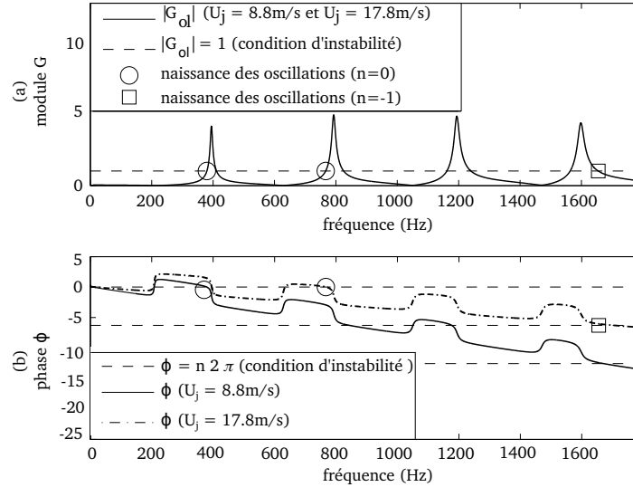
FIGURE 1.11: Module (a) et phase (b) du gain en boucle ouverte G_{ol} du modèle linéarisé autour de sa solution statique, pour un résonateur cylindrique de rayon 8\text{mm} , et pour deux valeurs de U_j , et donc de \tau et de P_m . Le système peut auto-osciller si le module est égal à 1 et si la phase est un multiple de 2\pi . Ces conditions sont indiquées par les lignes pointillées.
