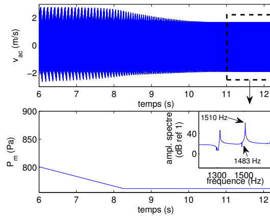
FIGURE 4.18: Signal de vitesse acoustique (en haut) obtenu lors de la simulation temporelle d'une rampe décroissante de P_m (en bas) se terminant par un plateau à P_m = 762 Pa , juste au-dessus du seuil de transition vers le premier registre prédit par le diagramme de bifurcation 4.15. Juste au-dessus de ce seuil, le spectre met en évidence une fréquence de modulation de 27 Hz . Les paramètres sont identiques à ceux utilisés pour le diagramme de bifurcation 4.15.
