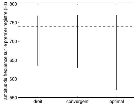
FIGURE 5.9: Représentation des plages de fréquence parcourues sur le registre principal, pour trois doigtés différents, et pour les trois canaux droit , convergent et optimal étudiés ici. Les lignes pointillées horizontales représentent la fréquence théorique de la note jouée.
