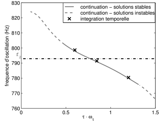
FIGURE 2.15: Fréquence d'oscillation en fonction du retard adimensionné \tilde{\tau} , pour une unique branche de solutions périodiques : comparaison des résultats obtenus par continuation numérique et par intégration temporelle. L'écart relatif maximum entre les résultats des deux méthodes est de 0.1% à \tilde{\tau} = 0.6 . La ligne noire en pointillés indique la valeur de la seconde fréquence de résonance ( f_2 = \frac{\omega_2}{2\pi} ).
