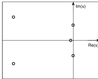
(d) Plan complexe : valeurs propres \kappa du système linéarisé autour de la solution statique en \lambda = 5 . Un couple de valeurs propres complexes conjuguées traverse l'axe imaginaire : point de Hopf.
