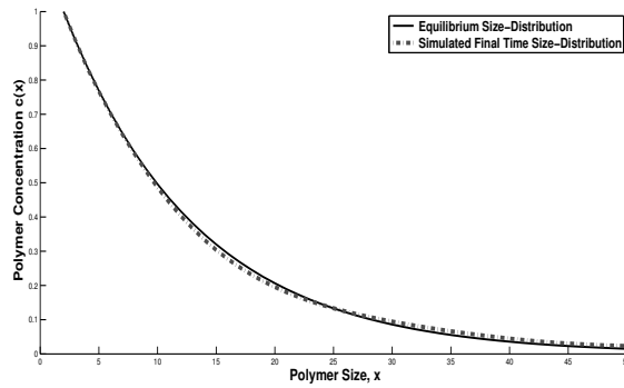
FIGURE 2.1 – Distribution des tailles à l'équilibre. La courbe en ligne continue noire représente la distribution des tailles théorique à l'équilibre, tandis que la courbe en tirets représente la distribution des tailles simulée pour des temps grands ( t = 10^6 \text{min} ). Les deux courbes coïncident, ce qui valide notre code numérique. Pour ces simulations on a pris k^{\text{dep}}/k^{\text{on}} = 2 \cdot 10^{-5} \mu M , et \rho = c_1(t = 0) = 22 \cdot 10^{-6} \mu M .
