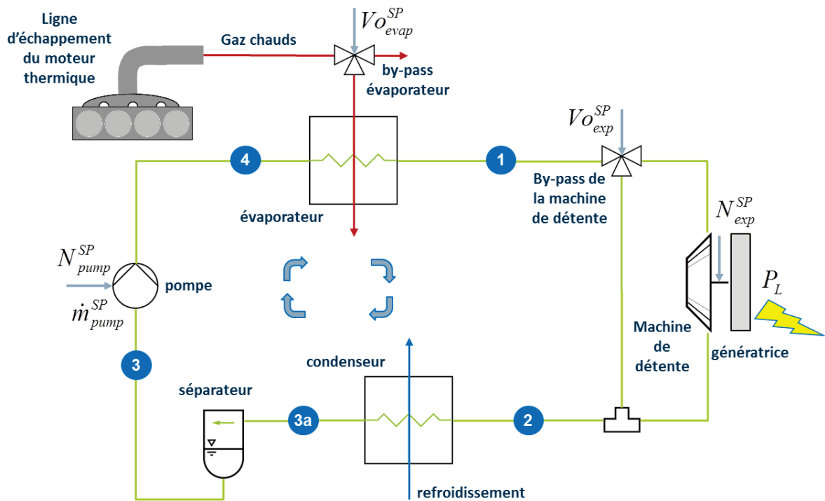
FIGURE 1.3 : Architecture matérielle d'un cycle de Rankine.
