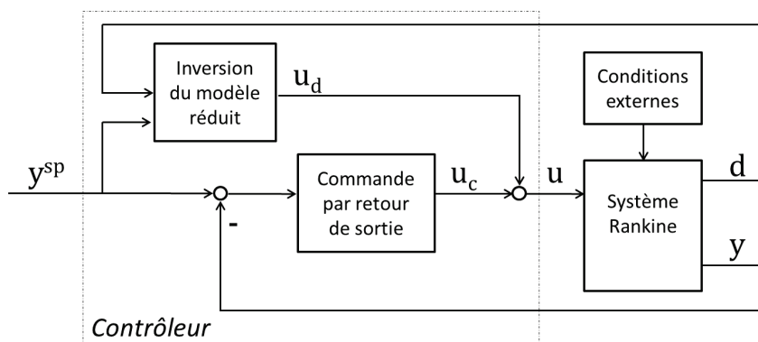
FIGURE 5.3 : Régulateur avec pré-compensation par inversion du modèle réduit.
