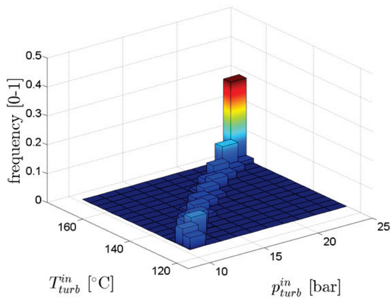
(b) Histogramme des points de fonctionnement turbine pour un grand volume de paroi évaporateur.
