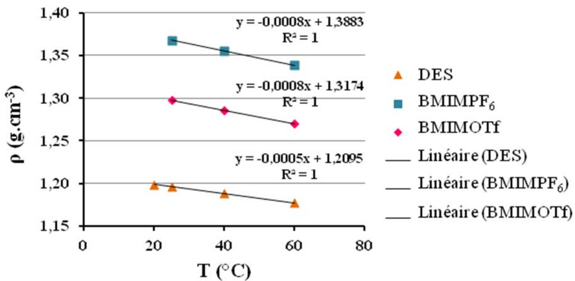
Figure 1. Droite de corrélation de la densité en fonction de la température ( \rho = f(T(^{\circ}\text{C})) ) pour les trois LIs (DES, BMIMPF 6 et BMIMOTf).
