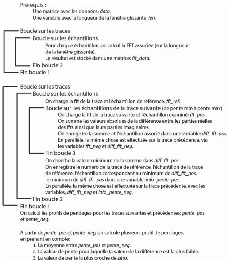
Figure 16 : Schéma explicatif de l'algorithme de calcul des pendages en domaine de Fourier.
