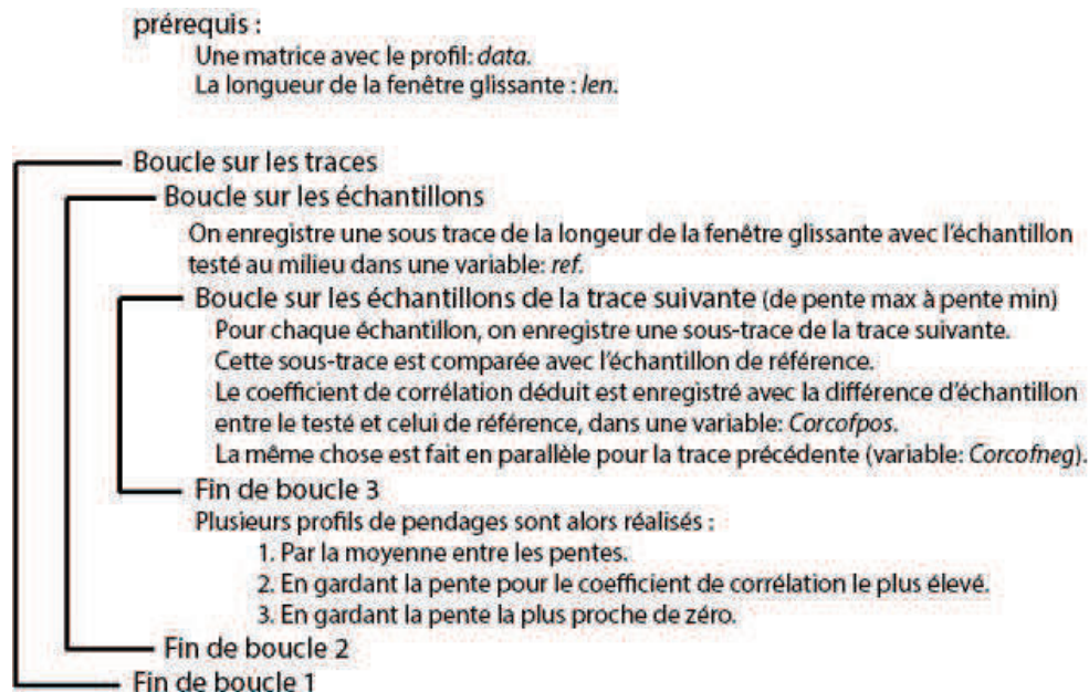
Figure 15 : Schéma présentant l'algorithme de calcul des pendages dans le domaine temporel.
