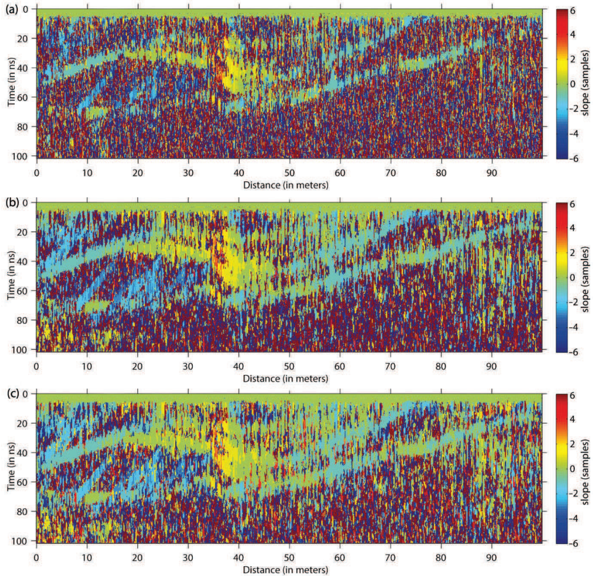
Figure 18 : Profils de pendages calculés en domaine temporel. L'algorithme calcule deux profils de pendages, l'un vers la trace suivante (pentes positives) et l'autre vers la trace précédente (pentes négatives). Les profils sont ensuite mélangés en prenant (a) la moyenne entre les pentes positives et les pentes négatives ; (b) la pente avec le coefficient de corrélation associé le plus élevé et (c) la pente la plus faible entre la pente positive et la pente négative.
