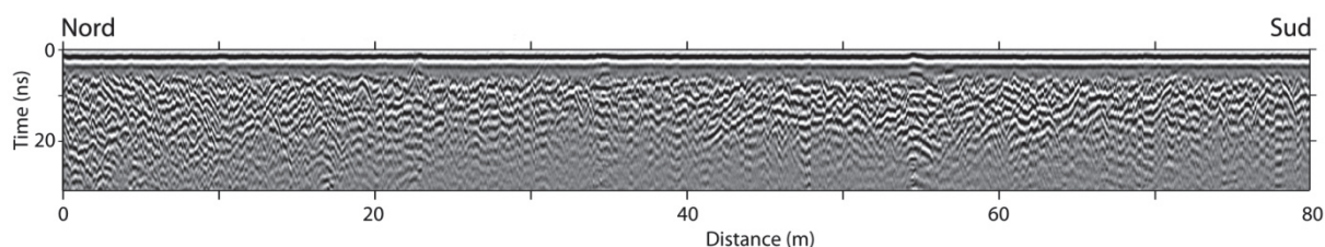
Figure 20 : Exemple d'un profil réalisé avec l'antenne de 500 MHz sur la zone ZO. Seuls les 80 premiers mètres sont affichés. Un unique faciès, présentant des réflexions à continuité modérée à discontinue, et affichant une configuration chaotique, localement subparallèle est observé.
