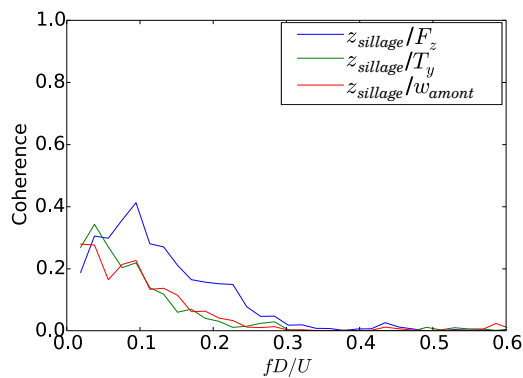
FIGURE 5.19 – Cohérences entre la position verticale du sillage, les efforts et la vitesse verticale en amont du disque pour le cas avec un disque unique
