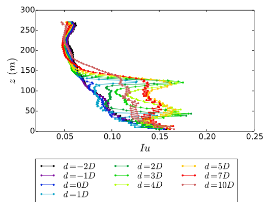
FIGURE 6.9 – Profils verticaux d'intensité turbulente longitudinale à différentes positions sur l'axe x
