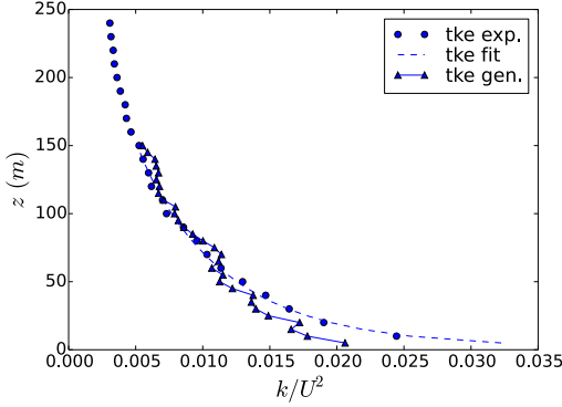
FIGURE 4.5 – Profil d'énergie cinétique turbulente k du champ synthétique
