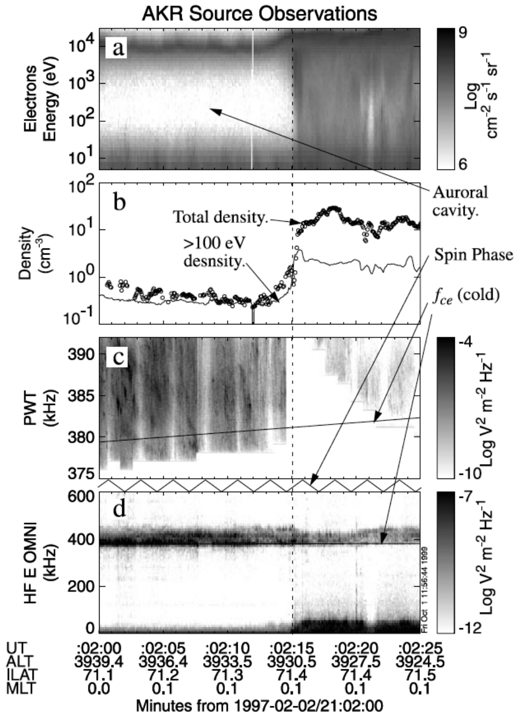
FIGURE 8.1 – Mesures par le satellite FAST (Fast Auroral Snapshot) de l'énergie et de la densité des électrons dans une région source de l'AKR. L'axe horizontal représente \sim 150 \text{ km} ( 25 \text{ s} d'observation) d'une zone aurorale située à 4000 \text{ km} d'altitude et à 70^\circ de latitude. La ligne verticale pointillée correspond à la sortie du satellite hors de la cavité aurorale. a) Flux d'énergie des électrons en fonction de l'énergie et du temps. Il n'y a aucun flux d'électron mesurable entre \sim 100 \text{ eV} et \sim 1 \text{ keV} dans la cavité aurorale. Les flux inférieurs à 100 \text{ eV} correspondent aux photoélectrons produits par le satellite. b) Densité totale d'électrons (cercles) et densité des électrons chauds ( > 100 \text{ eV} , trait plein). Une population chaude et une population froide sont présentes en dehors de la cavité, tandis que la cavité n'est peuplée que d'électrons chauds. c) Densité spectrale de puissance du champ électrique mesuré par l'instrument Plasma Wave Tracker. La ligne horizontale représente la fréquence cyclotron en plasma froid ( 400 \text{ kHz} ). Les émissions s'étendent en dessous de f_{ce} (froid). d) Densité spectrale de puissance du champ électrique entre 0 et 600 \text{ kHz} . D'après [Ergun 2000].
