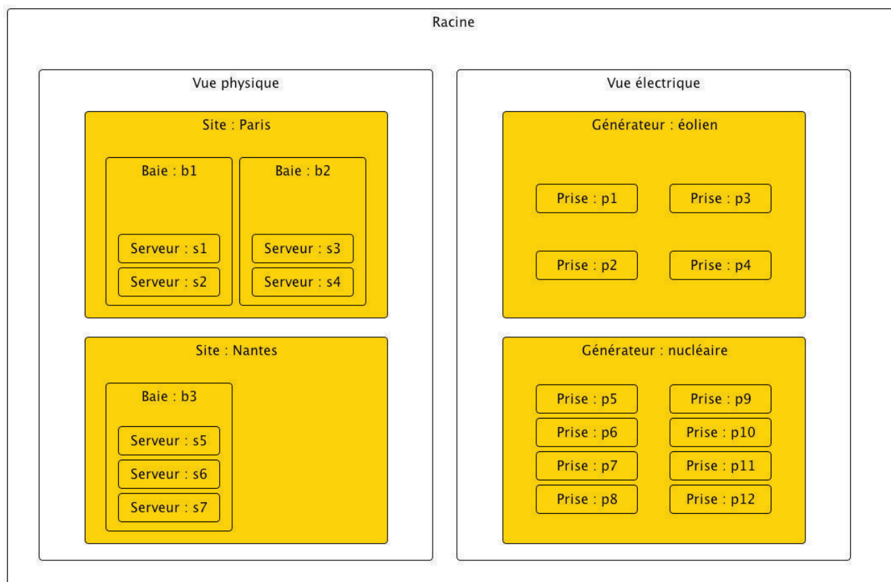
FIGURE 4.1 – Utilisation des types comme conteneurs d'éléments
