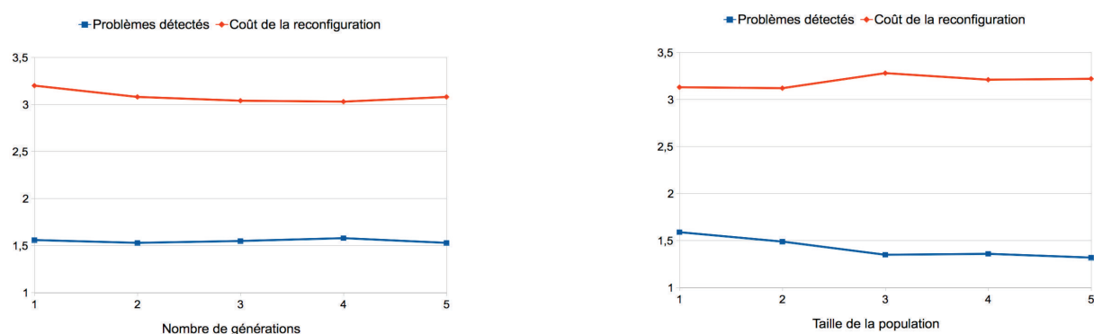
FIGURE 6.1 – Influence du nombre de générations et de la taille de la population
