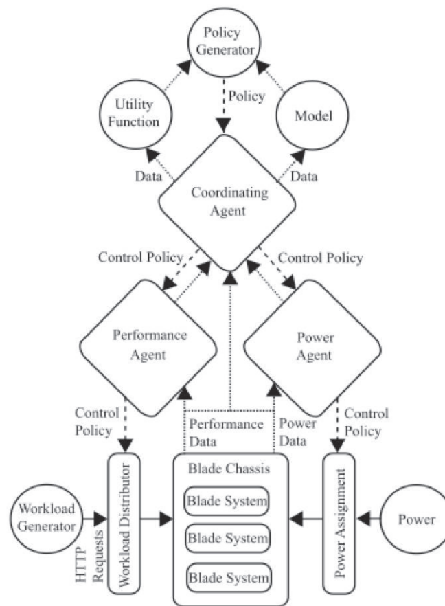
FIGURE 3.5 – Architecture multi-agents pour la mise en place d'une politique d'économie d'énergie
