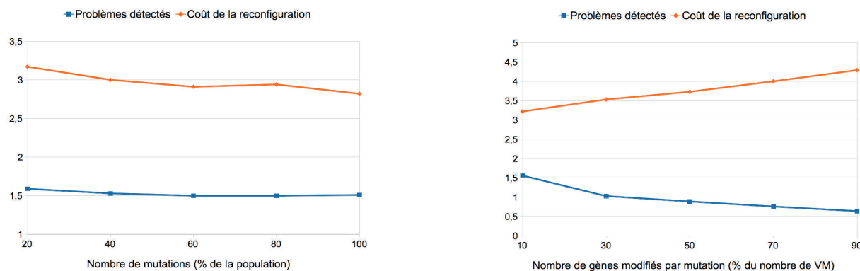
FIGURE 6.2 – Influence du nombre de mutations et du nombre de gènes modifiés par mutation
