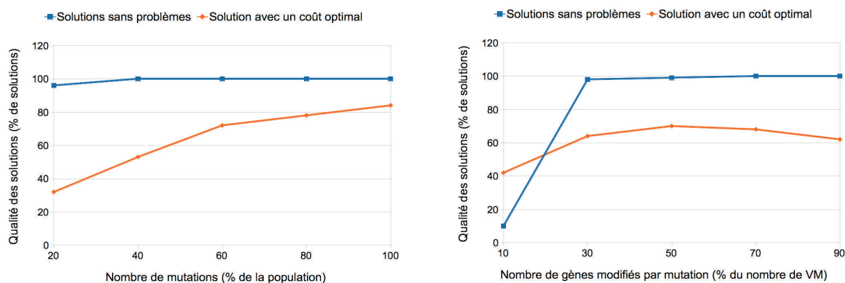
FIGURE 6.5 – Affinage du nombre de mutations et du nombre de gènes modifiés par mutation
