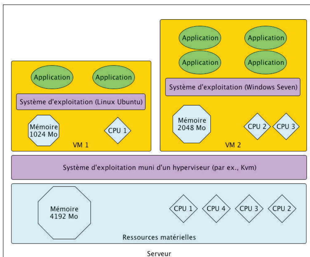
FIGURE 2.1 – Un serveur hébergeant des machines virtuelles
