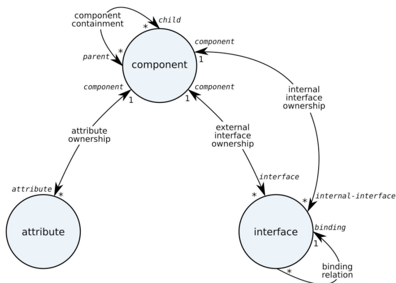
FIGURE 3.9 – Les axes de navigation utilisés par FPath
