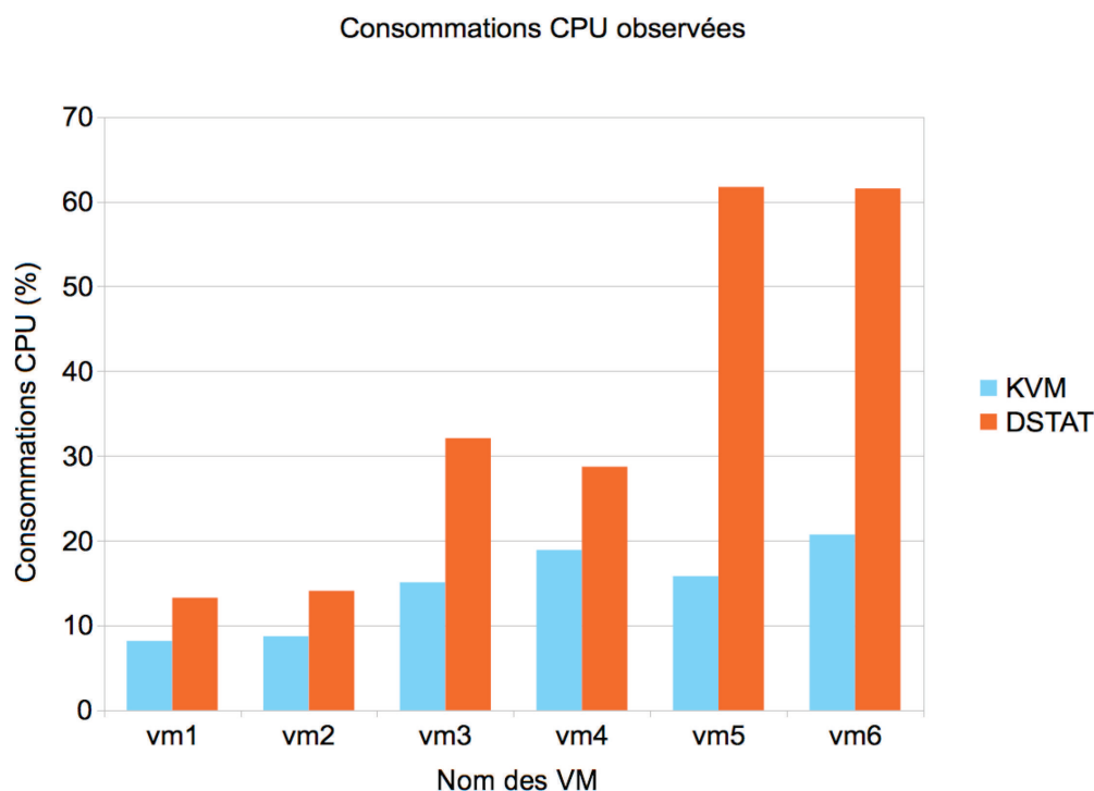
FIGURE 5.5 – Consommations CPU observées à partir de l’hyperviseur KVM et à l’aide de l’outil dstat
