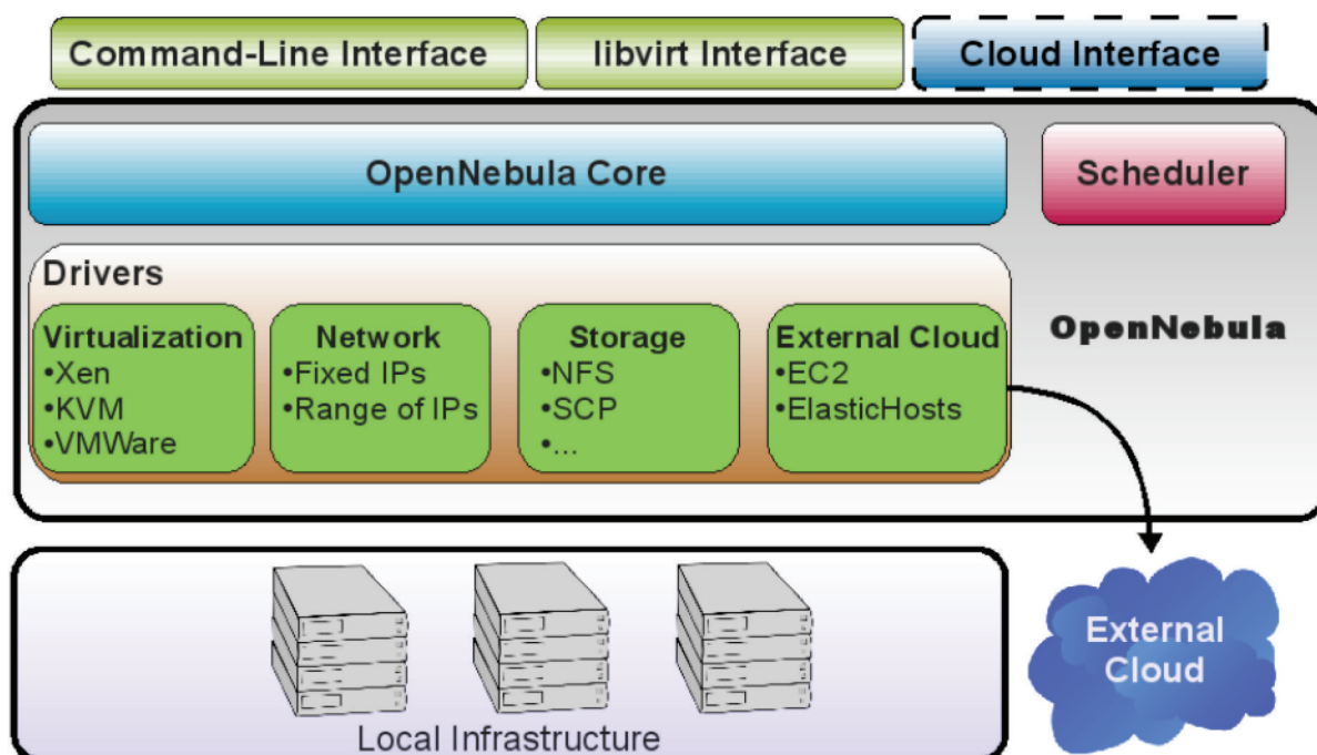
FIGURE 3.3 – Les différents modules d'OpenNebula
