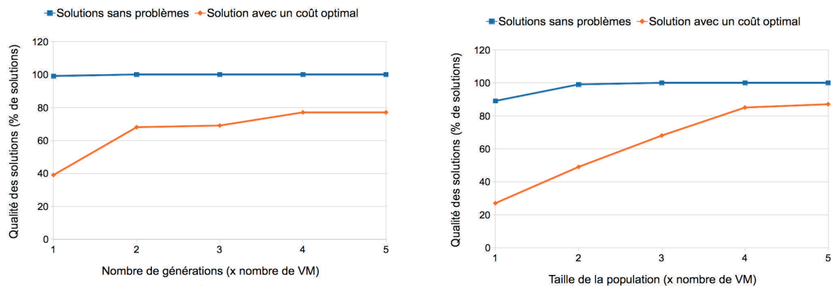
FIGURE 6.4 – Affinage du nombre de générations et de la taille de la population
