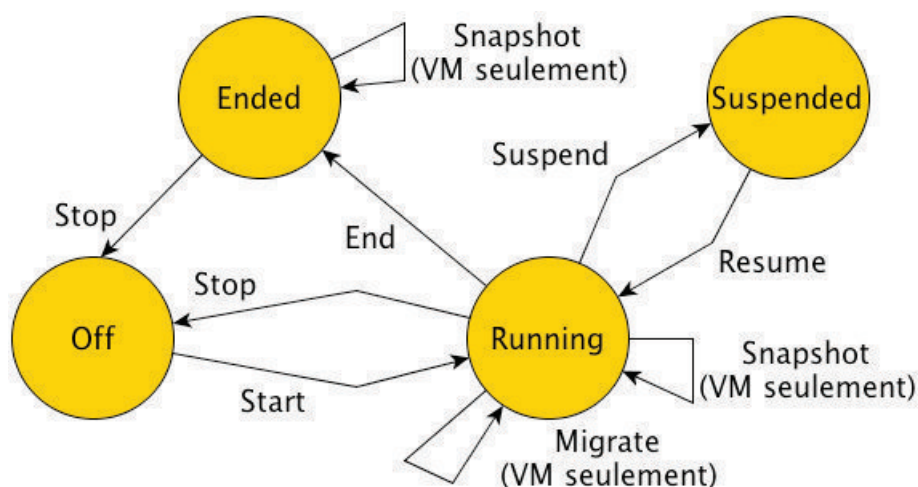
FIGURE 3.1 – Le cycle de vie d'un serveur ou d'une machine virtuelle. Les flèches montrent les reconfigurations modifiant l'état de la VM ou du serveur. L'état « ended » permet de spécifier que le serveur ou la VM doit être arrêté. Pour un serveur, cet état permet de programmer une maintenance. Le serveur doit être vidé de ses VM et ne peut pas accueillir de VM supplémentaires. Pour une VM, l'état « ended » permet à l'administrateur d'effectuer une sauvegarde avant l'extinction de la VM.
