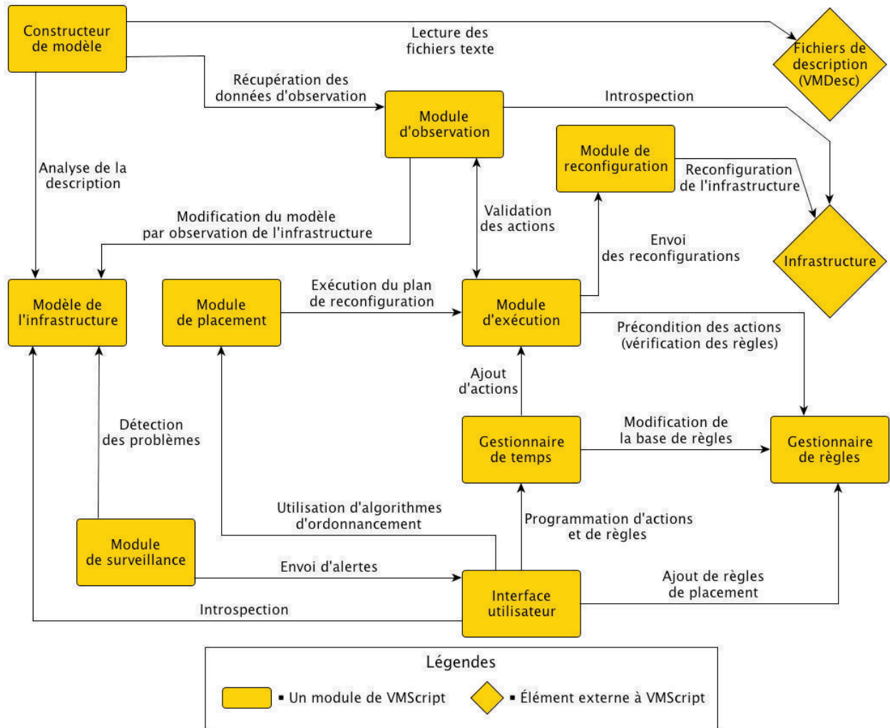
FIGURE 5.4 – Les différents modules de l'outil d'administration
