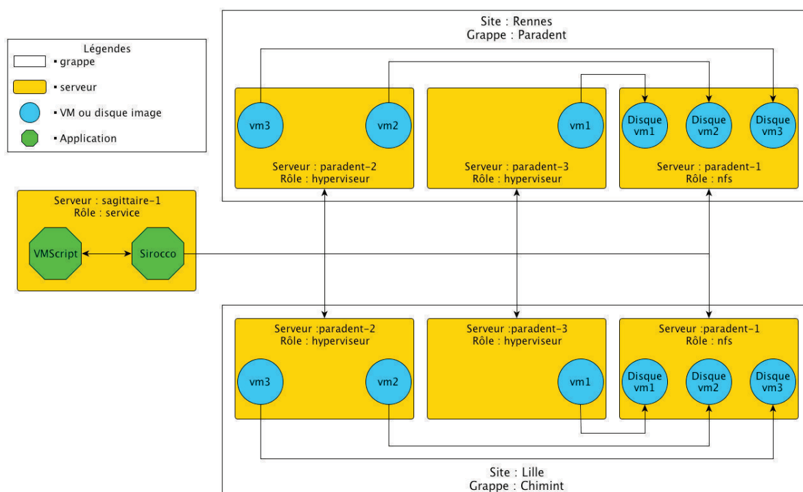
FIGURE 6.7 – Description de l'infrastructure déployée sur Grid5000
