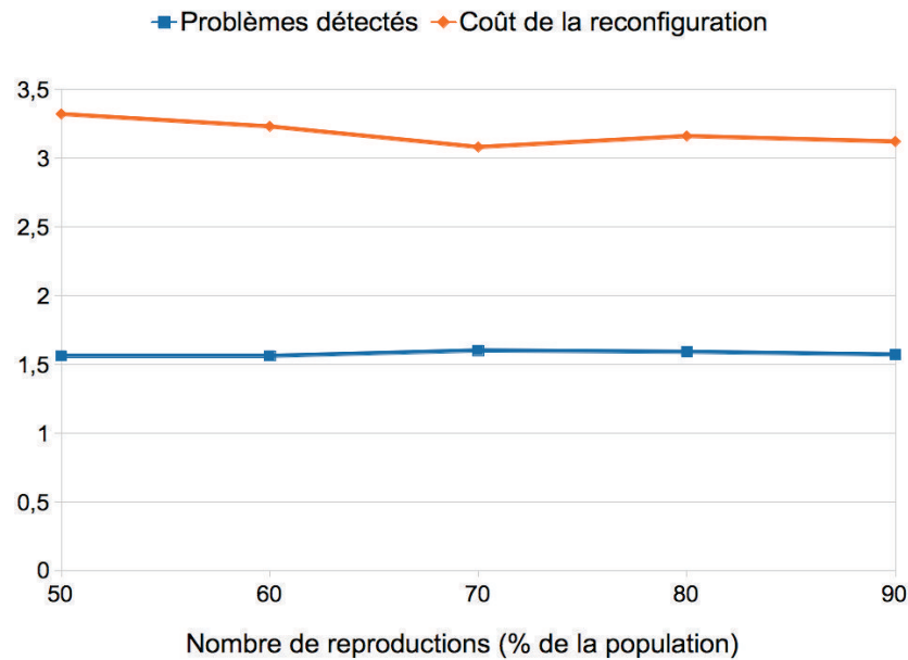
FIGURE 6.3 – Influence du nombre de reproductions
