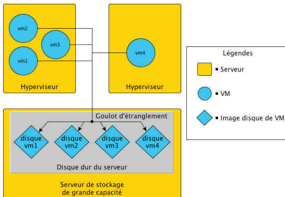
FIGURE 3.4 – Plusieurs hyperviseurs utilisent un même stockage pour faciliter l'administration de leurs VM
