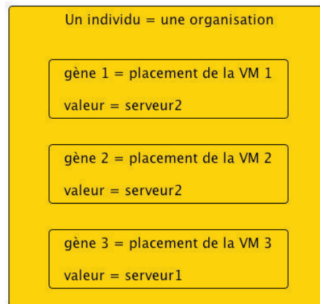
FIGURE 5.3 – Modélisation d'une organisation à l'aide d'un individu
