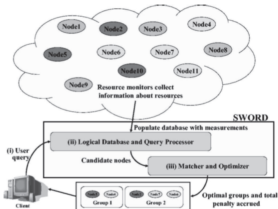
FIGURE 3.8 – Fonctionnement général de l’outil Sword
