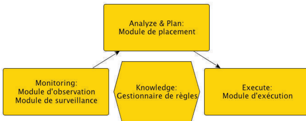
FIGURE 5.1 – Architecture MAPE-K utilisé par VMScript
