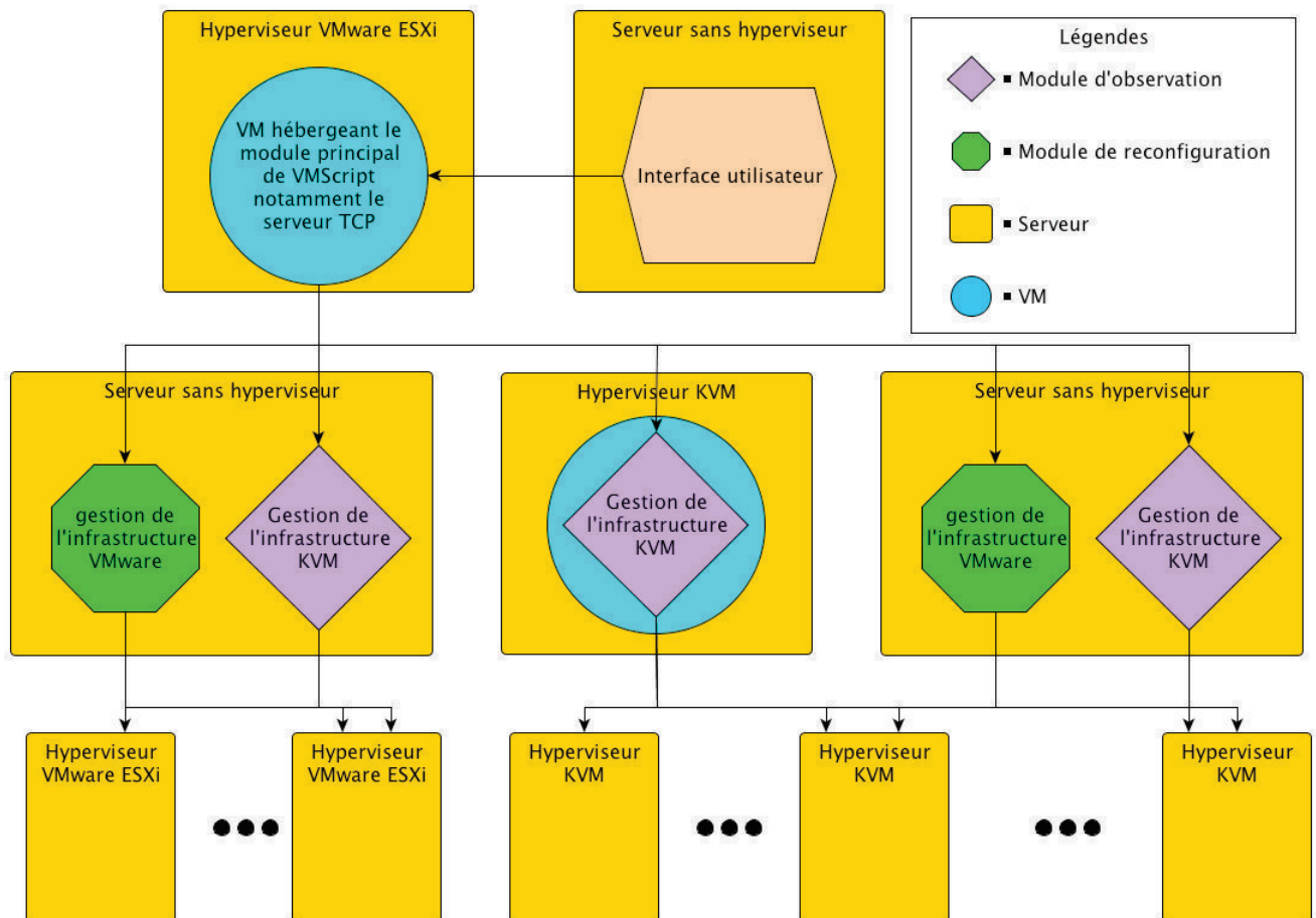
FIGURE 5.6 – Exemple d'architecture distribuée pour l'outil d'administration VMScript
