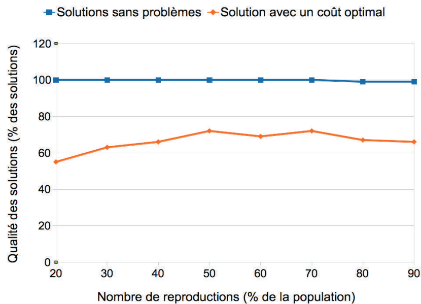
FIGURE 6.6 – Affinage du nombre de reproductions
