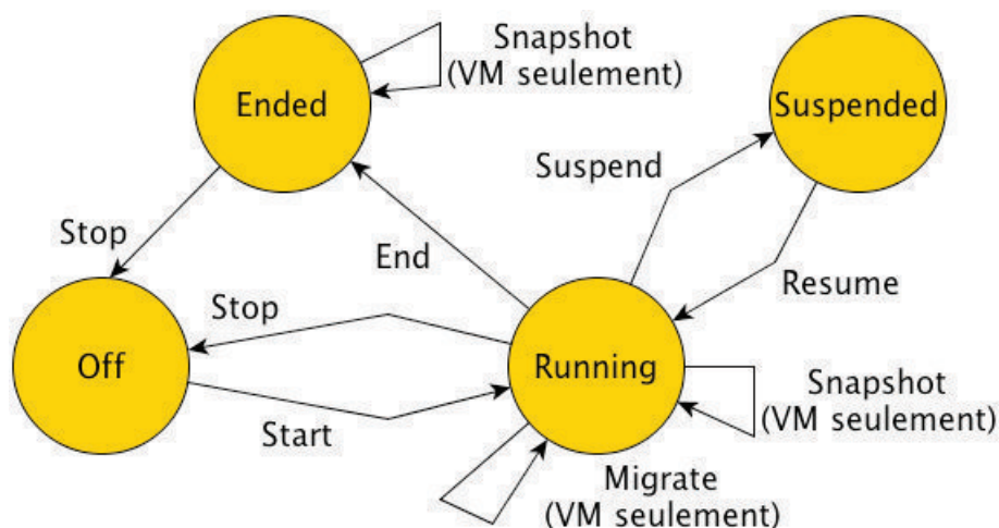
FIGURE 5.2 – Le cycle de vie d'un serveur ou d'une machine virtuelle. Les flèches montrent les reconfigurations modifiant l'état de la VM ou du serveur. L'état « ended » permet de spécifier que le serveur ou la VM doit être arrêté. Pour un serveur, cet état permet de programmer une maintenance. Le serveur doit être vidé de ses VM et ne peut pas accueillir de VM supplémentaires. Pour une VM, l'état « ended » permet à l'administrateur d'effectuer une sauvegarde avant l'extinction de la VM.
