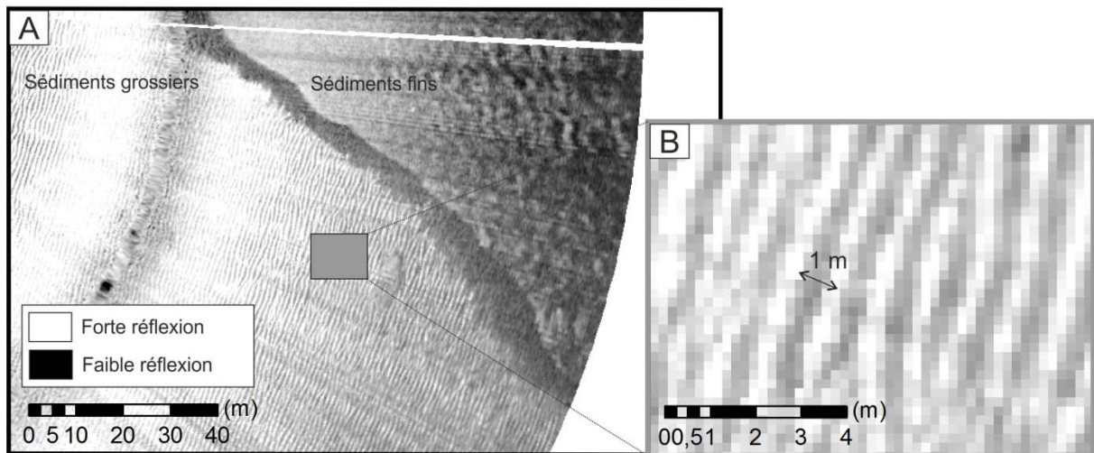
Figure III.14 : Profil sonar latéral. A : Vue d'ensemble à 20 m. B : Zoom sur un champ de rides de houle (longueur d'onde : 1 m, hauteur estimée : < 0,15 cm, D50 : ~2,2 mm). Pour la localisation se reporter à la Figure III.12-B.
