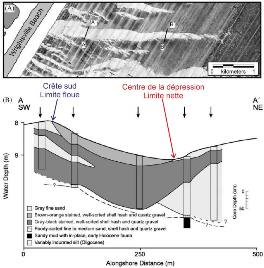
Figure I.23 : Carte (A) et section (B) montrant la morphologie et la stratigraphie des sorted bedforms présents sur la shoreface et le plateau continental interne au large de Wrightsville Beach, en Caroline du Nord (Murray et Thielert, 2004).
