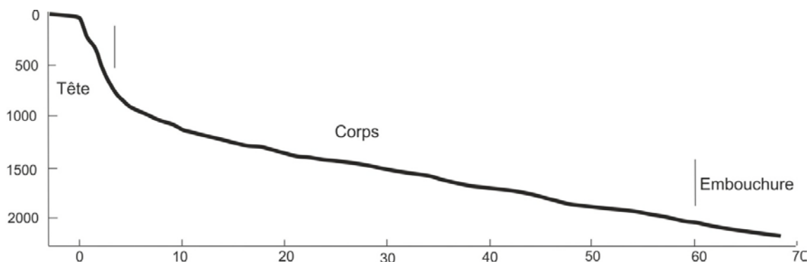
Figure I.34 : Profil « type » d'un canyon. Exemple du profil bathymétrique longitudinal de l'axe du canyon de Kaikoura (Nouvelle-Zélande). Modifié de Lewis et Barnes (1999).
