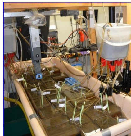
Figure IV.1 : Schéma et photographie présentant le plan expérimental avec les différentes conditions d'enrichissement et de temps de prélèvement, les différents paramètres mesurés et les répliqués (Rep).
