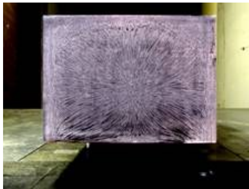
Figure 3.6 - Photographie de visualisation pariétale sur un corps de Ahmed à culot droit
