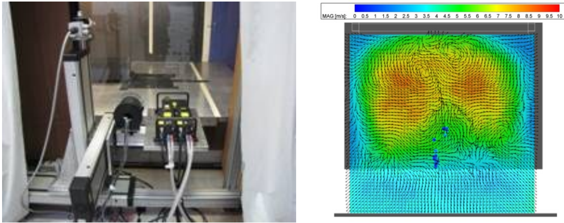
Figure 3.7 – À gauche : Laser du système PIV tirant dans le plan YZ à X=2H en aval du culot à travers une vitre en plexiglas bordant la section de la soufflerie. Le mat portant la caméra est situé en aval de l'écoulement et n'est pas visible sur cette photographie. À droite : Résultats après post traitements du champ de vitesse moyenné pour cette configuration de mesure.
