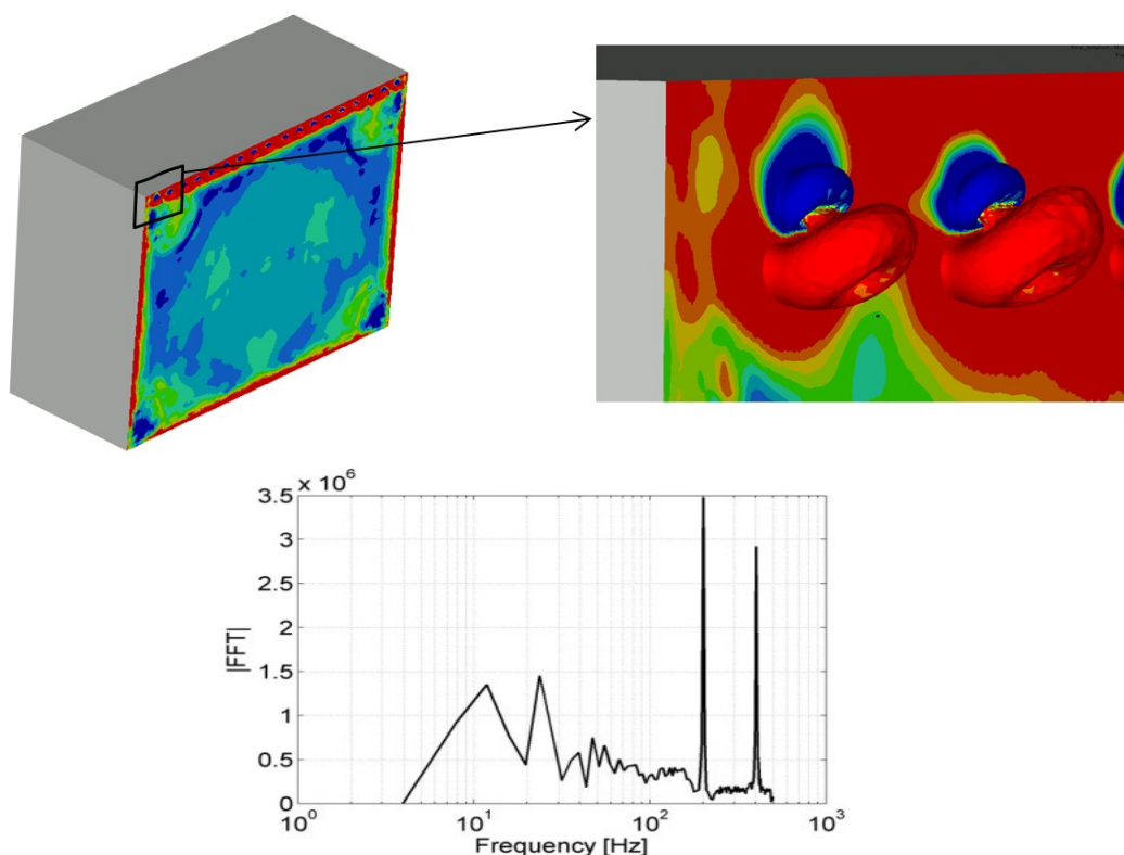
Figure 5.37 – Description du premier mode de pression fluctuante en sortie de jet et transformée de Fourier du coefficient modal associé
