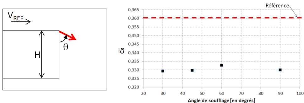
Figure 5.6 – Evolution du coefficient de la traînée moyen en fonction de l'angle de soufflage pour les configurations de contrôle par fente discontinue en partie supérieure du culot, pour une vitesse de jet fixée de V_{jet}=75m/s
