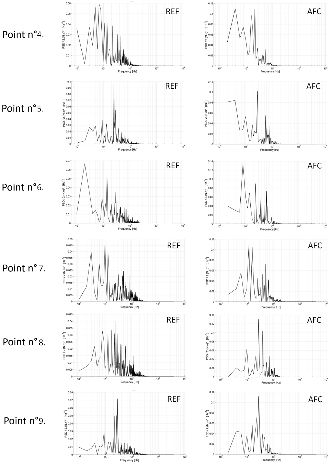
Figure 5.32 - Comparaison point à point des spectres dans le plan Y=0 . A gauche : cas de référence. A droite : cas avec contrôle
