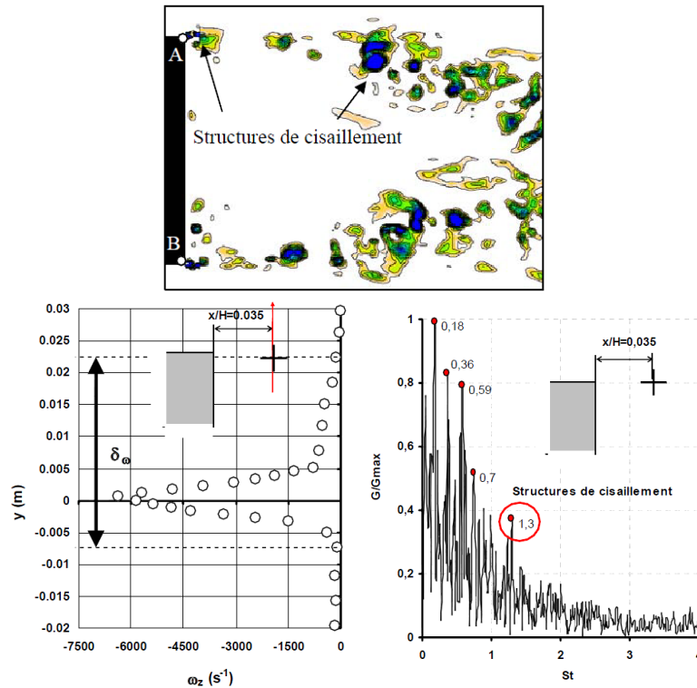
Figure 1.27 - Description d'une zone d'écoulement cisailé [Rou06]
