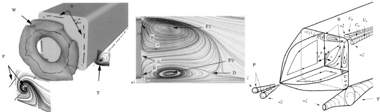
Figure 1.33 - Visualisation d'un isocontour de pression moyenne à l'arrière du culot (gauche) Lignes de courant moyennes dans le plan YO (centre) et topologie schématisée de l'écoulement (droite) [Kra03]
