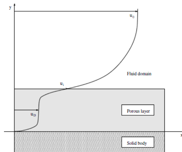
Figure 1.41 - Écoulement fluide autour d'un milieu poreux et profil de vitesse longitudinal associé
