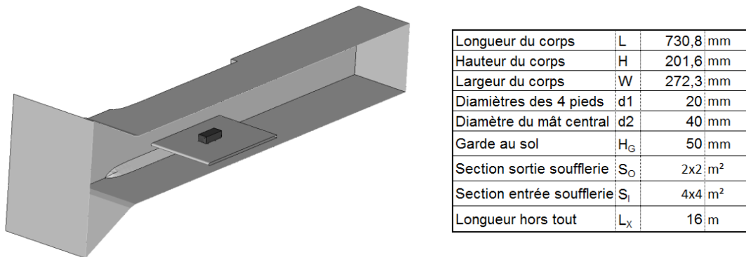
Figure 4.1 - Soufflerie reproduite en calcul. Le corps de Ahmed (en noir) est disposé sur une plaque au centre.
