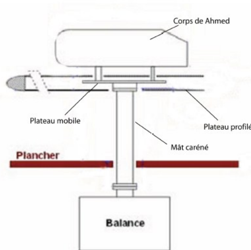
Figure 3.2 - Montage d'une maquette sur la balance aérodynamique
