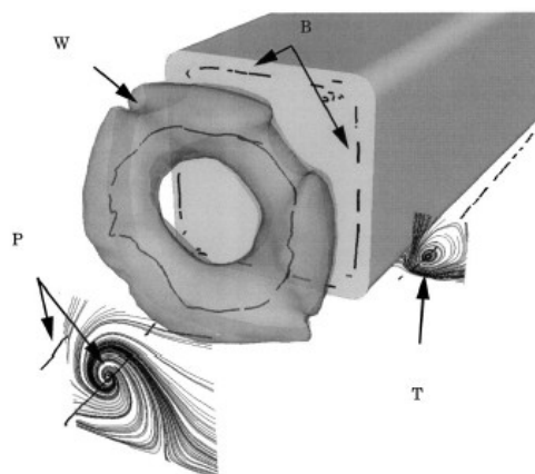
Figure 1.26 - Topologie de l'écoulement dans le sillage d'une géométrie de type culot droit [Kra03]
