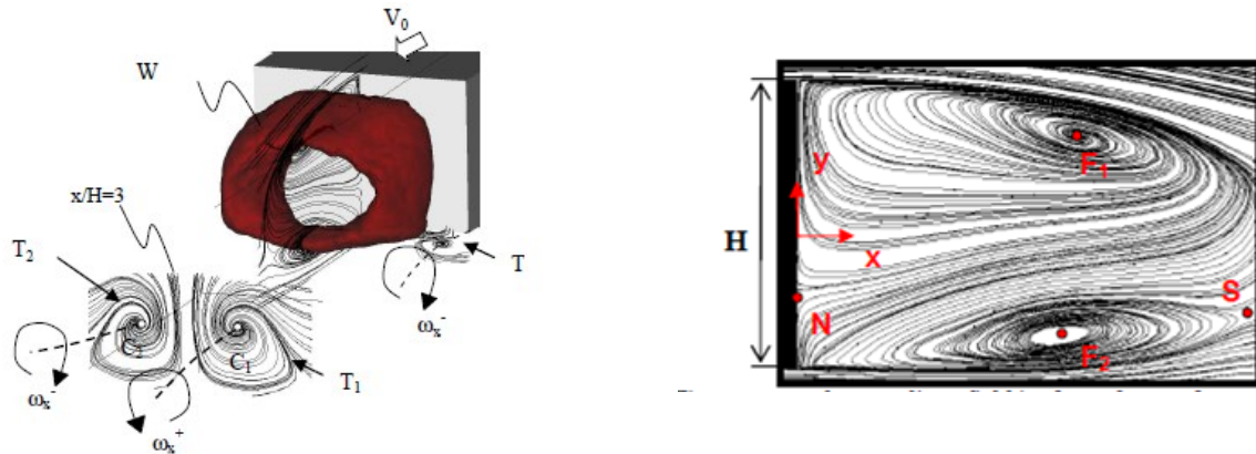
Figure 1.36 - Topologie de l'écoulement de sillage [Rou09]
