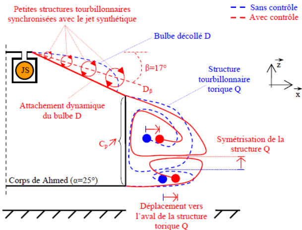
Figure 1.59 - Dispositif de jet synthétique (en haut) et représentation schématique de son effet sur le sillage (en bas) [Lec08]
