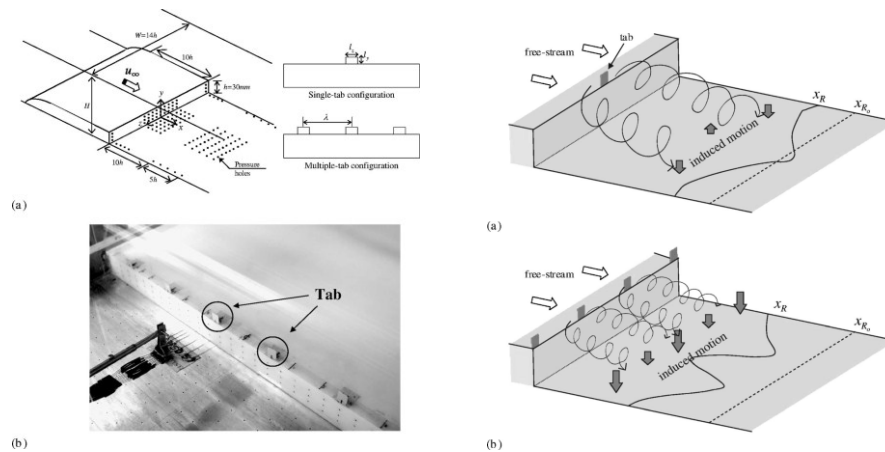
Figure 1.46 - Expérience de vortex generator sur une marche descendante à culot droit [Par07]
