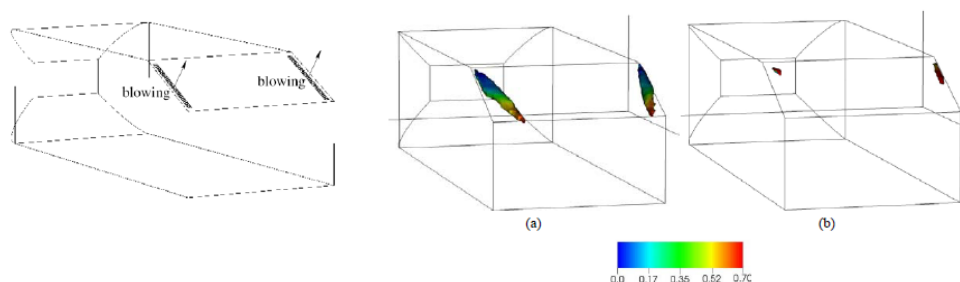
Figure 1.72 - Contrôle actif longitudinal (à gauche). Comparaison de coefficients de pression sans (a) et avec (b) soufflage [Bru11]
