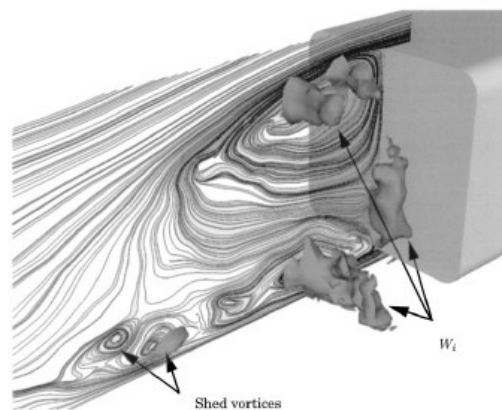
Figure 1.34 – Iso contour instantané de pression avec superposition de lignes de courant instantanées dans le plan YO [Kra03]
