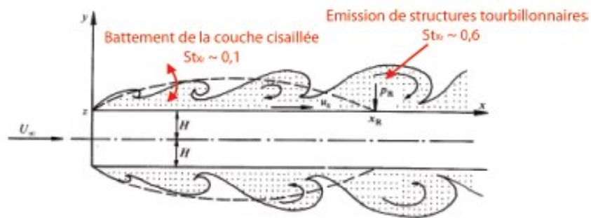
Figure 1.10 - Mécanismes instationnaires d'une couche limite se développant sur une plaque plane d'épaisseur 2H d'après Kiyama et al. [Kiy86]
