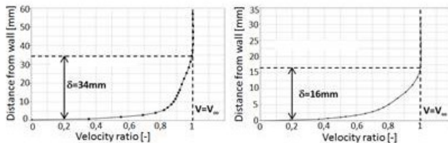
Figure 4.9 - Profils de vitesse dans la couche limite relevés en Y=0 (à gauche) et Z=H/2 (à droite)
