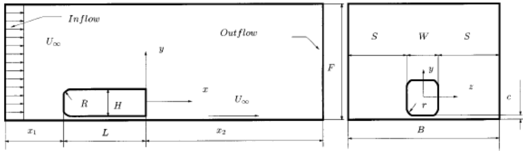
Figure 1.32 - Géométrie du 'bus shaped body' de Krajinovic [Kra03]
