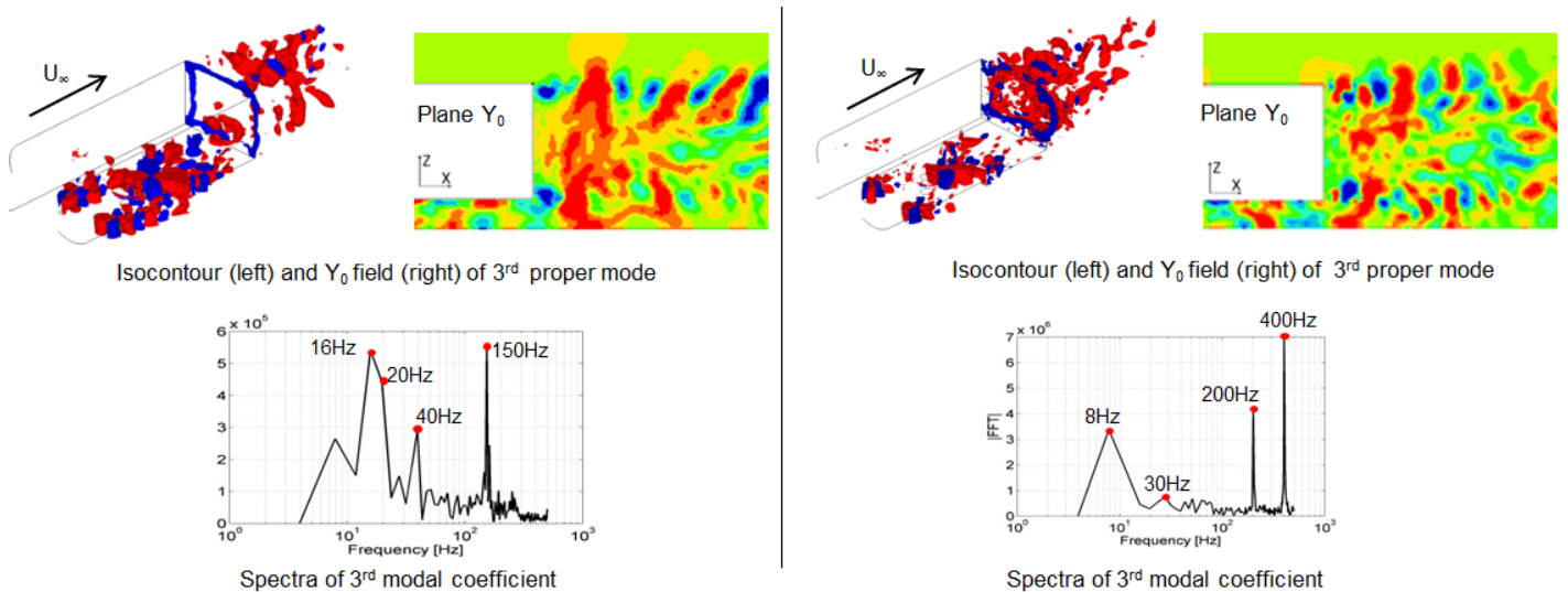
Figure 4.51 - Description du 3ème mode de pression fluctuante pour le cas de référence (à gauche) et le cas avec jet pulsé à 400Hz (à droite)
