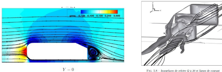
FIG. 5.8 - Isosurfaces de critère Q à 20 et lignes de courant
