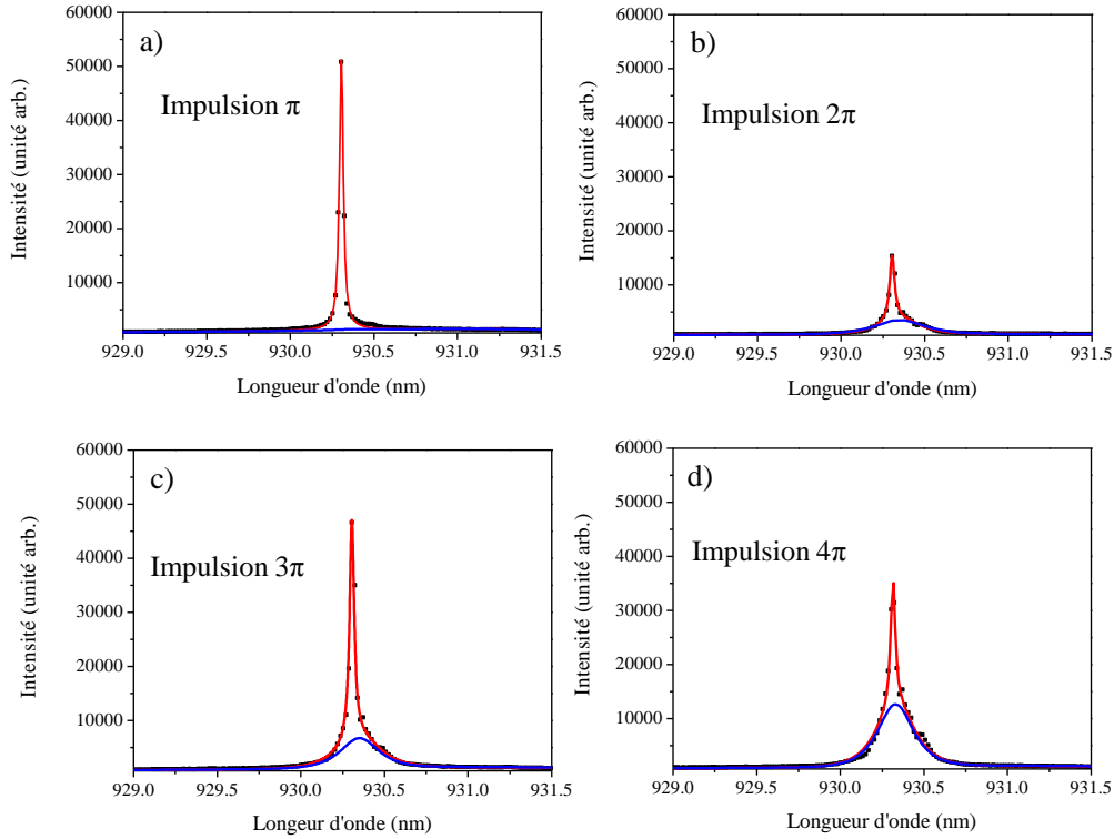
FIGURE 3.8 – Spectres de \mu -PL résonants de la boîte S1A pour différentes puissances d’excitation. Le laser est ajusté par une gaussienne en bleu et la luminescence est ajusté par une lorentzienne en rouge.
