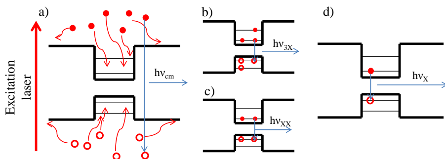
FIGURE 2.20 – Exemple de cascade radiative lorsque le laser génère un grand nombre de paires dans la couche de mouillage (a). Certaines paires peuvent se recombinaison radiativement (flèche bleu verticale) en émettant un photon (flèche bleu horizontale) à l'énergie de la couche de mouillage ( h\nu_{cm} ). D'autres relaxent non radiativement (flèches rouges) hors de la boîte observée, ou peuplent les niveaux de plus basse énergie de la boîte (b). Chaque paire va successivement se recombinaison (b et c), émettant un photon à une énergie différente de celle de l'exciton qui est le dernier à émettre (d).
