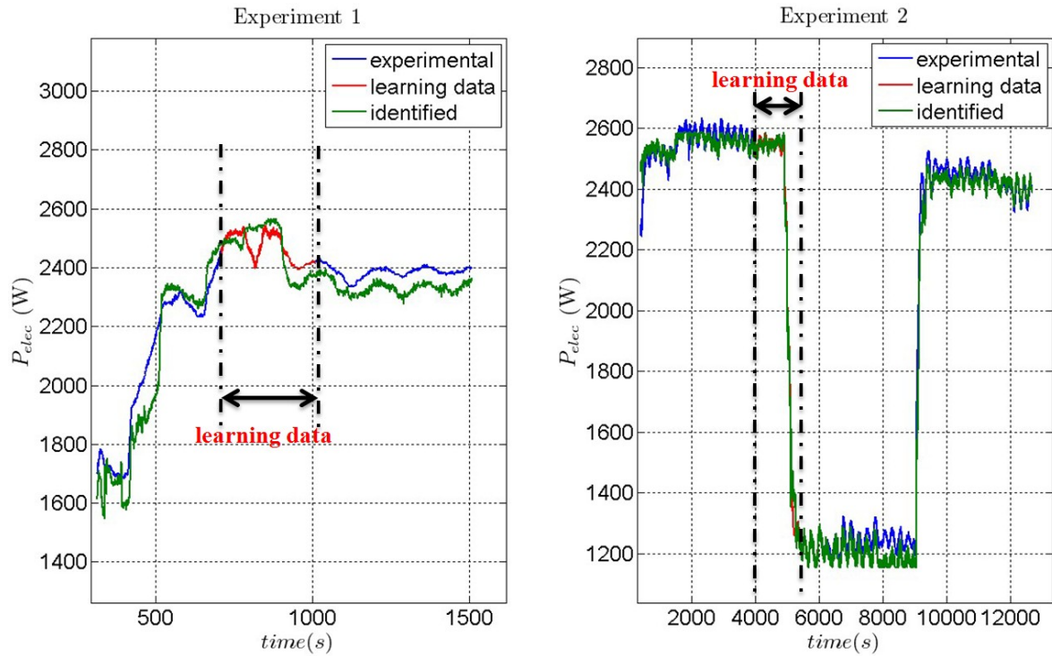
(a) Profils temporels des puissance électrique P_{elec} mesurée et identifiée sur l'ensemble des données d'apprentissage et de validation.
