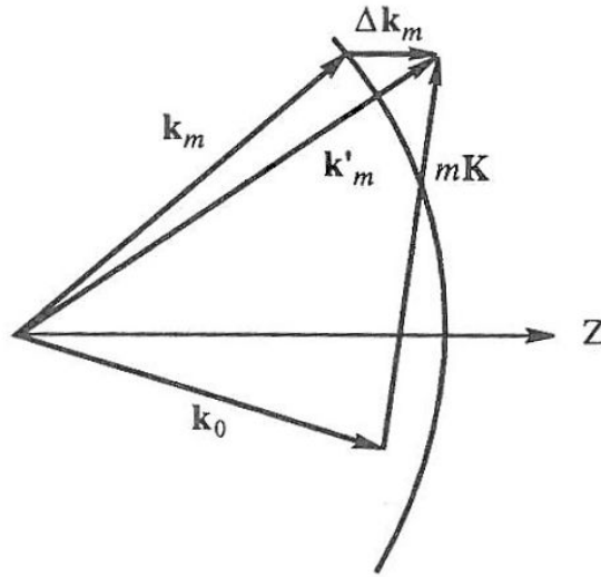
FIGURE 2.2 – Représentation du désaccord de phase entre k'_m et k_m [40].
