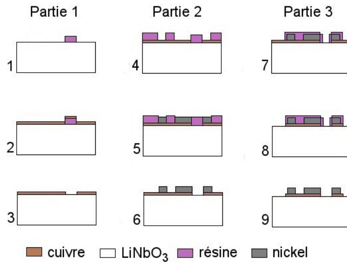
FIGURE 3.10 – Diagramme de procédé complet pour la réalisation des HAR IDTs. Partie 1 : dépôt du plan de masse de cuivre, partie 2 : électroformage, partie 3 : gravure de l'excédent de cuivre
