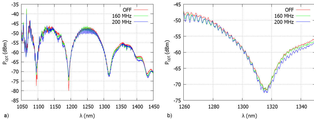
FIGURE 5.19 – Transmission spectrale du modulateur 576-52 avec excitation du transducteur à des fréquences autres que les fréquences de résonance avec une puissance de 20 dBm. (a) Spectre complet, (b) spectre centré sur le creux à environ 1317 nm.
