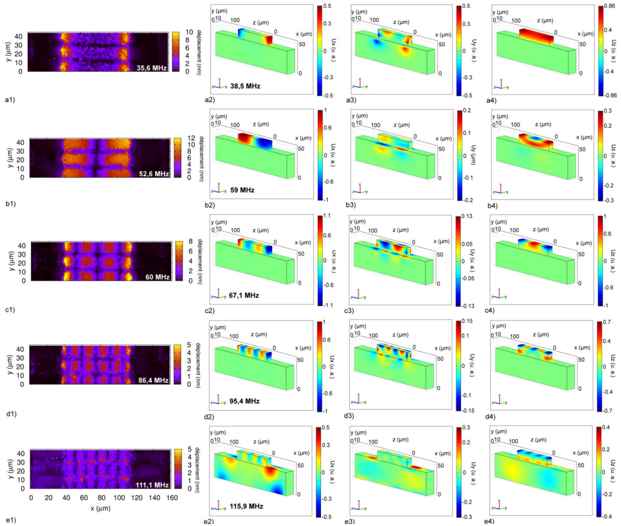
FIGURE 3.18 – Comparaison entre les résultats expérimentaux et les résultats de la simulation périodique 3D par éléments finis des modes de vibration d’une électrode simple d’une longueur de 72 \mu\text{m} , d’une hauteur de 13,7 \mu\text{m} et d’une largeur de 9 \mu\text{m} . Les images d’indice 1 représentent le relevé expérimental du déplacement selon x pour seulement trois électrodes. Les images d’indice 2, 3 et 4 représentent le déplacement obtenu par simulation périodique selon les axes x , y et z respectivement. La barre de couleur correspondante représente l’amplitude de déplacement normalisée par rapport à un déplacement de 3,3 \text{ nm} d’amplitude. Les axes x , y et z correspondent aux axes cristallographiques. Les images a, b, c, d et e montrent respectivement les déplacements pour les modes A, B, C, D et E de la Figure 3.13(a).
