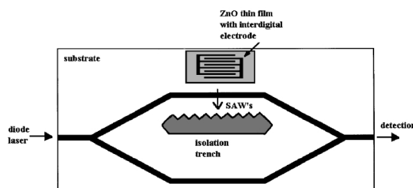
FIGURE 2.8 – Schéma d'un modulateur acousto-optique intégré sur silicium. Une onde acoustique interagit avec un seul bras d'un interféromètre de Mach-Zehnder [94].
