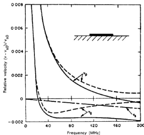
FIGURE 1.18 – Courbes de dispersion montrant l’évolution de la vitesse de phase ( v_p ) et de la vitesse de groupe ( v_g ) pour une couche de 50 nm d’aluminium sur un substrat de niobate de lithium. Les courbes solides montrent la variation due à l’effet de court-circuit seul alors que les courbes pointillées incluent l’effet de charge massique représenté par la courbe v_s . D’après [23].
