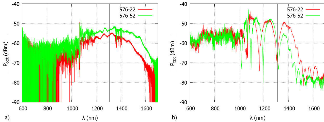
FIGURE 5.9 – Transmission spectrale mesurée en lumière blanche pour les 2 cellules retenues pour les tests de modulation. Les deux cellules ont un HAR IDT d'ouverture acoustique 16\lambda et le guide optique partiellement recouvert par un doigt. La ligne verticale correspond à une longueur d'onde d'environ 1309 nm. (a) Transmission des guides droits. (b) Transmission des interféromètres de Mach-Zehnder.
