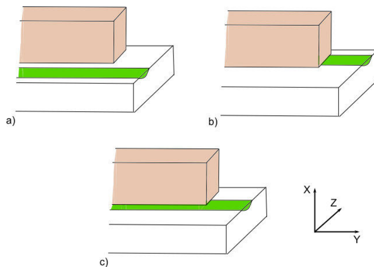
FIGURE 5.5 – Schémas des 3 positions utilisées du guide optique par rapport aux doigts du HAR IDT. (a) Guide entre les doigts, (b) guide sous un doigt et (c) guide à moitié sous un doigt.
