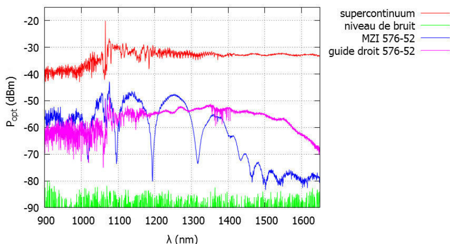
FIGURE 5.10 – Comparaison entre les spectres du supercontinuum mesuré en fibre à fibre, de bruit de l’analyseur, du MZI 576-52 et du guide droit associé à ce dernier.
