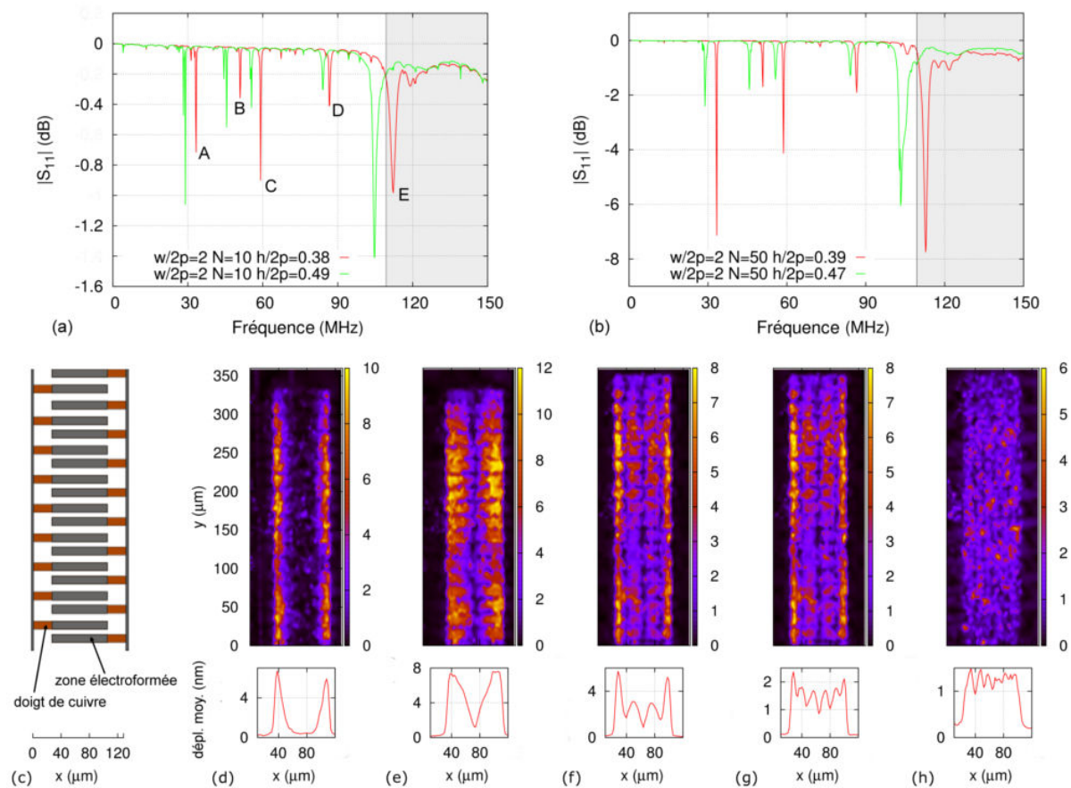
FIGURE 3.13 – (a) et (b) Mesures du paramètre S_{11} pour des HAR IDTs ayant une ouverture acoustique de 72\ \mu\text{m} ( 2\lambda ) et possédant (a) 10 paires de doigts et (b) 50 paires de doigts. (c) Schéma représentatif de la zone balayée lors des mesures par sonde optique. (d), (e), (f), (g) et (h) Mesures des déplacements mécaniques hors plan induits par les modes résonants de la courbe correspondant à un h/2p de 0,38 présente sur la mesure S_{11} de peignes à 10 paires de doigts. (d) Mode A à 35,6 MHz; (e) mode B à 52,6 MHz; (f) C à 60 MHz; (g) mode D à 86,4 MHz; (h) mode E à 111.1 MHz.
