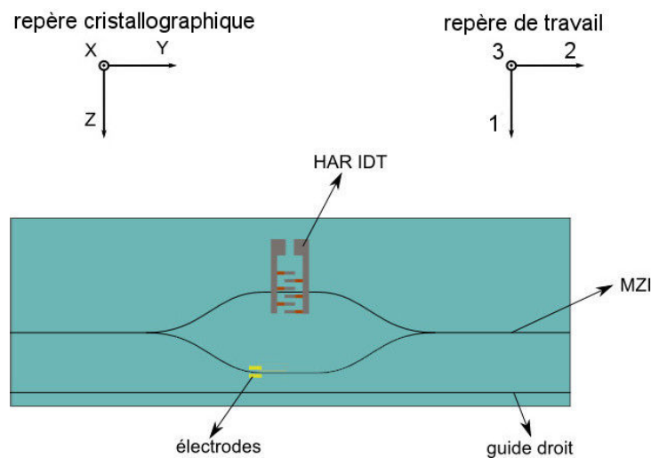
FIGURE 5.4 – Schéma d'une cellule contenant un guide optique droit et un interféromètre de Mach-Zehnder réalisé avec un HAR IDT disposé sur un bras et des électrodes déposées autour du second bras. Le repère cristallographique définit les axes du cristal et le repère de travail est le repère défini par la Figure 1.6 servant aux calculs.
