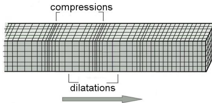
FIGURE 1.2 – Représentation des déplacements induits par une onde élastique de polarisation longitudinale.
