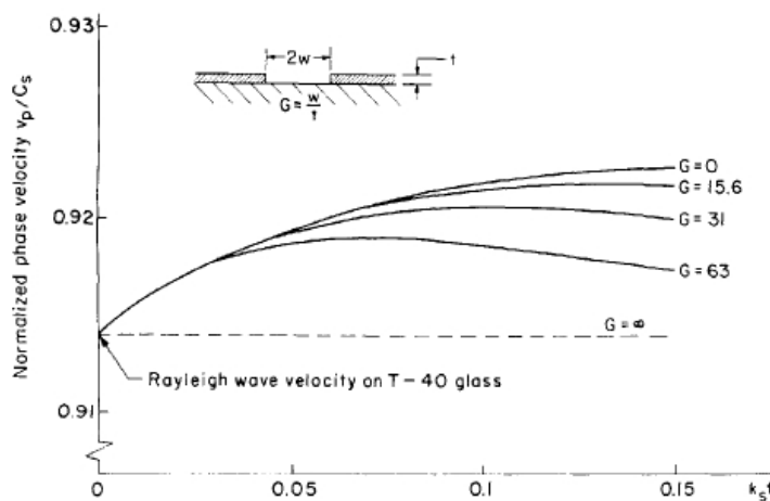
FIGURE 1.19 – Courbes de dispersion pour un mode des guides montrés sur la Figure 1.14(c) sur un substrat de verre T-40 et pour différents rapports d'aspect. C_s est la vitesse des ondes de volume dans le substrat et k_s est le nombre d'onde. D'après [23].
