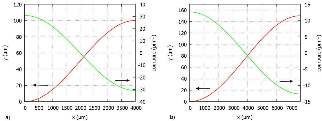
FIGURE 5.3 – En rouge, tracé de la courbe dessinant une séparation en cosinus (5.9). En vert, tracé de la courbure (5.10) correspondante. (a) Jonction définie d'après [146] avec h = 100 \mu\text{m} et L = 4000 \mu\text{m} . (b) Jonction définie pour les MZIs réalisés au cours de ces travaux avec h = 150 \mu\text{m} et L = 7650 \mu\text{m} .
