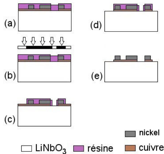
FIGURE 3.9 – Étapes du procédé de gravure du cuivre et du chrome.
