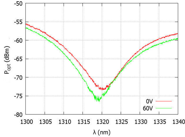
FIGURE 5.11 – Spectres avec 0 et 60 V appliqués au électrodes. Les tracés sont centrés sur le creux à 1317 nm du spectre 576-52 de la Figure 5.9.
