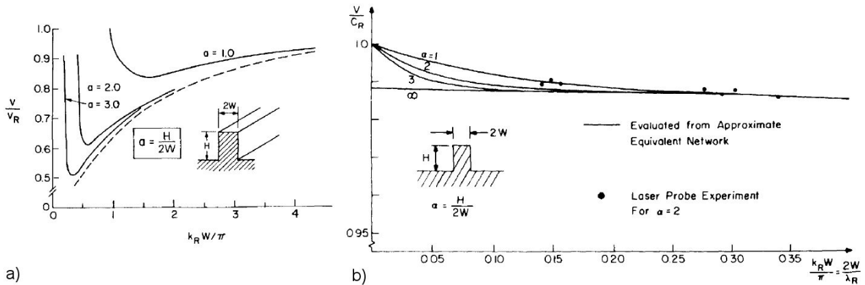
FIGURE 1.15 – Courbes de dispersion des modes anti-symétriques et symétriques dans une arête rectangulaire. a) Mode anti-symétrique, b) mode symétrique. D’après [23].
