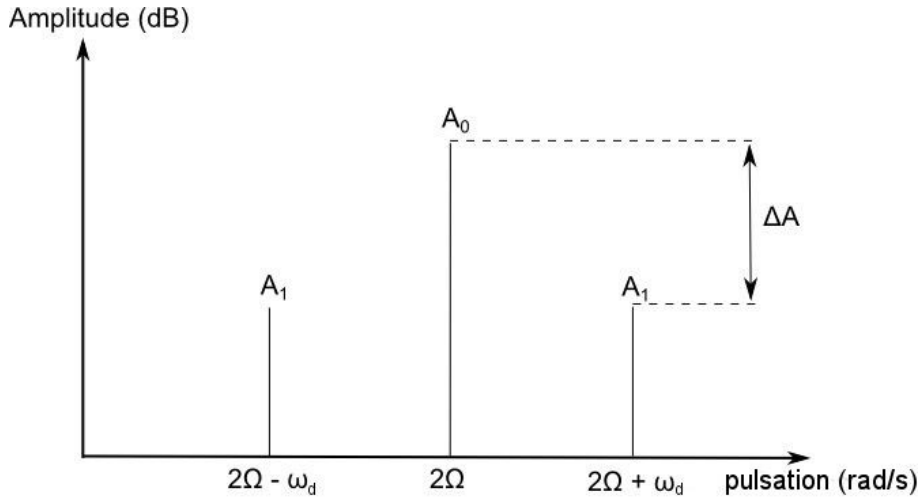
FIGURE B.3 – Spectre de puissance issu de l'interférence entre le signal sonde et le signal référence dans le cas où u \ll \lambda . Il possède une raie centrale à 2 fois la fréquence du modulateur acousto-optique et 2 raies latérales décalées de plus ou moins la fréquence de l'onde acoustique traversant l'échantillon mesuré.
