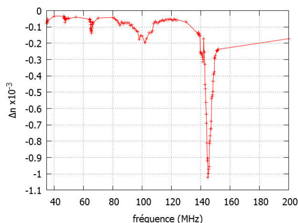
FIGURE 5.20 – Évolution de la variation d’indice de réfraction correspondant au décalage de longueur d’onde du spectre cannelé en fonction de la fréquence appliquée au HAR IDT pour une puissance RF de 20 dBm.
