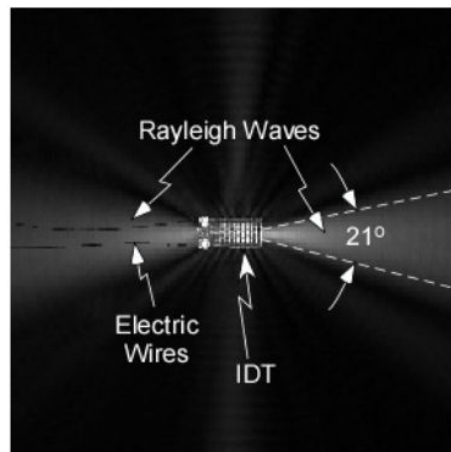
FIGURE 1.9 – Image de l'onde de Rayleigh générée par un IDT, extraite de [10].
