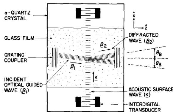
FIGURE 2.7 – Schéma de l'expérience réalisée par Kuhn et al. d'une déflexion optique par une onde acoustique de surface dans une couche mince de verre déposée sur un substrat de quartz [91].
