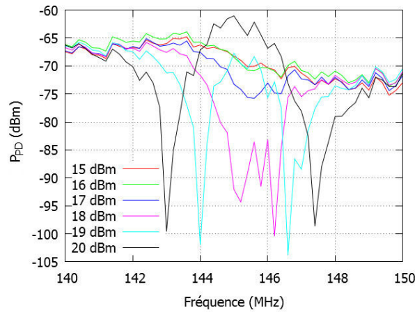
FIGURE 5.16 – Évolution de la puissance électrique mesurée en sortie de la photo-diode P_{PD} en fonction de la fréquence appliqué au HAR IDT sur une bande s'étendant de 140 à 150 MHz.
