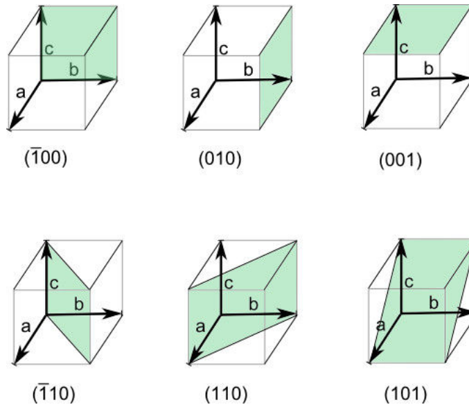
FIGURE C.2 – Représentations de quelques plans d'une structure cubique.
