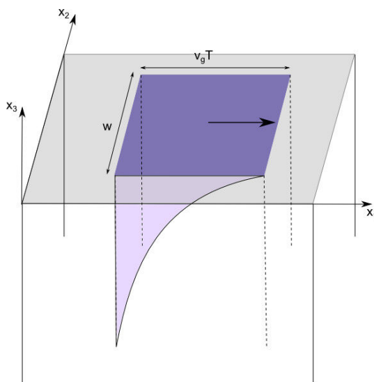
FIGURE 4.1 – Représentation de la décroissance de l'énergie acoustique dans la profondeur. v_g désigne la vitesse de groupe, T le temps pendant lequel l'onde se propage et w la largeur du faisceau.
