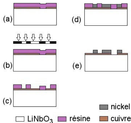
FIGURE 3.7 – Étapes du procédé d'électroformage de nickel.
