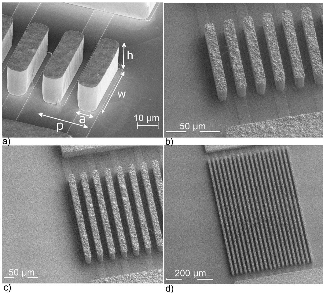
FIGURE 3.11 – Images prises au microscope électronique à balayage d'HAR IDTs après toutes les étapes de fabrication. (a) Peigne avec h/2p = 0,43 , w/2p = 1 , p = 18 \mu\text{m} et a = 9 \mu\text{m} . (b) Peigne avec w/2p = 2 . (c) Peigne avec w/2p = 4 . (d) Peigne avec w/2p = 16
