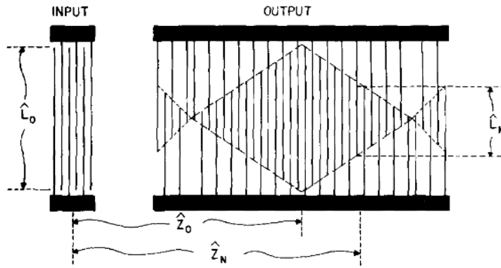
FIGURE 1.11 – Schéma de la structure proposée par Szabo et al. [11] permettant de corriger la diffraction du faisceau acoustique. La correction se fait en optimisant la valeur de L_N .
