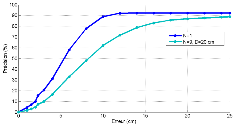
FIGURE 4.7: Comparaison des fonctions de distribution cumulative de l'erreur de localisation pour N \in \{1, 9\} et f = 200Hz .
