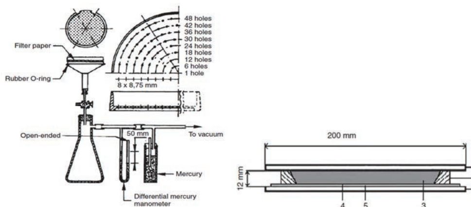
Figure 4 : Schéma de principe de la mesure de rétention d'eau selon l'ASTM C 1506-09
