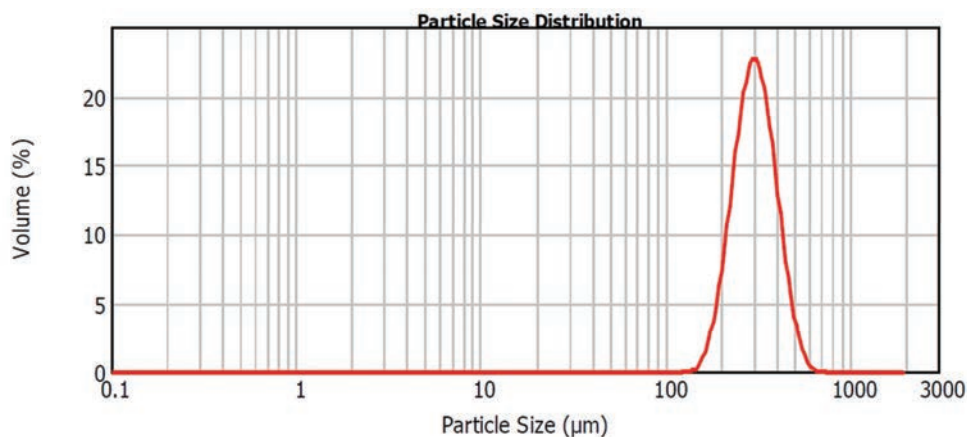
Figure II- 5 : Répartition granulométrique du sable Durance DU 0,1/0,35_ Mesure en voie sèche 0,5 bars, 30% d'obscuratation
