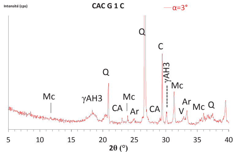
Figure II- 22 : GIRDX du CAC G 1 C _ \gamma AH 3 : gibbsite ; Mc : Monocarboaluminate ; Q : quartz ; V : vatérite ; C : Calcite ; Ar : Aragonite
