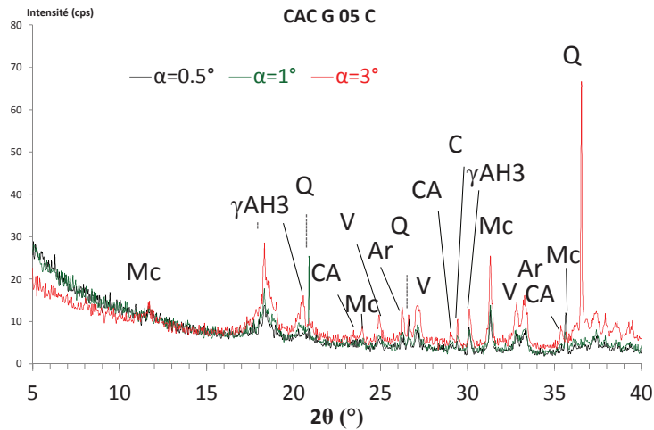
Figure II- 21 : GIRDX du CAC G 05 C _ \gamma AH 3 : gibbsite ; Mc : Monocarboaluminate ; Q : quartz ; V : vatérite ; C : Calcite ; Ar : Aragonite
