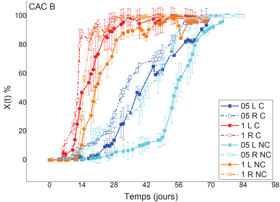
Figure III- 17 : Taux de recouvrement des éprouvettes de CAC B
