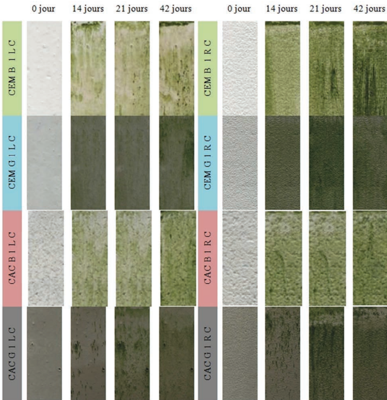
Figure III- 36 : Comparaison visuelle de la biodéterioration des éprouvettes carbonatées de E/C=1
