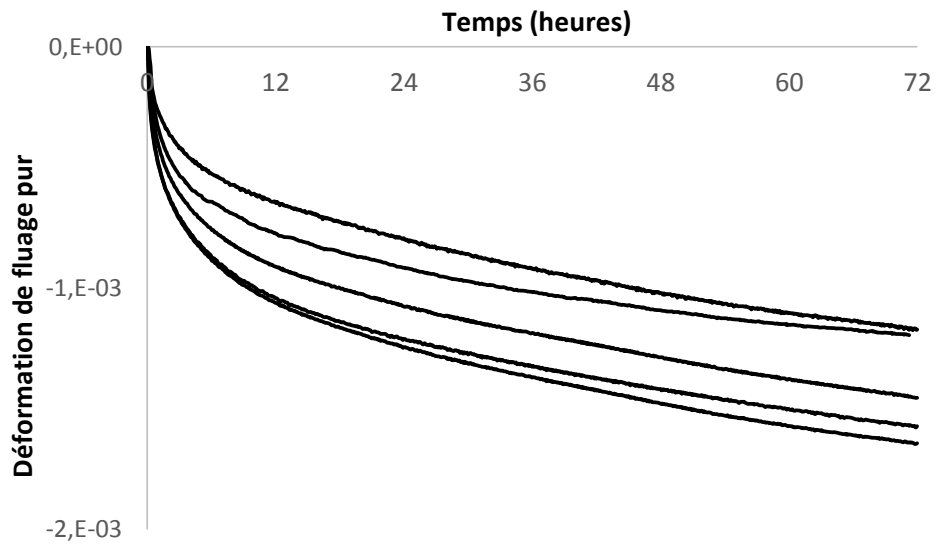
Figure 56 : Déformations différées mesurées à 20°C
