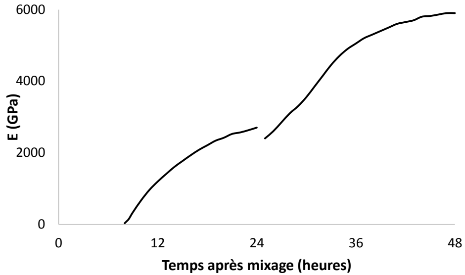
Figure 68 : Résultats de module d'Young en compression mesurés à la DMA à 20°C
