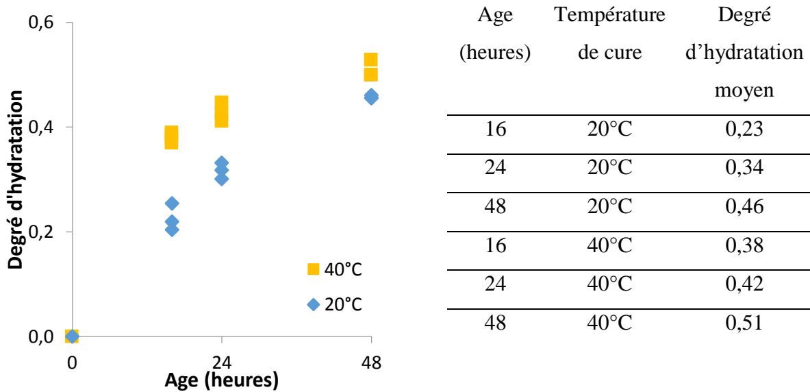
Figure 5 : Degré d'hydratation mesuré par séchage en fonction de l'âge et de la température de cure
