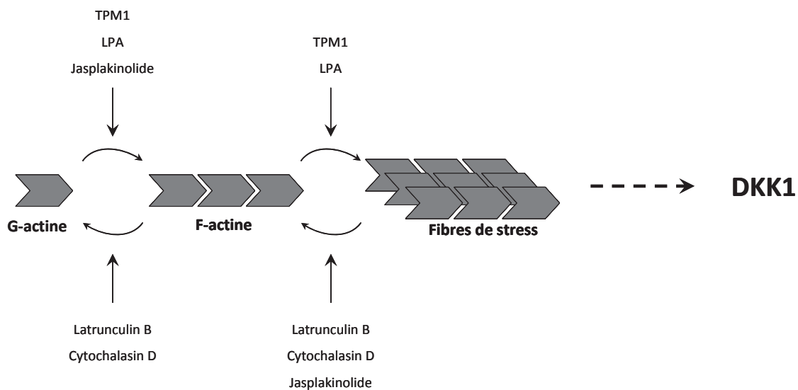
Figure : Résumé des principaux résultats concernant le mécanisme de régulation de Dikkopf-1 (DKK1) par la ténascine-C (TNC) et ses conséquences.
