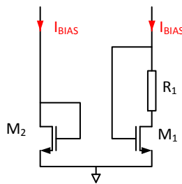
Figure 2.34 : Schéma de test.
