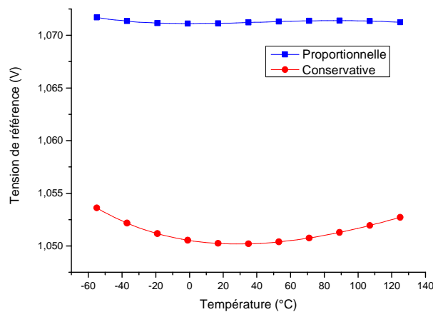
Figure 2.18 : Variation de la tension de référence à la température pour les deux configurations.
