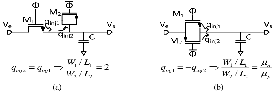
Figure 3.10 : Compensation de l'injection de charges par l'ajout d'un transistor factice (a) et d'un transistor complémentaire (b).
