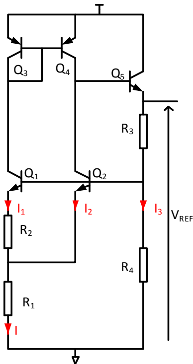
Figure 2.3 : Référence de tension bandgap de Brokaw
