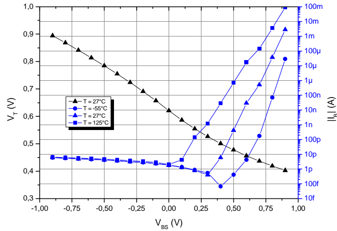
Figure 2.11 : Evolution de la tension de seuil et de la valeur absolue du courant du bulk en fonction de la polarisation du potentiel de bulk référencé à la source d'un transistor NMOS de dimensions W = 2 \text{ um} et L = 1 \text{ um} .
