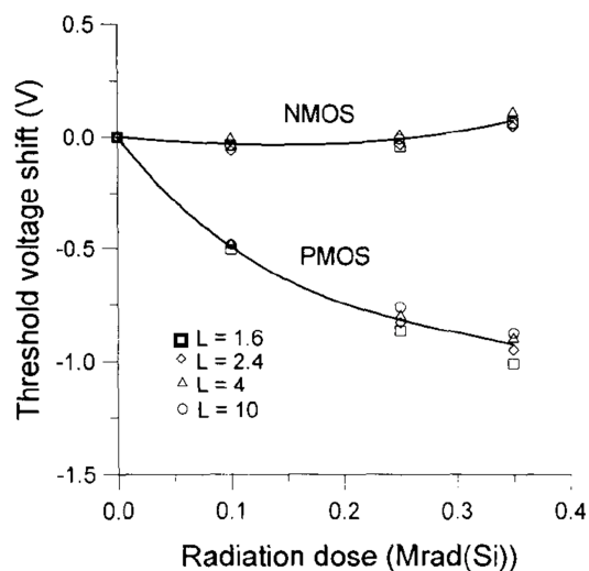
Figure 1.11 : Dérive de la tension de seuil due à la dose pour des transistors de type NMOS ( W=10 \text{ nm} ) et PMOS ( W=20 \text{ nm} ).
