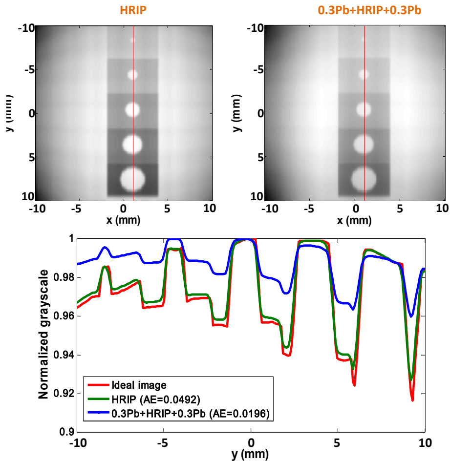
Figure 17: Résultat de simulation sans prendre en compte l'effet de la lecture optique. En haut images latentes obtenues avec les deux configurations de détecteur, et en bas, profils de niveaux de gris le long de la ligne indiquée en rouge dans les images. Le profil idéal représente le profil obtenu dans l'image spectrale de l'objet " Obj(x, y, z) ".
