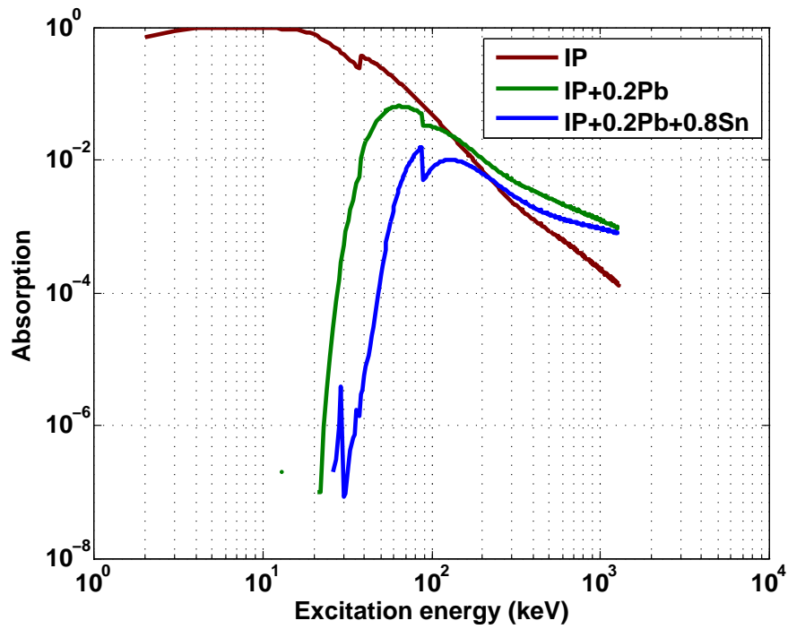
Figure 7: L'efficacité de l'absorption des photons en fonction de l'énergie pour les configurations différentes du détecteur.
