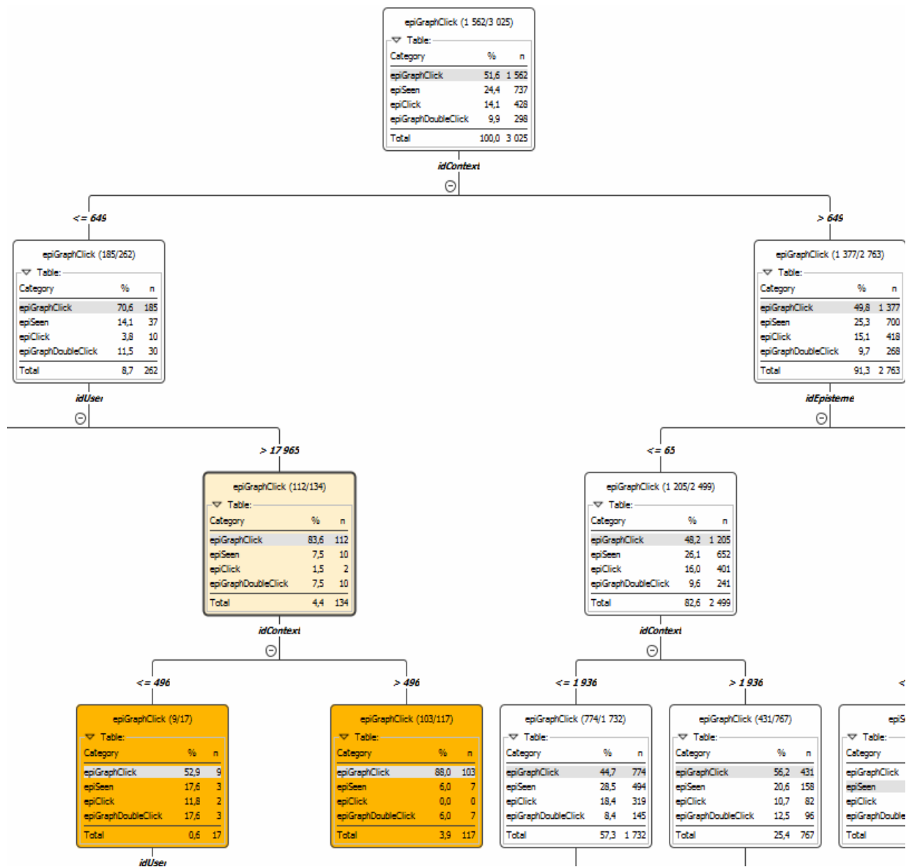
Figure 86 : arbre partiel de décision généré par Knime
