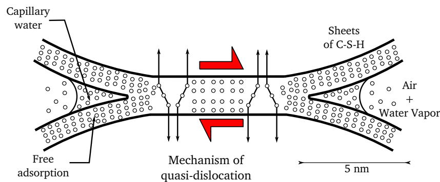
FIGURE 4.5: Mécanisme de glissement des feuilletts C-S-H [Ulm et Acker, 1998]
