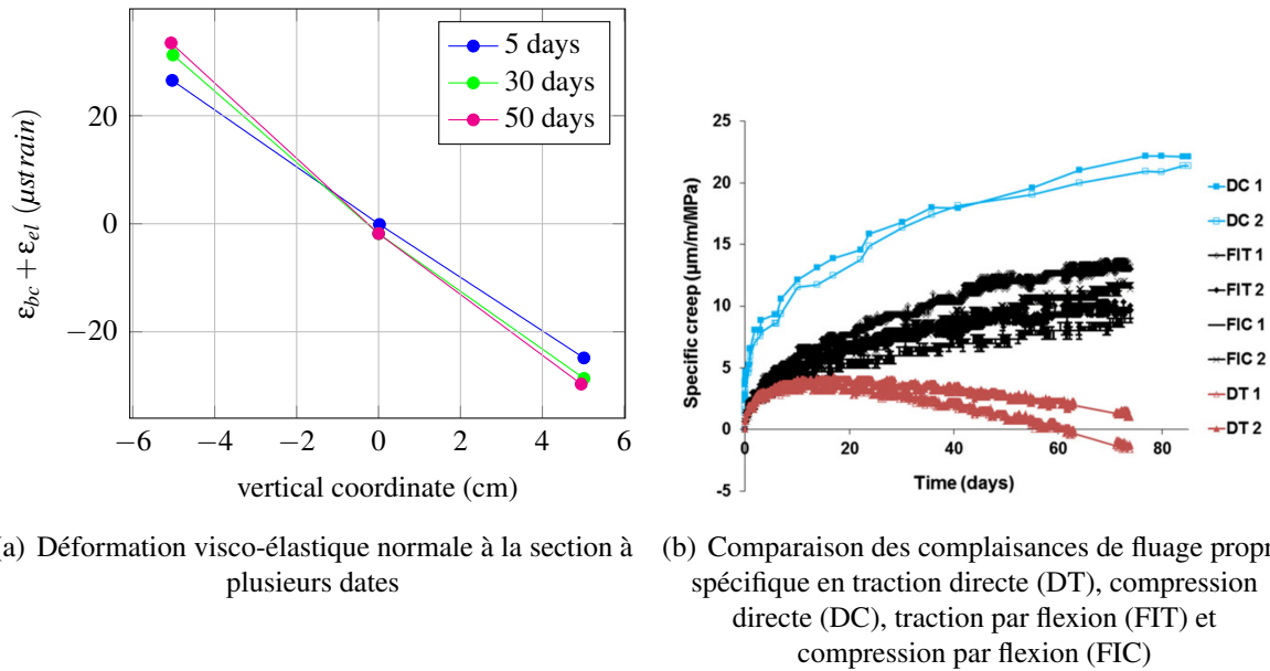
FIGURE 10.1: Fluage d'une poutre sous chargement maintenu [Ranaivomanana et al. , 2013a]
