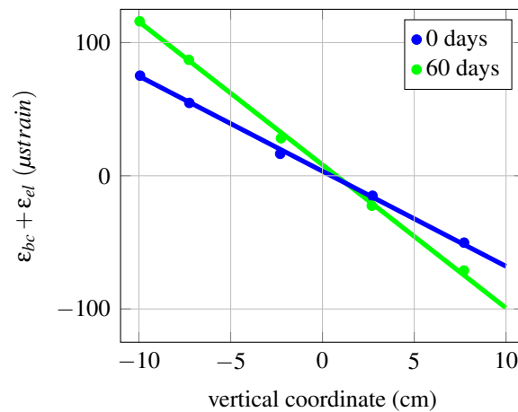
FIGURE 10.2: Déformation visco-élastique normale à la section à plusieurs dates [Tailhan et al. , 2013]
