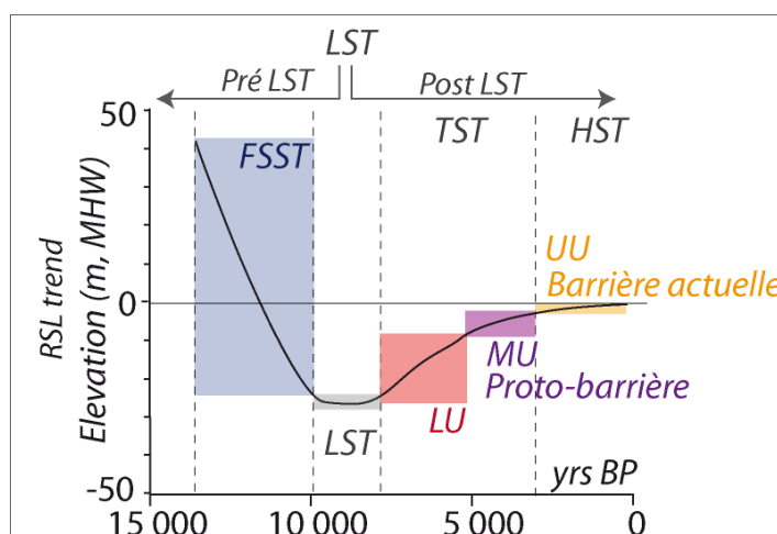
Figure VI-5 : Courbe de l'évolution du RSL pour le sud-est de Terre-Neuve (d'après Bell et al. (2003)) soulignant les périodes supposées de dépôts des différentes unités sismiques observées sur l'archipel lors de la chute du RSL (FSST: falling stage system tract), du bas niveau marin (LST: lower system tract), de la hausse du RSL (TST: transgressive system tract; unités LU, MU et la proto barrière) et le haut niveau marin (HST: high system tract, UU et la barrière actuelle).
