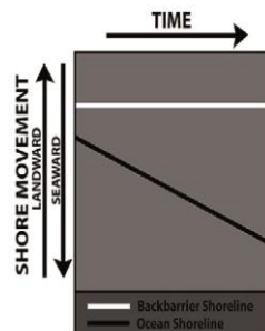
Figure I-7: Modèles stratigraphiques des barrières A) aggradantes, B) transgressives et C) régressives (d'après Galloway and Hobday, 1983; dans Timmons et al., 2010), ainsi que l'évolution de leur trait de côte (côté mer et côté lagune) au cours du temps.
