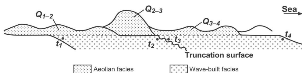
Figure I-27 : Schéma d'une section de beach ridges , montrant les relations chrono-stratigraphiques entre la progradation de la plage et la construction des dunes éoliennes (Espanberg spit, Chulchi, Alaska dans Tamura (2012) d'après Mason et al. (1997)), avec t_{1-4} pour les âges de dépôts et Q_{1-4} pour les quantités de sables éoliens accumulés.
