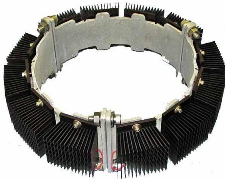
Figure 4.20: Système de conversion thermoélectrique sous forme d'anneau [Marlow Industries].
