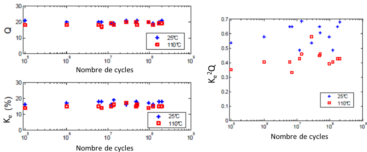
Figure 6.16: Evolution du facteur de qualité mécanique, du facteur de couplage et du produit K_e^2 Q en fonction du nombre de cycles pour une sollicitation de 600 V crête à crête (test fait par P.J. Cottinet/ LGEF).
