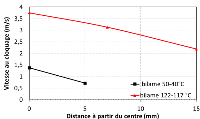
Figure 2.14: Vitesses au cloquage en fonction de la distance au centre pour un bilame 50-40 °C et un bilame 122-117 °C.
