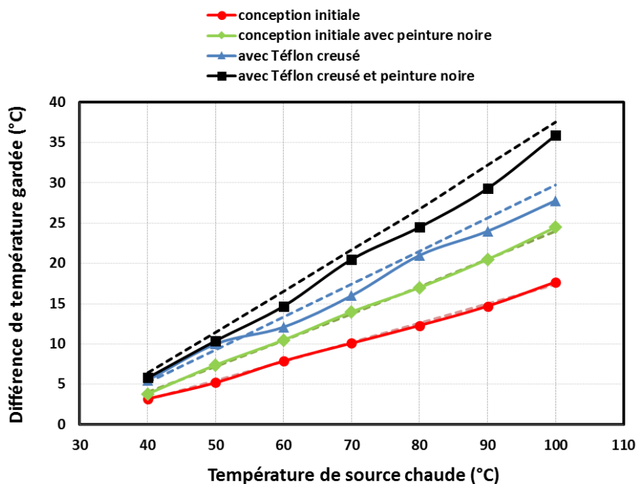
Figure 4.42: Différence de température gardée par le corps d'une cellule en fonction des étapes d'optimisation. Les traits pleins correspondent aux mesures et les traits interrompus correspondent au modèle analytique.
