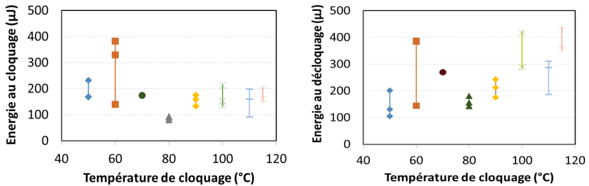
Figure 2.15: Energie développée au cloquage est au décroquage par des bilames de dimension 36 \times 18 \times 0.3 \text{ mm}^3 ayant une hystérésis autour de 3^\circ\text{C} . Les valeurs sont données en fonction de la température de cloquage.
