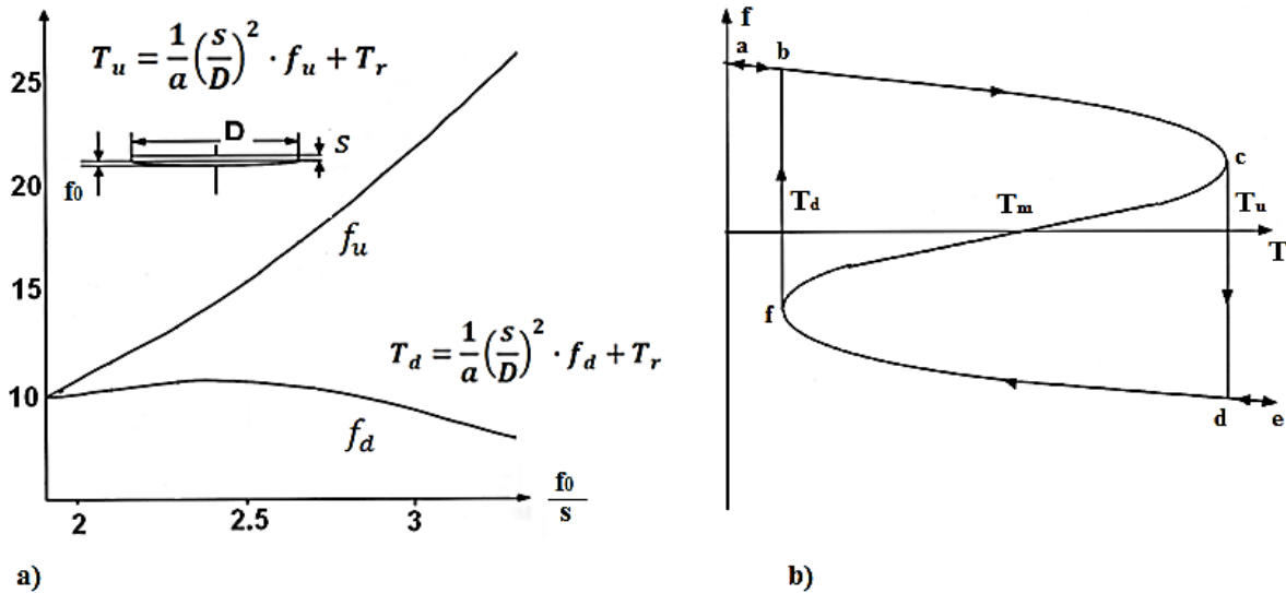
Figure 2.4: a) évolution des paramètres f_u et f_d avec le rapport flèche initiale/épaisseur ; b) flèche d'un disque cloquant en fonction de la température [30].
