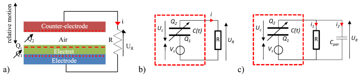
Figure 3.2: Récupérateur d’énergie mécanique à base d’électrets : a) schéma de la structure avec charge résistive en sortie ; b) modèle électrique équivalent ; c) modèle électrique avec capacité parasite [10].
