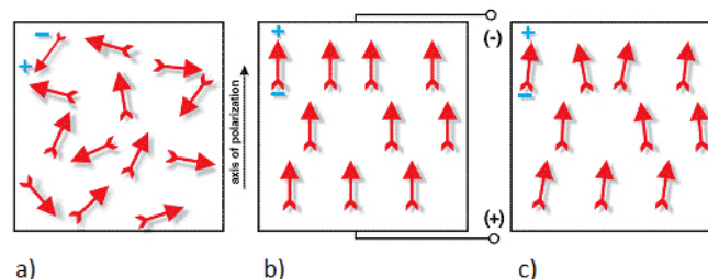
Figure 3.20: Etape de polarisation d'une céramique : a) orientation spontanée des domaines avant polarisation ; b) polarisation en imposant un champ électrique externe ; c) polarisation rémanente [39].
