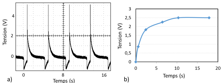
Figure 4.7: Chargement du condensateur 10 µF avec un bilame 122-117°C et un piézoélectrique Murata 220 nF.
