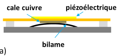
Figure 4.19: Prototypes fonctionnant avec refroidissement par convection naturelle : a) prototype à un bilame et un piézoélectrique, photo en fonctionnement et schéma en section ; b) prototype à deux bilames et deux piézoélectriques, photo en fonctionnement et schéma en section.
