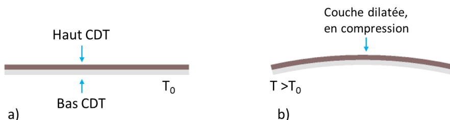
Figure 1.36: Déformation d'un bilame lors du chauffage : a) état initial plat ; b) état courbé quand la température augmente. La couche active (en marron) est à l'extérieur de la courbure.
