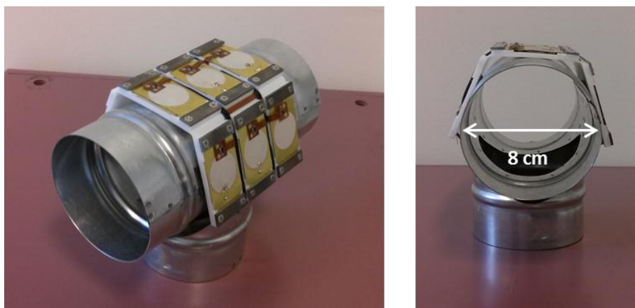
Figure 4.25: Matrice 3x3 avec pistes d'interconnexion flexibles disposée sur un tuyau de 8 cm de diamètre. Vue en perspective et de profil.
