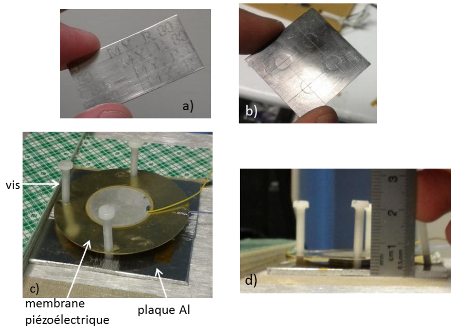
Figure 4.12: a) bilame 43-35 °C ; b) bilame 50-40°C ; c) prototype fin à refroidissement par convection, vue en perspective ; d) vue de profil : épaisseur de 5 mm.
