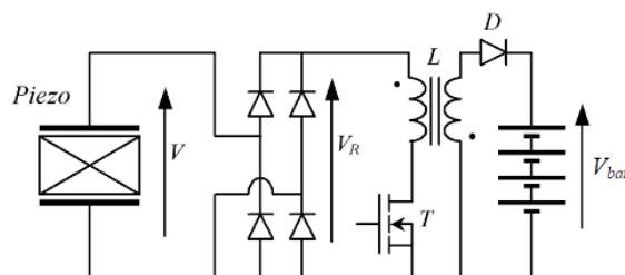
Figure 3.34: Circuit pour la technique SECE. Le piézoélectrique transmet son énergie au transformateur L , commandé par le transistor T [19].
