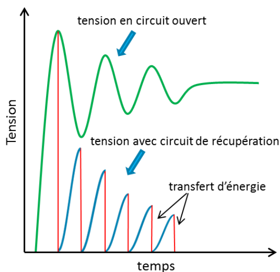
Figure 4.30: Signal en circuit ouvert et avec circuit de gestion de puissance idéal (principe SECE).
