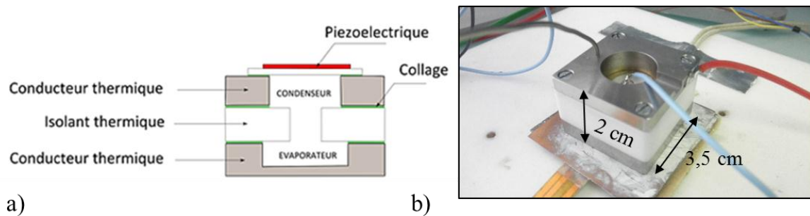
Figure 1.27: Prototype fonctionnant avec des gouttes de liquide : a) schéma montrant la séparation en deux chambres ; b) vue en perspective d'un prototype fabriqué (images offertes par U. Soupremanien/ CEA Liten).
