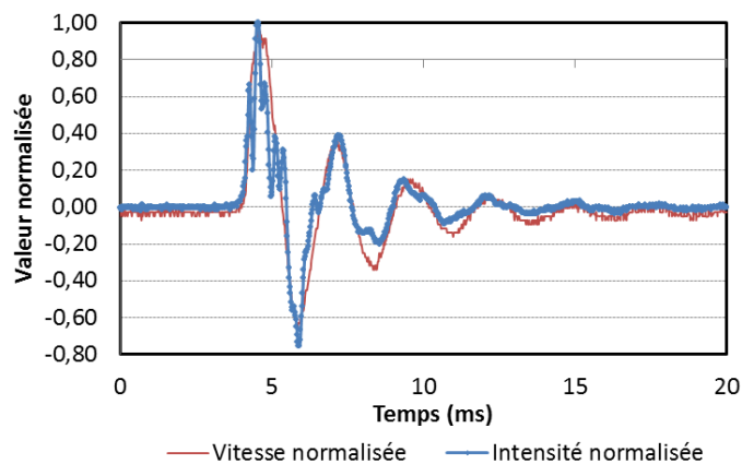
Figure 4.17: Vitesse au centre et intensité normalisées.
