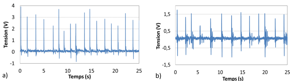
Figure 1.28: Signaux générés par des cellules fonctionnant avec des gouttes d'eau (impédance de mesure de 1 M \Omega ) : a) grande cellule, 3,5 cm de côté ; b) petite cellule 2 cm de côté (données offertes par U. Soupremanien/ CEA Liten).
