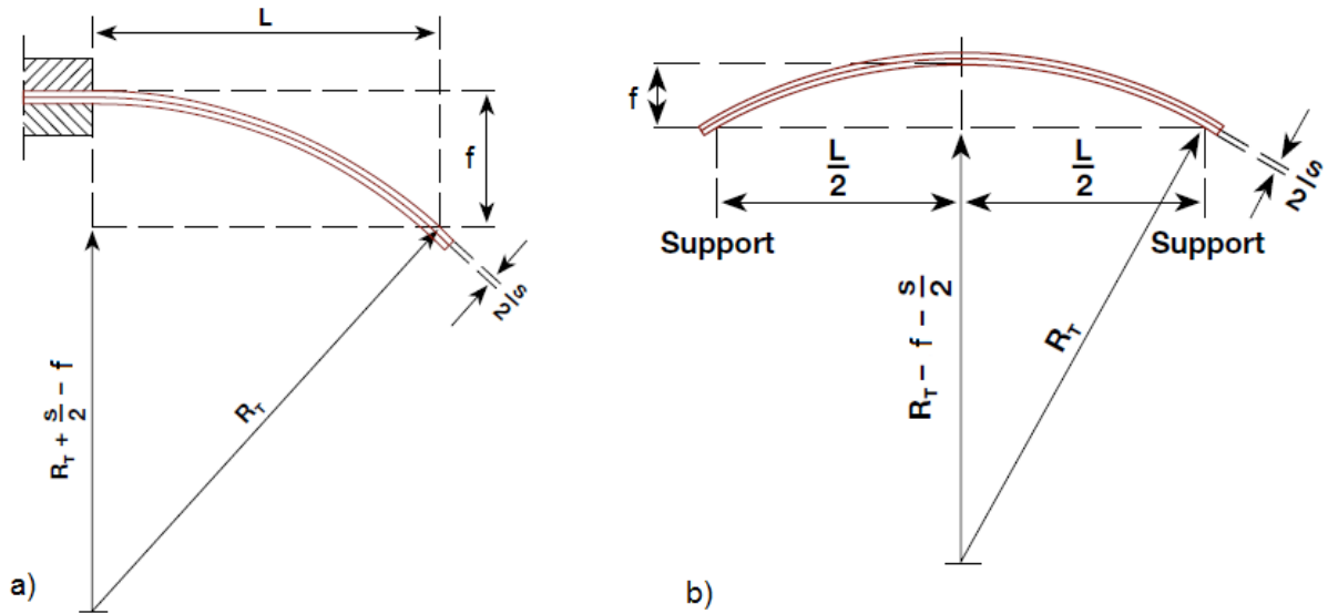
Figure 2.2: Déformation d'un bilame sous forme de poutre soumise à une variation de température :a) bilame encastré d'un côté ; b) bilame libre [30].
