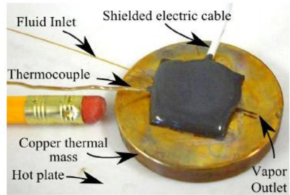
Figure 1.30: Schéma en section et photo d'un prototype à circulation horizontale de fluide. Des gouttes de liquide sont introduites par un tube capillaire et explosent au contact avec le substrat en silicium chauffé [25].
