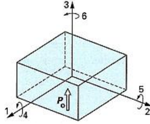
Figure 3.15: Directions pour la notation matricielle [38].
