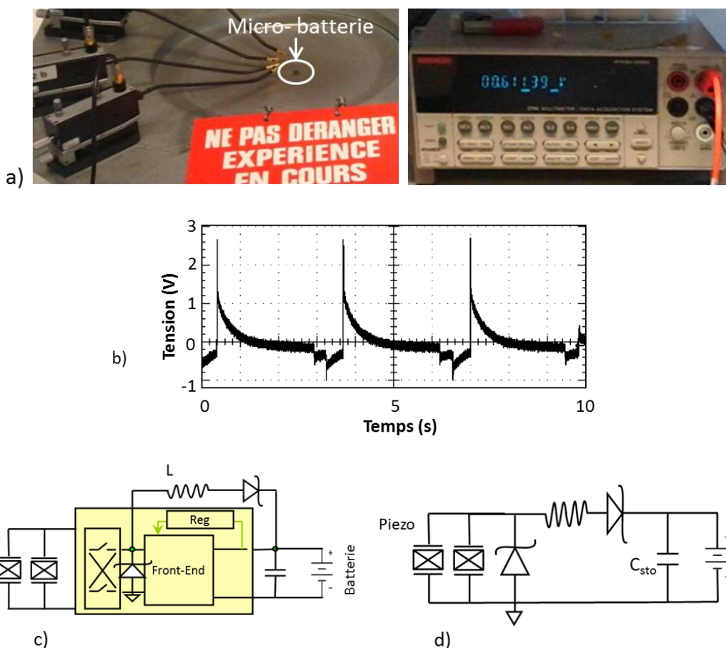
Figure 4.9: a) micro-batterie sous pointes et mesure de sa tension ; b) signal généré par un seul piézoélectrique; c) montage électrique pour chargement jusqu'à 1 V ; d) montage pour chargement au-delà de 1 V.
