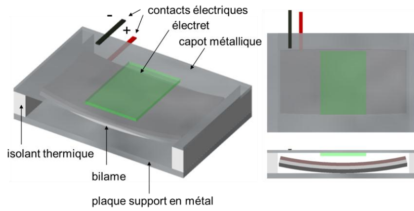
Figure 1.40: Schéma d'un dispositif de récupération d'énergie thermique à base de bilame et électret. Vue en perspective (à gauche) et vue de dessus et de face (à droite).
