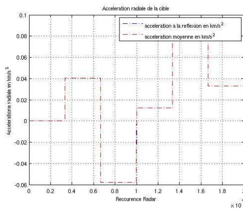
(a) Commandes d'accélération radiale
