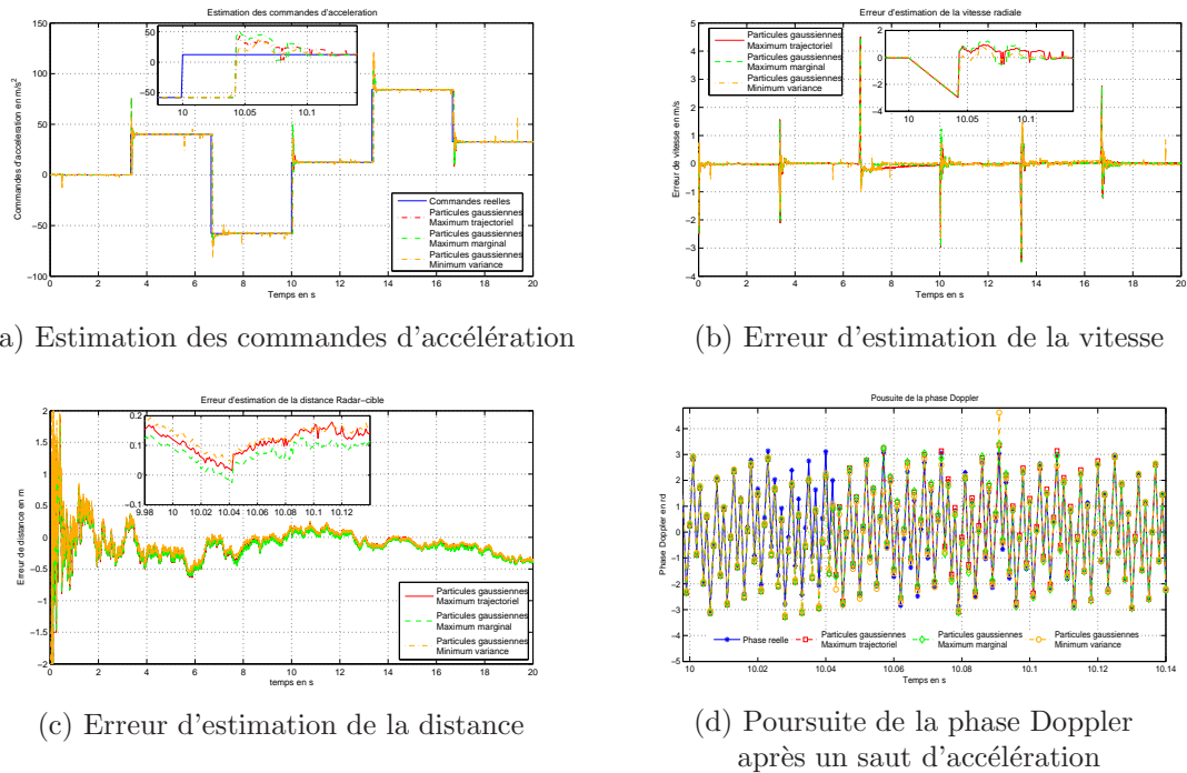
FIG. I.3.4 – Performances de différentes versions du filtre particulaire déterministes dans le traitement des mesures radiales d'un radar de poursuite ( RSB \in [0, 5 \text{ dB}] ).
