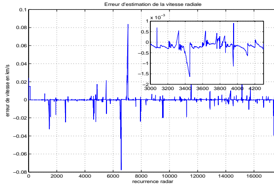
(e) Erreur d'estimation de la vitesse radiale.
