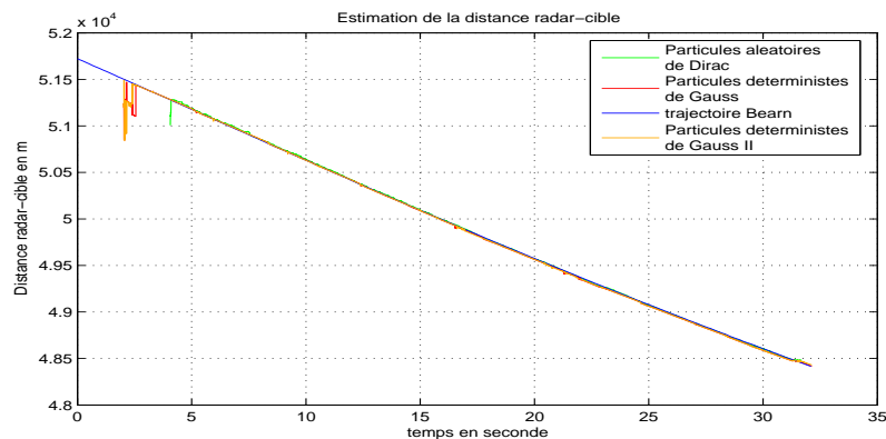
(f) Estimation de la distance radar-cible
