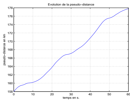
(e) Pseudo-distance récepteur-satellite
