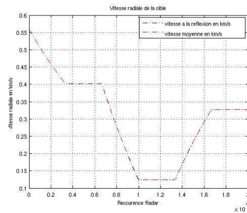
(b) Vitesse radiale
