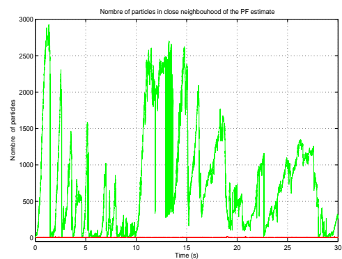
(d) Redondance particulaire autour de la gaussienne la plus massive
