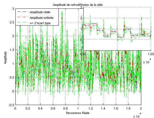
(b) Estimation : Amplitude de la SER
