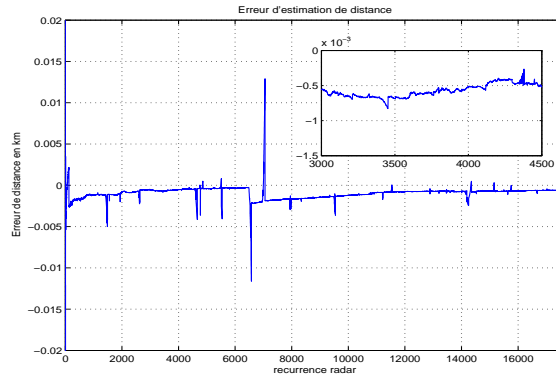
(g) Erreur d'estimation de la distance.
