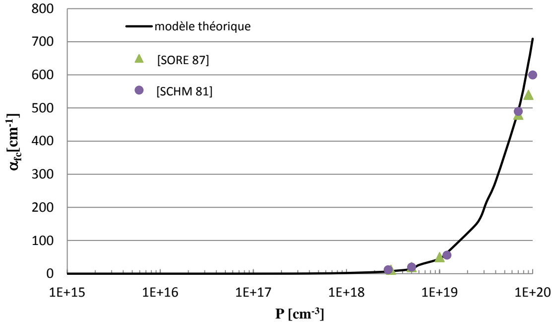
Figure II.3.1.B.2 : Coefficient d'absorption par porteurs libres en fonction de la densité des trous à T=300 K et \lambda=1330 nm.
