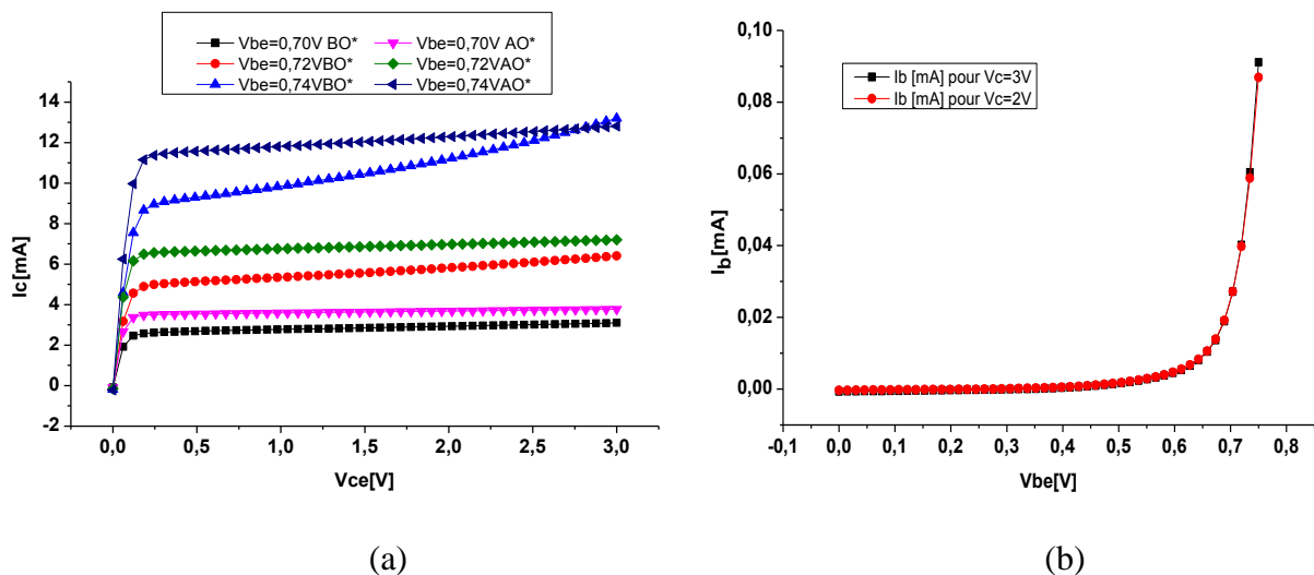
Figure IV.5.2.B.1 : Caractéristique I_C(V_{CE}) du transistor en mode émetteur commun avant (BO) et après (AO) ouverture du composant par la face arrière (a) et caractéristique I_B(V_{BE}) (b)
