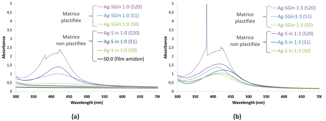
Figure V-8 : Spectres d'absorbances des films élaborés par voie in situ sans plastifiant au cours du stockage à température ambiante (23°C) selon les rapports molaires \text{AgNO}_3 /glucose (a) 1:0 et (b) 1:3. Les films correspondants avec une matrice amidon plastifiée glycérol sont en pointillés.
