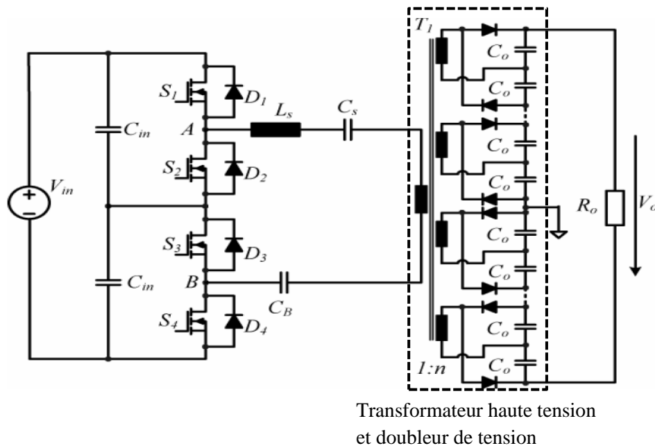
Figure 1-20 Convertisseur résonant série multiniveaux [Wu99]
