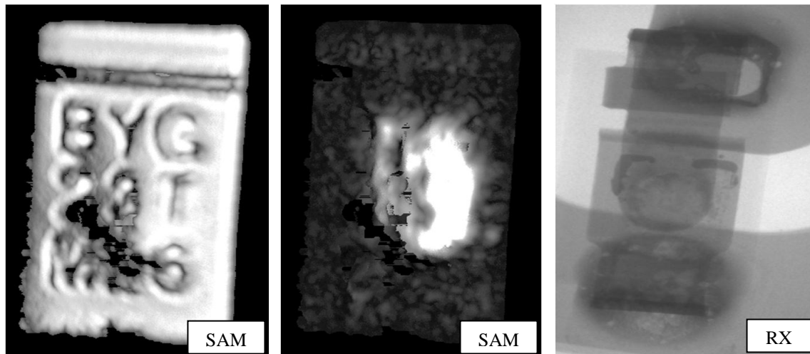
Figure 3-29 Images SAM (à gauche et au milieu) et RX (à droite) de D6
