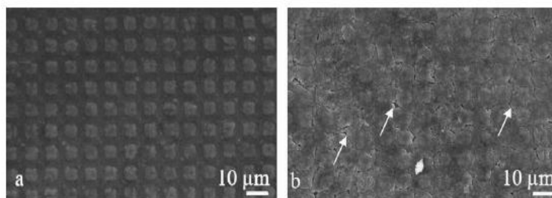
Figure 2-11 Vue au MEB de la métallisation en aluminium avant (a) et après cyclage (b) [Mart09]
