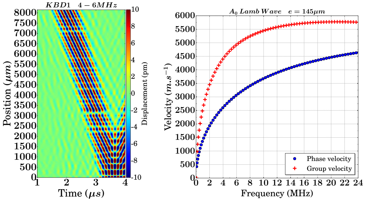
(a) Cartographie le long de la direction de propagation [110]. (b) Vitesses de groupes et de phases des ondes de Lamb A_0 sur plaque e = 145\mu m selon la direction [100] (simulation).
