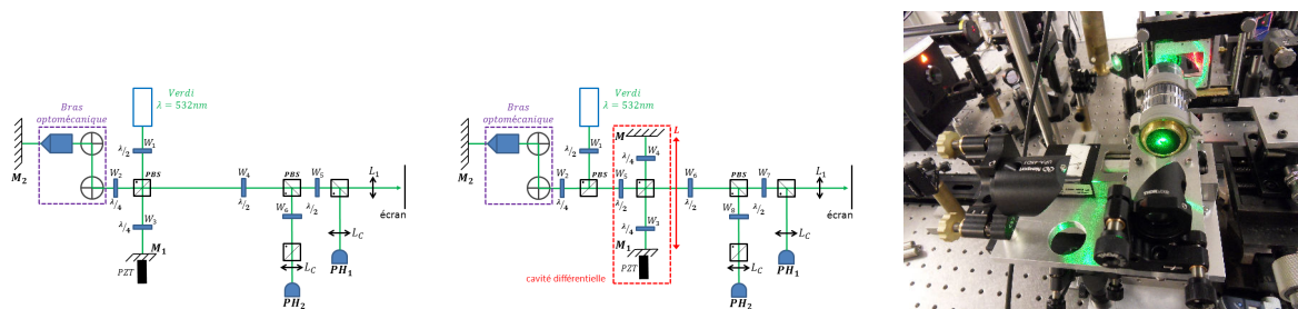
(a) Schéma optique de l'interféromètre de Michelson utilisé pour la mesure de comparaison 2.22. Cette configuration permet de passer très rapidement à celle du montage différentiel.
