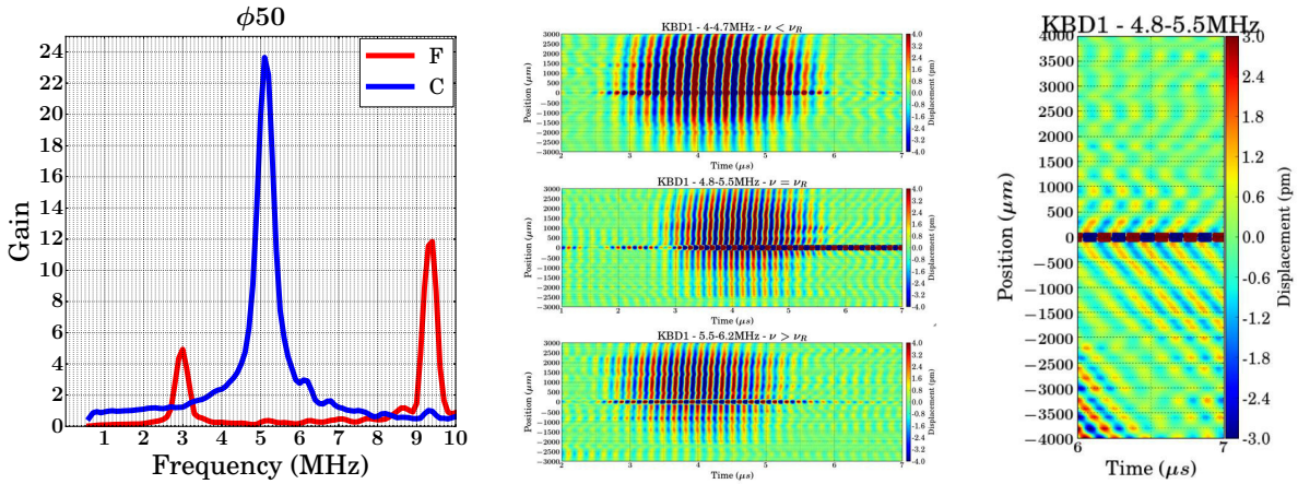
(a) Gains GF et GC du pilier de diamètre \phi 50 . Les modes F_1 et C_0 de fréquences propres respectives \nu \approx 3MHz et \nu \approx 5MHz sont bien séparés.
