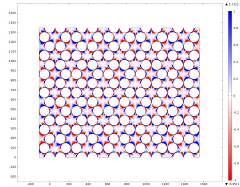
FIGURE 4.12 – Simulation mode propre de vibration du cristal phononique à 20.1MHz correspondant à un mode optique en bord de gap.
