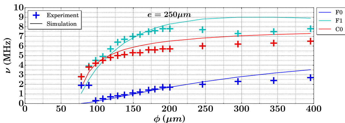
(c) Comparaison des mesures expérimentales des fréquences propres en fonction du diamètre des piliers ( h = 240\mu\text{m} ) du wafer e = 250\mu\text{m} (carrés) aux valeurs simulées des fréquences propres d'un cône d'angle 9^\circ et de hauteur h = 240\mu\text{m} (trait plein).
