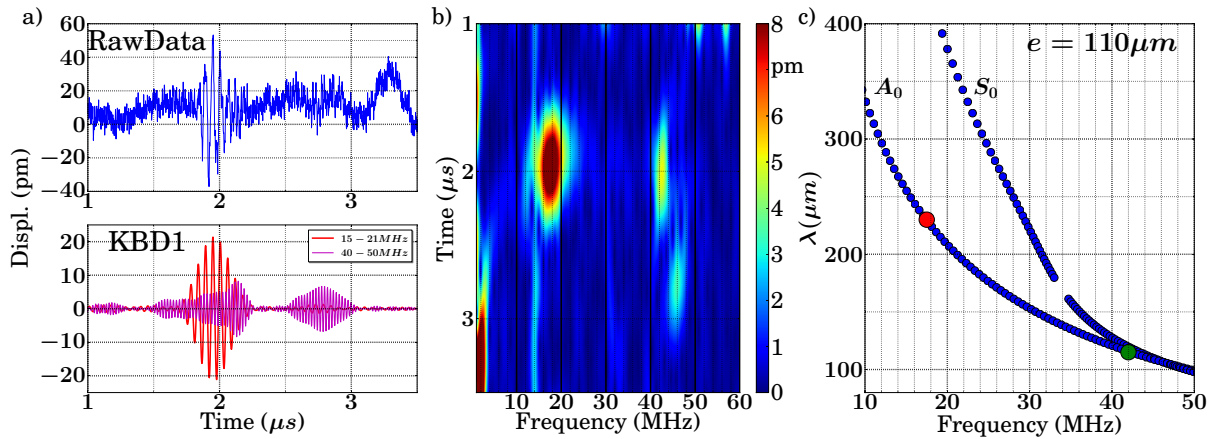
FIGURE 3.19 – Données obtenues par la technique de génération par imagerie d'un masque sur wafer d'épaisseur e = 110\mu\text{m} . a) Signaux expérimentaux du déplacement de surface respectivement « brut » et filtré. b) Spectrogramme du signal calculé à l'aide d'une fenêtre de filtrage gaussienne de largeur à mi-hauteur fixe égale à 1.5\text{MHz} . c) Longueur d'onde théorique en fonction de la fréquence pour une plaque de silicium d'épaisseur e = 110\mu\text{m} . Le mode fondamental ( 17.5\text{MHz} ) ainsi que l'harmonique symétrique ( 46\text{MHz} ) et l'harmonique antisymétrique ( 42\text{MHz} ) sont générés.
