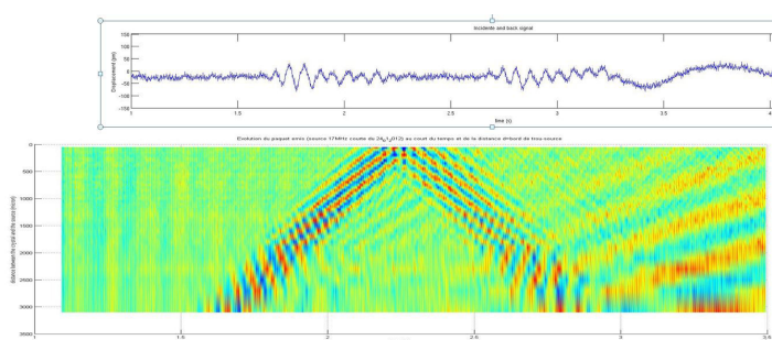
(a) Evolution spatio-temporelle du déplacement sans post-traitement le long de la ligne n^01 . La figure du haut correspond à l'évolution temporelle du déplacement en un point tel que x \approx 1000\mu m .
