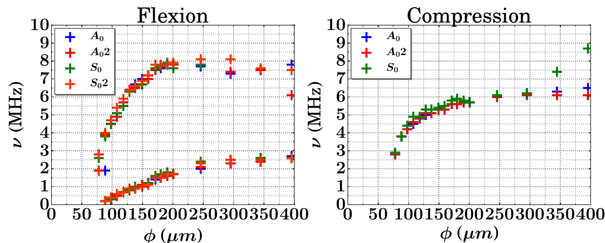
FIGURE 5.21 – Fréquences propres expérimentales de flexion et de compression des systèmes pilier sur plaque en fonction de \phi , pour une épaisseur du wafer de e = 250\mu m , et en fonction de la nature du mode excitant le pilier ( A_0 ou S_0 ). Les résultats sont affichés pour deux méthodes différentes de calcul (identifiées par l'indice 2 dans la légende).
