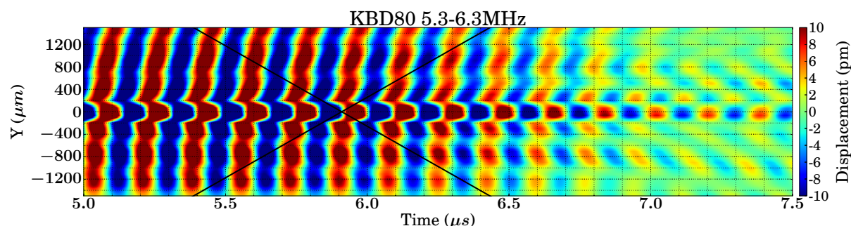
FIGURE 5.47 – Rayonnement polaire du mode C_0 à résonance, sous incidence A_0 . Les deux traits sont de pente égale à la vitesse de phase à \nu = 5.8\text{MHz} , selon la direction [100] ( V_\phi^{A_0} = 2870\text{m.s}^{-1} ). Le fort rayonnement est en quadrature par rapport au sommet du pilier.
