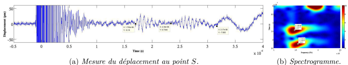
FIGURE 4.14 – Mesure du déplacement absolu au point S et spectrogramme associé. La source est un paquet d'ondes centré à \nu_0 \approx 15 MHz et le signal réfléchi est filtré en fréquence par le cristal (effet « bandgap »).
