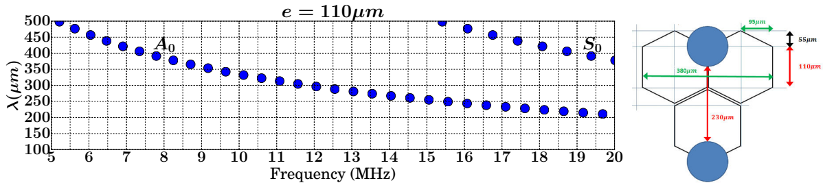
FIGURE 4.6 – Longueur d'onde des modes de Lamb A_0 selon la direction [100] pour une plaque d'épaisseur e = 110\mu m et schéma des grandeurs caractéristiques de la cavité.
