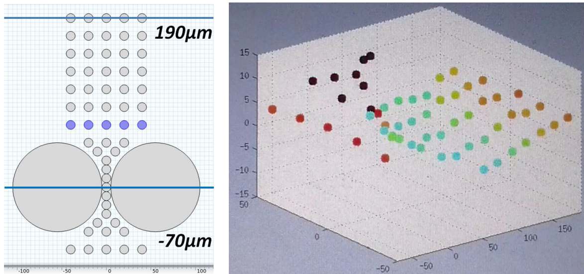
(a) Positions des points de mesures de la cartographie du champ de diffusion autour de la paire de trous i = 11\mu\text{m} .
