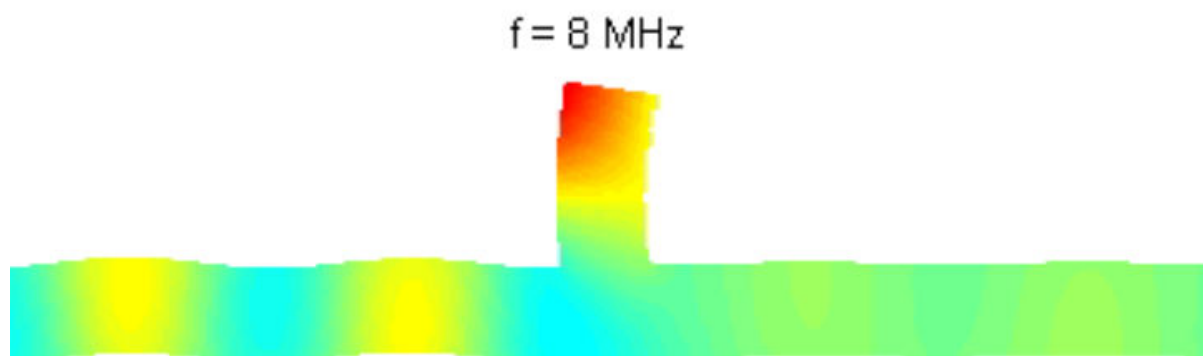
FIGURE 5.65 – Simulation du déplacement d'un pilier d'une ligne infinie à la fréquence de 8 MHz. Le pilier présente ce mouvement important du côté de l'onde incidente et un quasi zéro de déplacement partout sur l'arrière du pilier. Une léger fuite est visible. Cliquez sur l'image !
