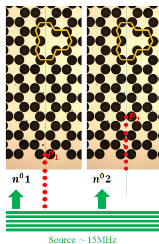
FIGURE 4.7 – Schéma de la configuration expérimentale des expériences n^01 et n^02
