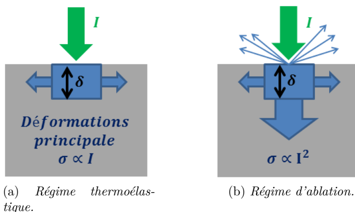
FIGURE 3.2 – Illustrations des deux régimes d'absorption lors de la génération d'une onde de type Lamb ou Rayleigh sur le silicium.
