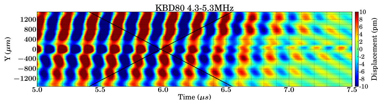
FIGURE 5.46 – Rayonnement polaire avant résonance \nu_{C_0} sous incidence A_0 . Les deux traits sont de pente égale à la vitesse de phase à \nu = 4.8\text{MHz} , selon la direction [100] ( V_\phi^{A_0} = 2650\text{m.s}^{-1} ), et permettent de constater que le faible rayonnement est en quadrature de phase avec le sommet du pilier.
