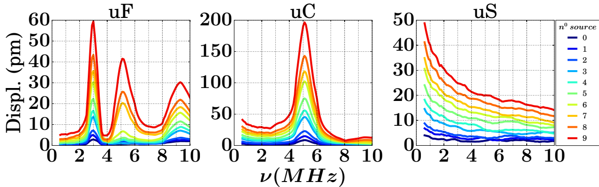
FIGURE 5.27 – Déplacements en flexion uF = \frac{u_A(\nu) - u_B(\nu)}{2} et en compression uC = \frac{u_A(\nu) + u_B(\nu)}{2} du pilier \phi = 49 \pm 1\mu m, h = 245 \pm 13\mu m, e = 175 \pm 5\mu m , ainsi que le déplacement uS de la source A_0 , en fonction des différentes puissances de sources utilisées, numérotées par ordre croissant de puissance de 0 à 9.
