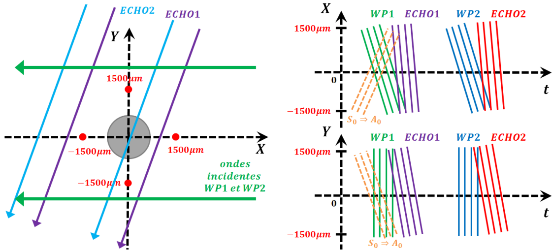
(a) Représentation schématisée de la position des faisceaux incidents WP1 et WP2 et des échos ECHO1 et ECHO2 sur le pilier.
