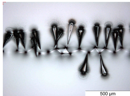
(b) « Fossiles » d'une ligne de piliers de diamètre inférieur à \phi_{limite} . La forme en cône d'angle 9^\circ peut laisser penser que toutes les gravures ont subi cette anomalie de verticalité.
