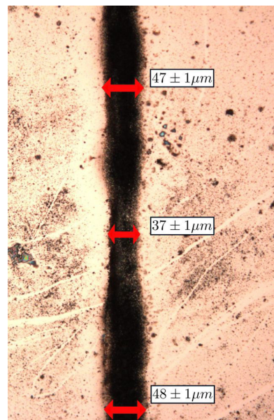
FIGURE 3.12 – Image microscope optique \times 20 du résultat de l'ablation d'un wafer de silicium ( e = 145 \pm 3\mu\text{m} ) par une ligne source focalisée à l'aide d'une lentille cylindrique de focale f' = 300\text{mm} .
