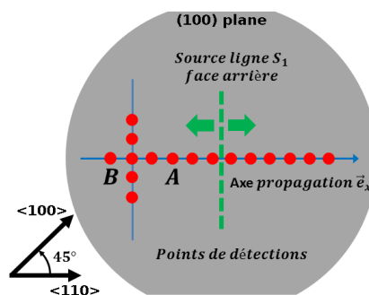
(b) Schéma du wafer et des points de détection pour l'étude de la génération ligne sur une plaque de silicium d'épaisseur 145 \pm 3\mu m (source S_1 ).
