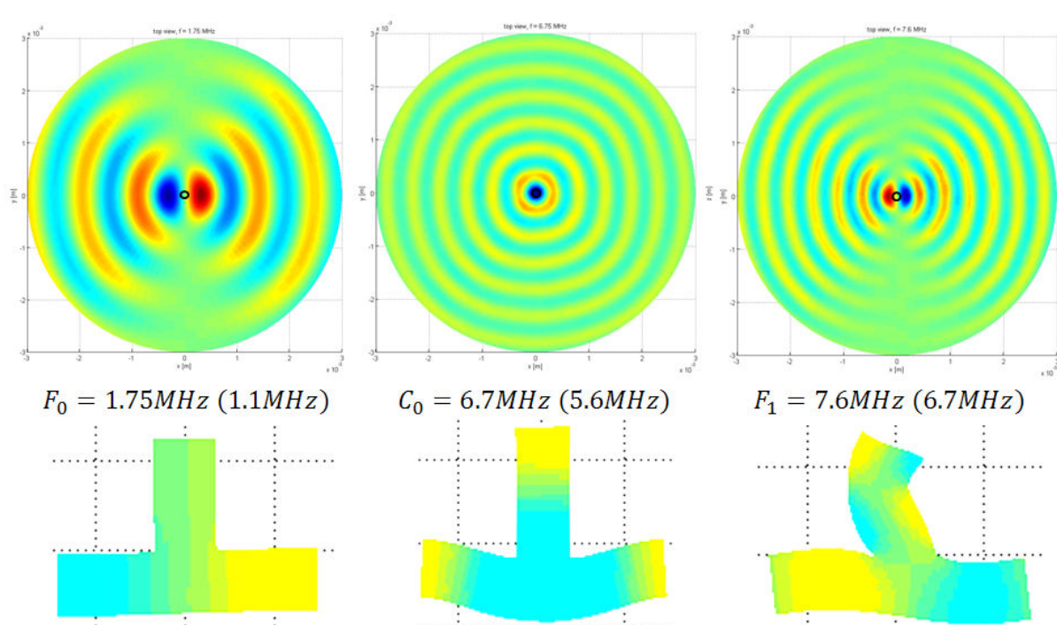
FIGURE 5.30 – Simulations des trois ondes réémises par la pilier \phi 150 par application d'une force surfacique au sommet du pilier purement longitudinale dans le cas des modes de flexion, et purement transversale dans le cas du mode de compression. La fréquence calculée est indiquée ainsi qu'entre parenthèse la fréquence mesurée expérimentalement pour un pilier avec e = 175 \pm 5\mu m / \phi = 150 \pm 2\mu m / h = 245 \pm 13\mu m (simulations réalisées par Fabrice Lemoult).
