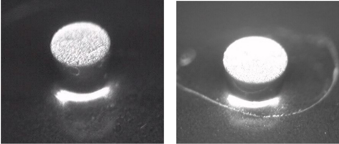
(a) Pilier isolé Si/Si avec \phi = 146 \pm 2\mu\text{m} , h = 240 \pm 10 , e = 125 \pm 5\mu\text{m} . (b) Pilier isolé tel que \phi = 293 \pm 6\mu\text{m} , h = 243 \pm 10 , e = 125 \pm 5\mu\text{m} .
