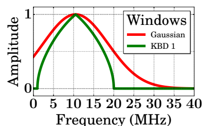
FIGURE 3.5 – Fenêtre gaussienne et KBD1 utilisées pour le filtrage de la figure 3.6
