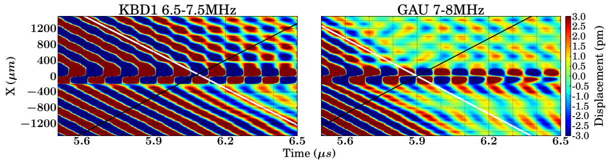
FIGURE 5.48 – Spatio-temporels à résonance ( 6.5 - 7.5\text{MHz} ) et après résonance ( 7 - 8\text{MHz} ) de flexion F_1 . Les droites tracées (toujours de pente égale à la vitesse de phase théorique) permettent de suivre le front d'onde des ondettes rayonnées, afin d'établir les relations de phases entre l'onde incidente, l'onde réémise et le sommet du pilier.
