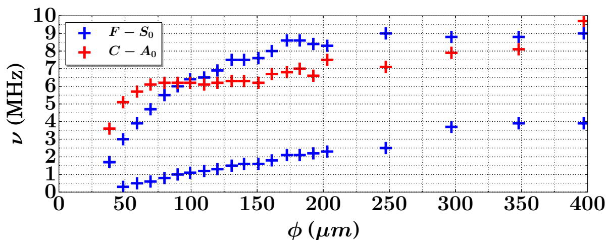
FIGURE 5.19 – Fréquences propres expérimentales d'un système pilier sur plaque en fonction de \phi sachant h = 250 \pm 15\mu\text{m} et e = 175 \pm 5\mu\text{m} .
