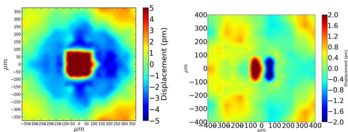
(a) Cartographie du champ diffusé à résonance de C_0 pour le pilier \phi 150 .
