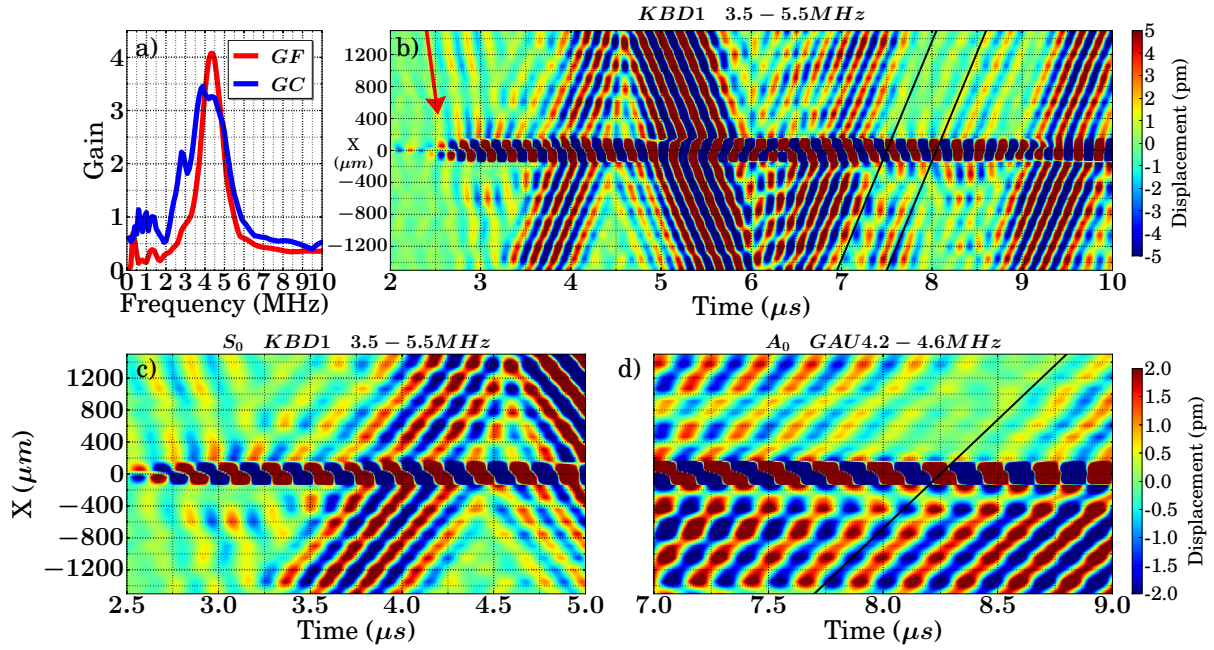
FIGURE 5.55 – a) Gains en flexion et en compression du pilier \phi 100 . Les fréquences des deux modes propres sont identiques, égales à \approx 4.5\text{MHz} . Les valeurs des gains sont semblables, égales à \approx 4 . b) Cartographie le long de X filtrée à l'aide d'une fenêtre KBD1 , entre 3.5 - 5.5\text{MHz} . La base de temps permet de voir arriver le signal de type S_0 , puis la formation de son écho de type A_0 , qui revient sur le pilier. c) et d) Agrandissement des zones de mélange d'ondelettes émises sous l'effet du paquet d'ondes S_0 et A_0 . La figure d) correspond au comportement attendu d'une cellule élémentaire métamatériaux pouvant être décrite simultanément par une masse et une compressibilité effectives négatives.
