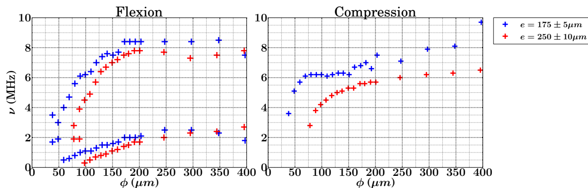
FIGURE 5.22 – Fréquences propres expérimentales d'un système pilier sur plaque en fonction de \phi , pour deux valeurs d'épaisseur du wafer e = 175\mu\text{m} et e = 250\mu\text{m} , sachant h = 250 \pm 15\mu\text{m} supposée constante pour tous les piliers.
