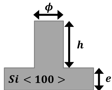
FIGURE 5.8 – Notation des paramètres du système \{\text{Pilier Si/Si}\}
