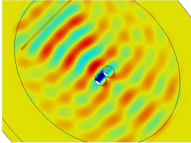
FIGURE 4.22 – Simulation numérique de la diffusion résonante d'une onde de Lamb A_0 de fréquence centrale 15MHz ( \lambda \sim 250\mu m ) sur une paire de trous i = 10\mu m fabriquée dans une plaque de silicium d'épaisseur 110\mu m .
