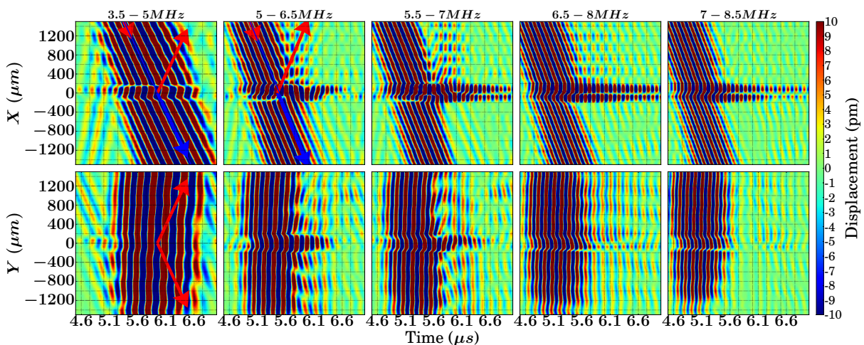
FIGURE 5.45 – Spatio-temporels du déplacement filtré à l'aide d'une fenêtre gaussienne de largeur à mi-hauteur indiquée en colonne. On peut y voir les rayonnements polaires et dipolaires associés respectivement aux modes C_0 et F_1 .
