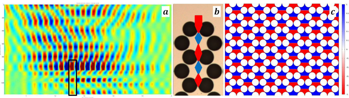
FIGURE 4.9 – Ensembles de données concernant le comportement des ondes autour du bas du bandgap du cristal phononique. a) Mesure expérimentale à l'interface silicium-cristal. L'onde arrive du haut de l'image. On identifie une onde réfléchi. La structure du déplacement dans le cristal est matérialisée par le rectangle noir. b) Schéma des ventres et des nœuds de déplacement mesurés sur la figure a). La figure c) est une simulation numérique des modes propres d'un cristal infini à 12.8MHz .
