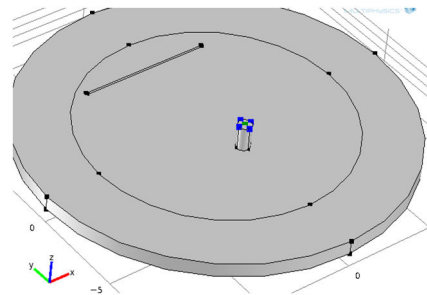
FIGURE 5.9 – Système simulé pour l'étude de la diffusion d'une onde de Lamb sur un pilier isolé Si/Si .
