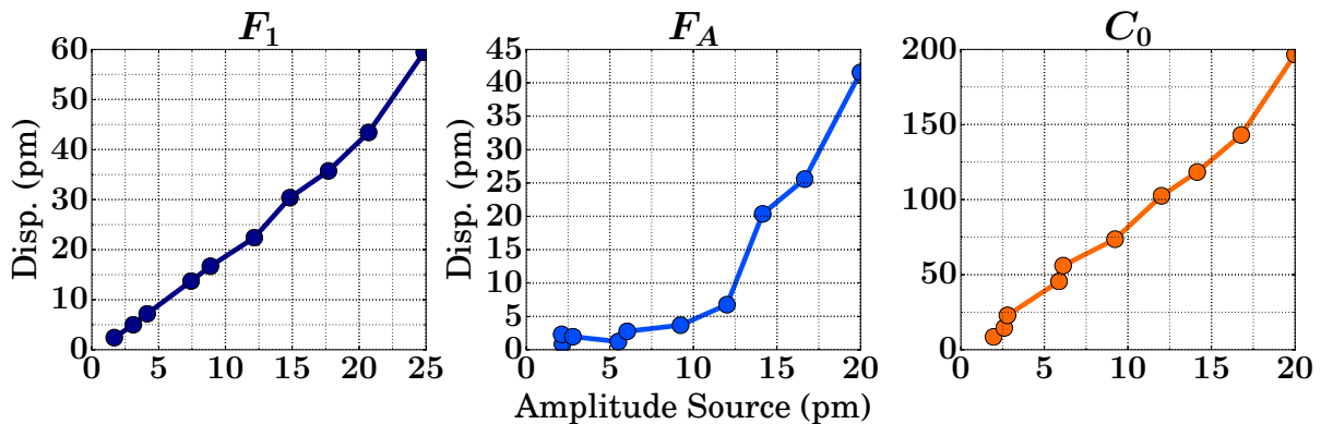
FIGURE 5.28 – Amplitudes des déplacements associées aux modes F_1 , C_0 , et F_A du pilier \phi = 49 \pm 1\mu m, h = 245 \pm 13\mu m, e = 175 \pm 5\mu m , en fonction de l'amplitude absolue de la source. Les tendances sont toutes linéaires avec l'amplitude de la source pour F_1 et C_0 . Le mode de flambage présente une énergie d'activation ( u_S > 10pm ).
