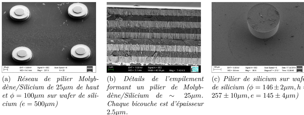
FIGURE 1.12 – Images MEB des deux types de structures piliers gravées par DRIE « Bosh Profond » sur substrat de silicium.
