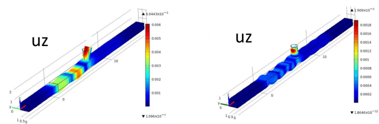
(d) Modes de vibration du pilier d'une ligne à la fréquence de \sim 2\text{MHz} (à gauche) et à la fréquence de \sim 8\text{MHz} (à droite). Ces vibrations correspondent aux mouvements des piliers au niveau des zéros de transmission.
