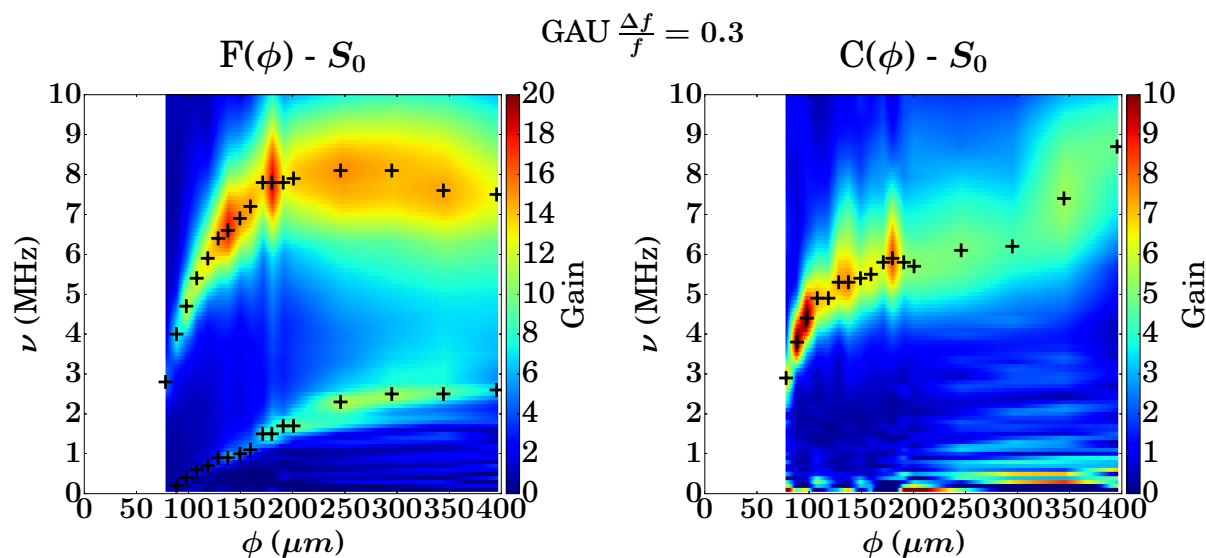
FIGURE 5.20 – Gains en flexion GF et en compression GC en fonction du diamètre des piliers sur plaque d'épaisseur e = 250 \pm 10\mu m .
