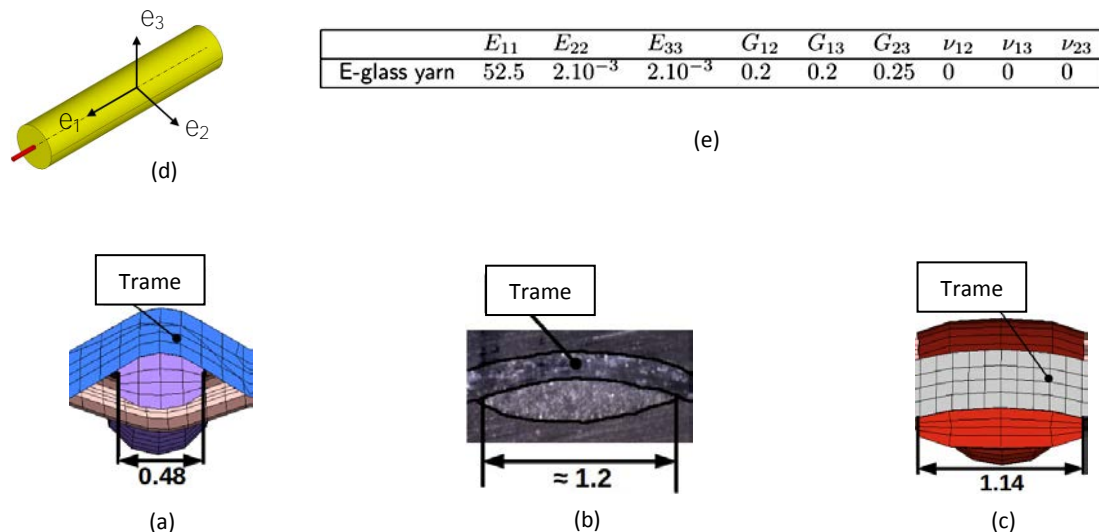
Figure 6-10. Effet du coefficient de poisson \nu_{23} sur l'écrasement du fil (longueur en mm) : (a) plan de coupe orthogonal à la direction du fil de chaîne, (b) échantillon de fil résiné (valeur moyenne), (c) plan de coupe orthogonal à la direction du fil de chaîne avec \nu_{23}=0.9 ; (d) repère matériau lié aux fils ; (e) paramètres élastiques de la loi de comportement isotrope transverse (unité de pression : GPa).
