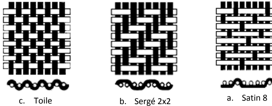
Figure 1-5. Les trois armures fondamentales du tissage [171].
