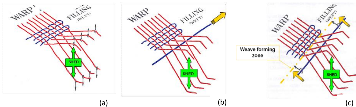
Figure 2-2. Etapes de la formation d'un tissu ; (a) ouverture de la foule ; (b) insertion du fil de trame ; (c) tassage du fil de trame.
