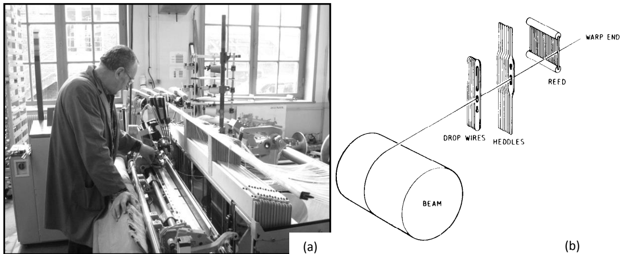
Figure 2-10. (a) Rentrage et piquage simultanés des fils de verre chaîne respectivement dans les lisses et le peigne ; (b) Eléments intervenants sur le fil de chaîne entre l'ensouple et le tissu.
