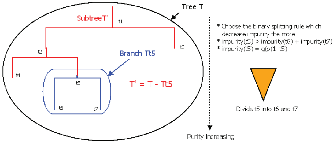
FIGURE B.2 – Construction d'un arbre binaire
