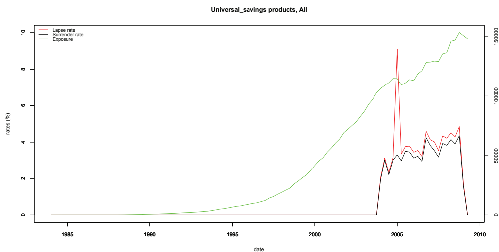
FIGURE C.21 – Exposition et taux de rachat trimestriel du portefeuille, Universal Savings.
