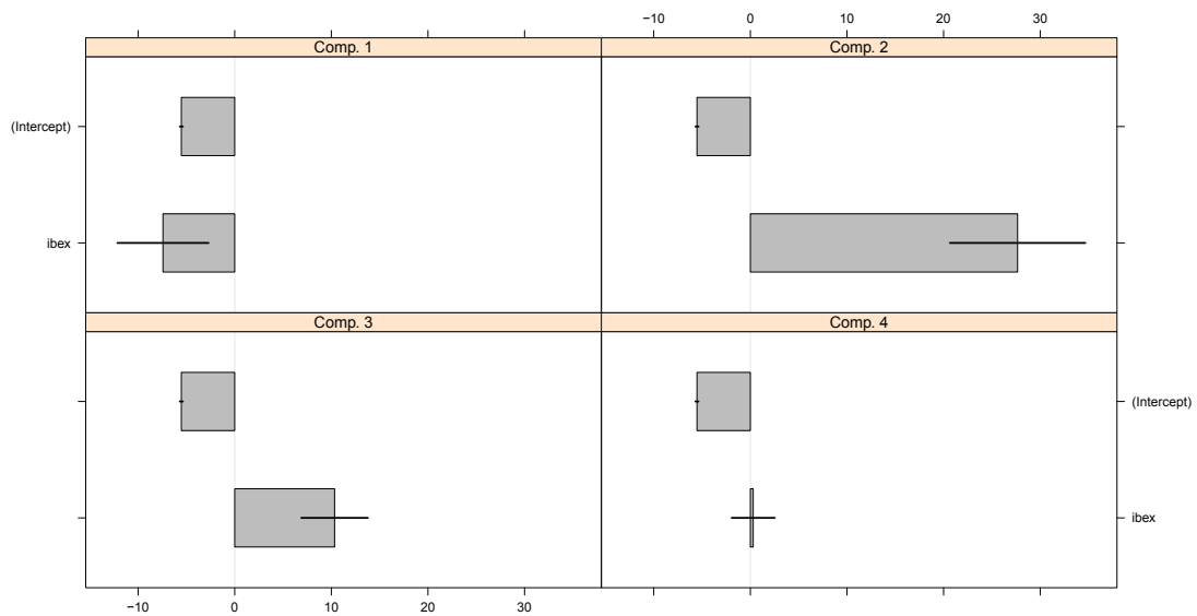
FIGURE C.36 – Coefficients de régression des composantes, produits structurés.
