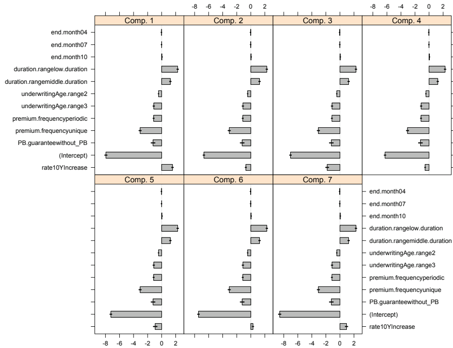
FIGURE 4.7 – Calibrage des coefficients de régression par BIC.
