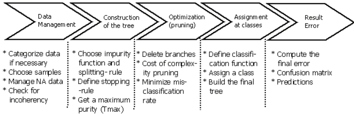
FIGURE B.1 – Etapes chronologiques de la procédure CART
