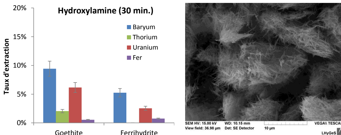
Figure IV-15 : A) Extraction à l'hydroxylamine de goethite et de ferrihydrite à 4mg/ml d'oxydes par ml d'extractant. B) Image MEB de goethite après attaque à l'hydroxylamine (voir goethite initiale Figure IV-7.A).
