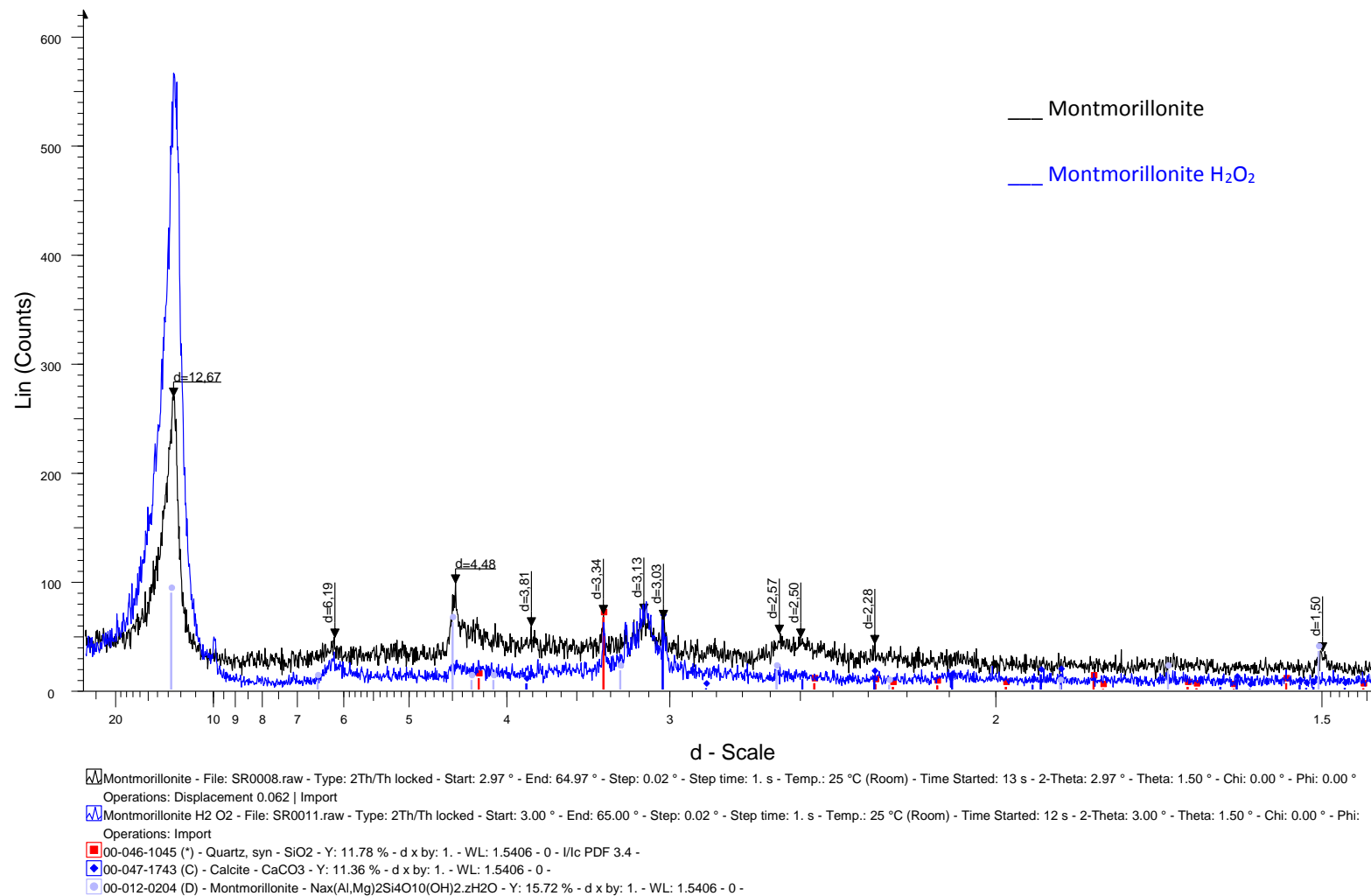
Figure A2-7 : Diffractogramme RX de la montmorillonite avant et après traitement à l'eau oxygénée.
