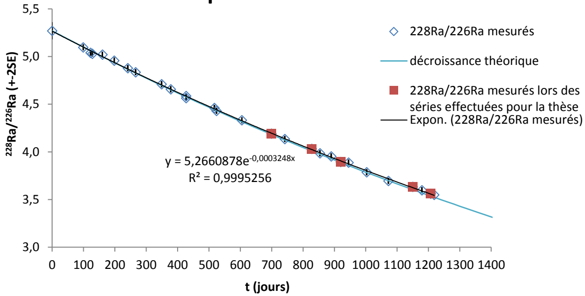
Figure A1-7 : Evolution du rapport ( ^{228}\text{Ra}/^{226}\text{Ra} ) du spike en fonction du temps. La taille des points correspond à la barre d'erreur.
