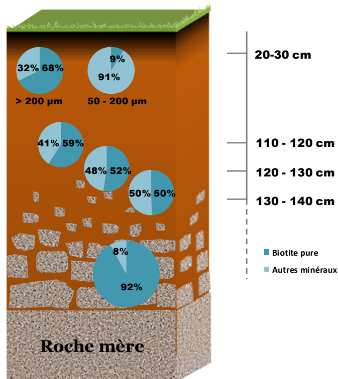
Figure V-2 : Récapitulatif des habitus de biotites issues du bloc 1 du site de Breuil avec les compositions en biotites pour chaque habitus.
