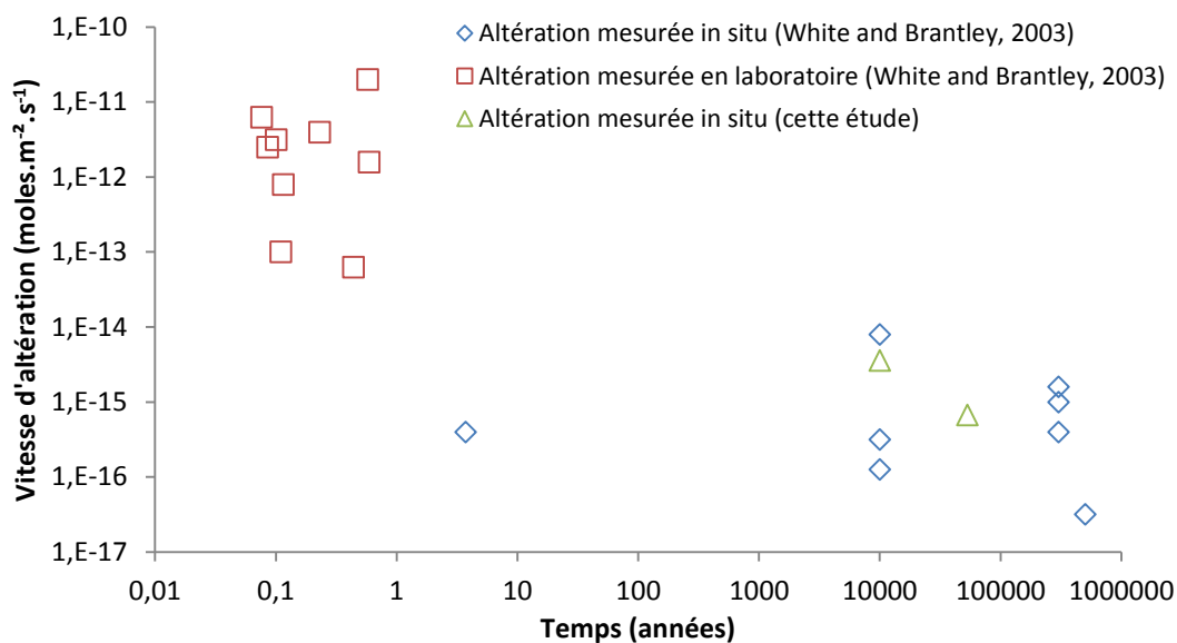
Figure V-14 : Vitesses d'altération calculées et comparées aux données de la littérature. Adapté de (White et Brantley, 2003).
