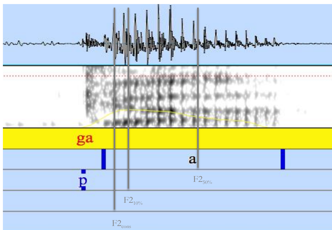
Figure 19 : Exemple schématisé des trois valeurs formantiques prises le long du F2 : au début de la voyelle ( F2_{cons.} ), à 10% ( F2_{10\%} ) et à 50% ( F2_{50\%} ).
