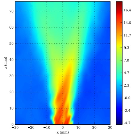
(d) LES - \widetilde{U}_z [m.s -1 ] - Plane Y = 4 mm
