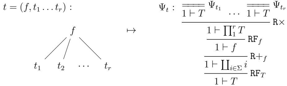
Figure 7.2 Représentation des \Sigma -arbres en preuves
