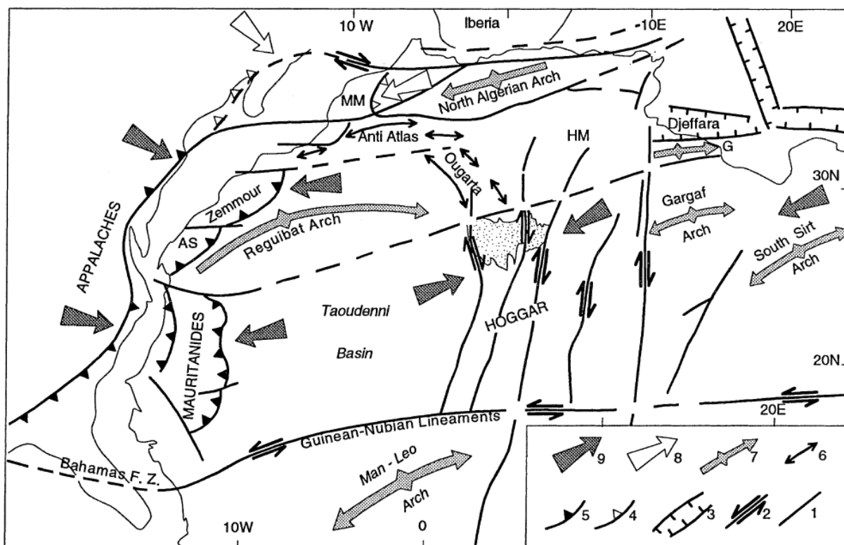
Figure II-6: Déformation intraplaque de la plateforme saharienne pendant les événements varisques, pour le Carbonifère, et le Permien. 1. Faille majeure ; 2. Faille décrochante majeure ; 3. Zone de rift ; 4. Zone de chevauchements majeure d'âge carbonifère supérieur ; 5. Zone de chevauchements majeure d'âge permien inférieur ; 6. Chaînes plissées d'avant-pays Carbonifère supérieur et Permien inférieur ; 7. Soulèvement d'« arches » ou bombements de socle ; 8. Direction de raccourcissement carbonifère supérieur ; 9. Direction de raccourcissement permien inférieur ; AS : Adrar Soutouf ; G : Gaharien Arch ; HM : Hassi Messaoud ; IB : Illizi Basin ; MM : Moroccan Meseta. D'après Haddoum et al. (2001).
