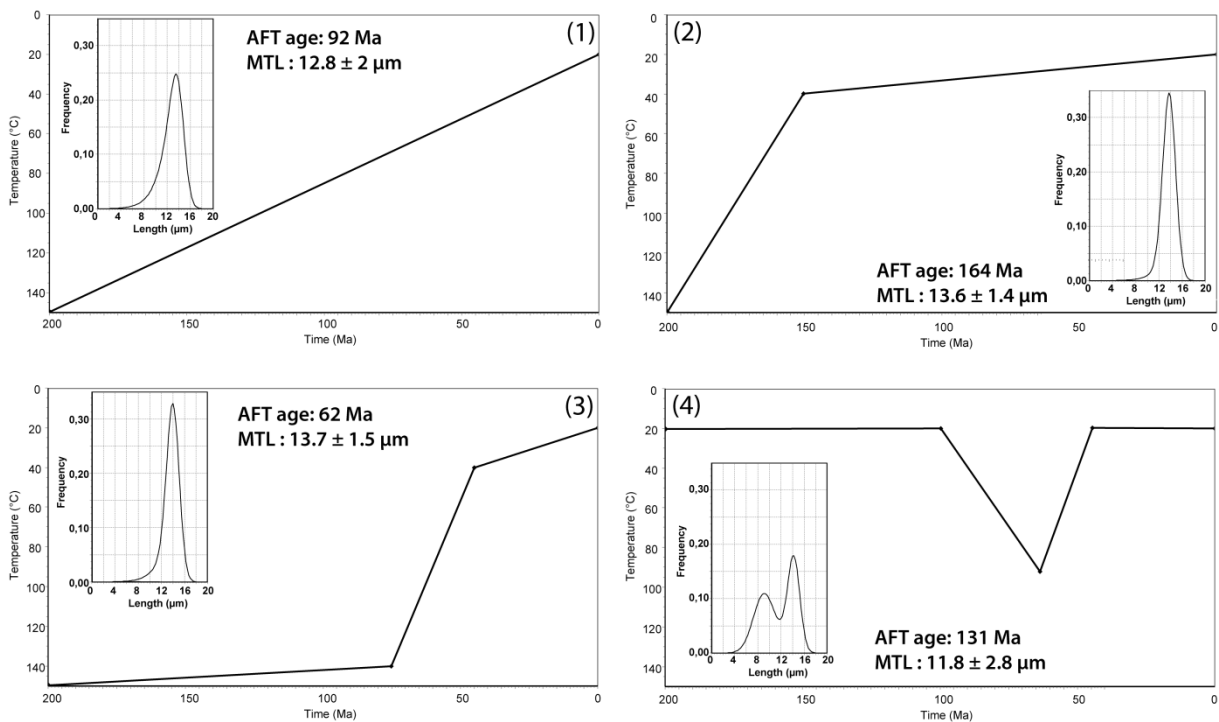
Figure III-3 : Modélisations d'histoires thermiques types avec HeFTy (Ketcham et al., 2005) et prédictions associées (âge AFT, moyenne des longueurs, distribution des longueurs). Pour les deux cas de refroidissement rapide (2) et (3), les distributions des longueurs de traces sont similaires et seuls les âges AFT permettent de les distinguer. La modélisation (1) montre qu'un refroidissement lent « étale » la distribution des longueurs vers les longueurs courtes, ceci étant dû au séjour prolongé dans la ZCP. Enfin, un événement de réchauffement (4) provoquera la cicatrisation partielle d'une partie des traces de fission déjà existantes, générant un pic de distribution autour de 8-9 µm tandis que le retour aux conditions "froides" de surface génère à nouveau un pic d'abondance en traces à 13-14 µm. D'autre part, cet événement rajeunit fortement l'âge AFT.
