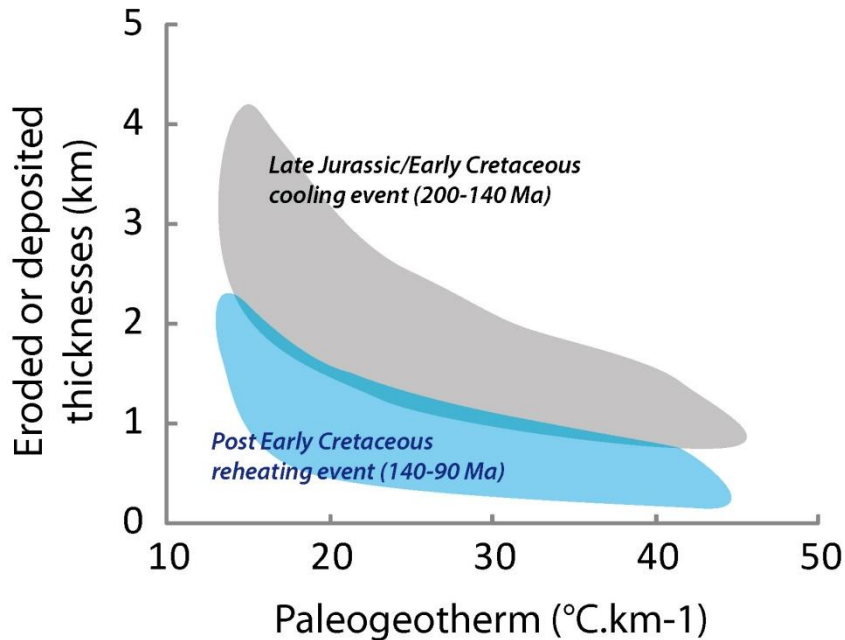
Figure IV-27. Estimations des épaisseurs déposées/érodées en fonction du paléogéotherme. En gris, la surface présente les estimations d'épaisseurs érodées pendant l'événement de refroidissement Jurassique supérieur/Crétacé inférieur. En bleu, la surface présente les estimations d'épaisseurs déposées pendant l'événement de réchauffement qui suit les conditions de subsurface au début du Crétacé inférieur.
