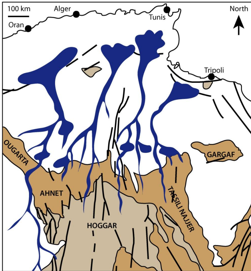
Figure II-8 : Interprétation paléogéographique des dépôts du Continental Intercalaire dans la partie centrale du Sahara pendant le Barrémien-Albien (d'après Lefranc et Guiraud, 1990). Gris : socle ; Marron : Paléozoïque ; Blanc : post-Paléoz.
