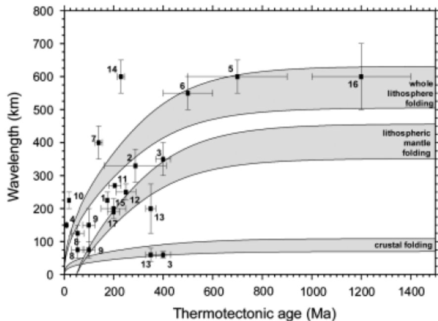
Figure VI-22: Estimations des longueurs d'ondes des plissements suivant l'âge thermotectonique de la lithosphère (de Cloetingh and Burov, 2011). Les nombres indiquent les différents contextes géologiques étudiés pour estimer ces longueurs d'ondes (figure 3 dans l'étude de Cloetingh and Burov (2011)).
