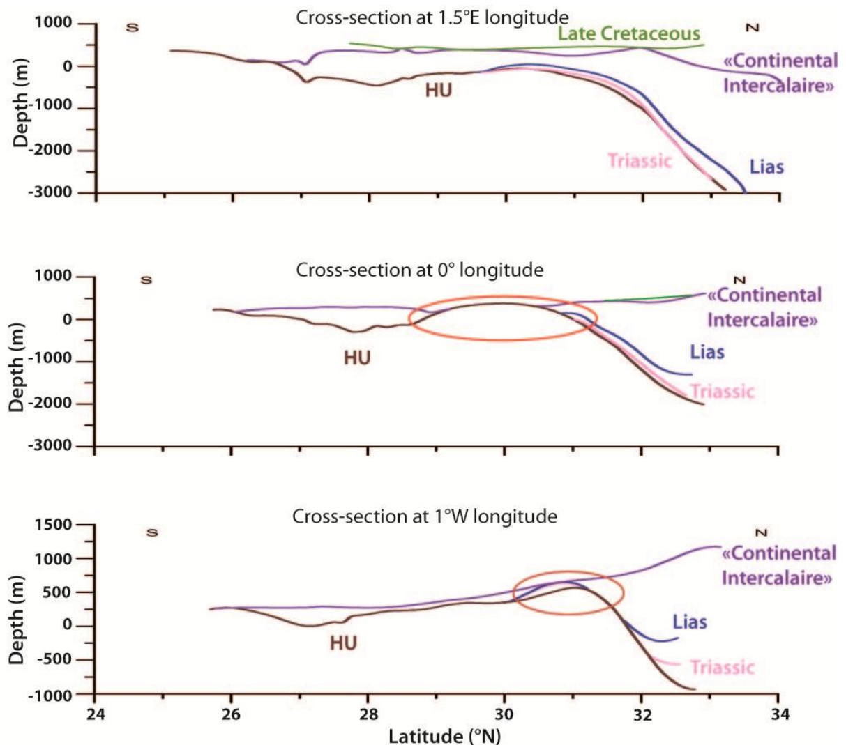
Figure VI-4 : Coupes Nord-Sud dans la plateforme saharienne (localisées sur la fig. VI-3). Tous les traits de couleur indiquent le sommet de la formation. HU : Discordance Hercynienne. Les cercles rouges soulignent les arches de socle.
