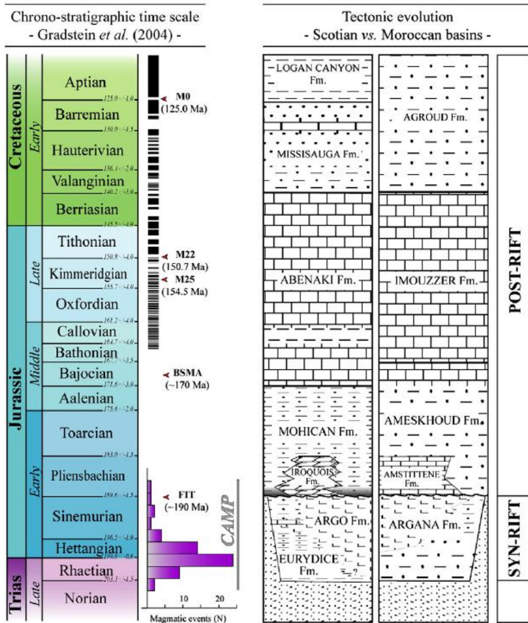
Figure VI-10 : Synthèse des données stratigraphiques dans les bassins conjugués de Nouvelle-Ecosse et du Nord du Maroc (d'après Labails et al. , 2010). On remarque les grandes similitudes partagées par ces deux régions jusqu'au Crétacé.
