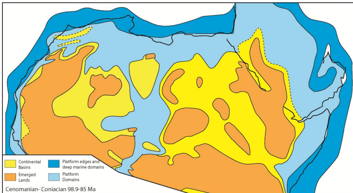
Figure II-12 : Paléogéographie de la plateforme saharienne du Cénomanién au Coniacien. Simplifiée d'après Guiraud et al. (2005).
