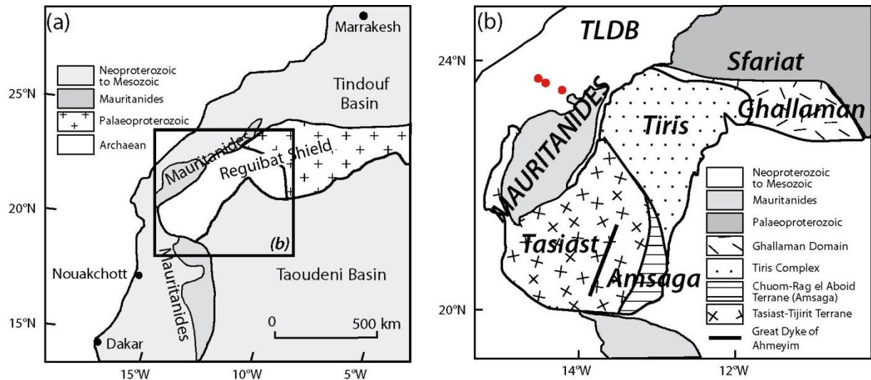
Figure IV-29 : (a) Carte schématique du Nord-ouest du COA. Le rectangle localise la carte (b). (b) Carte des domaines occidental et central du Bouclier Reguibat, avec les noms des différentes sous-régions (d'après Tait et al., 2013). Les points rouges montrent les lieux d'échantillonnage, tous en provenance des dépôts d'âge crétacé inférieur.
