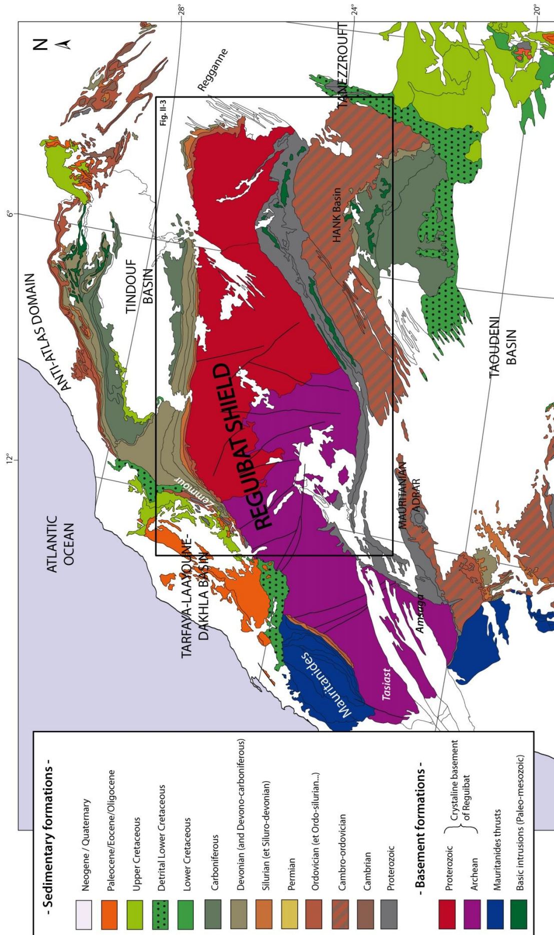
Figure II-2 : Carte géologique du Nord du COA, centrée sur le Bouclier Reguibat. La carte de la figure II-3 est localisée.
