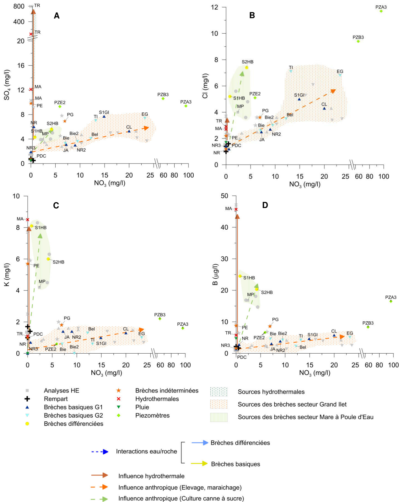
Figure 5.6 : Diagrammes binaires réalisés pour les éléments majeurs et traces analysés lors des campagnes spatiales en basses eaux (anions). Les analyses en hautes eaux sont représentées sous formes de symboles grisés.
