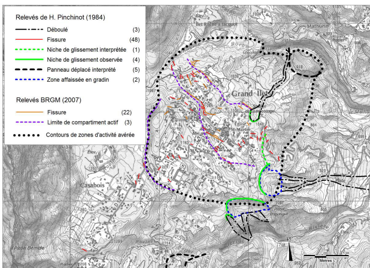
Figure 1.23 : Synthèse des marqueurs de mouvements gravitaires sur le secteur de Grand Ilet. Les relevés effectués par le BRGM en 2007 sont détaillés dans le rapport de Garnier (2008). L'appellation locale « déboulé » désigne les événements de coulées boueuses déclenchées lors du cyclone Hyacinthe en 1980.
