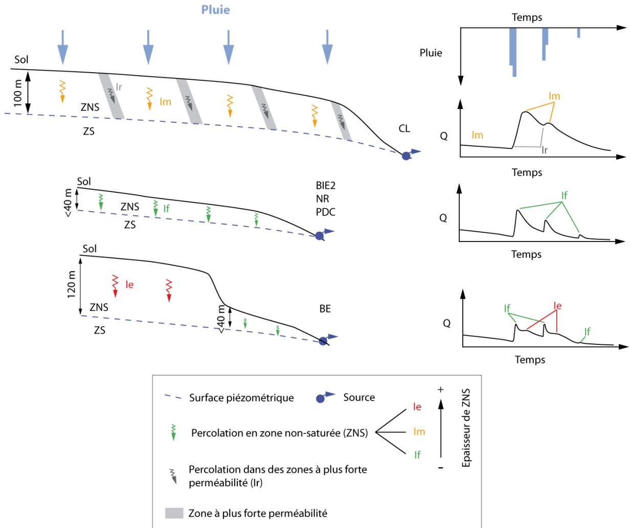
Figure 4.9 : Conceptualisation des processus de recharges des sources des brèches, à partir de l'interprétation des données de piézométrie et de débit des sources, et de la carte d'épaisseur de zone non-saturée (ZS : Zone Saturée ; ZNS : Zone Non-Saturée).
