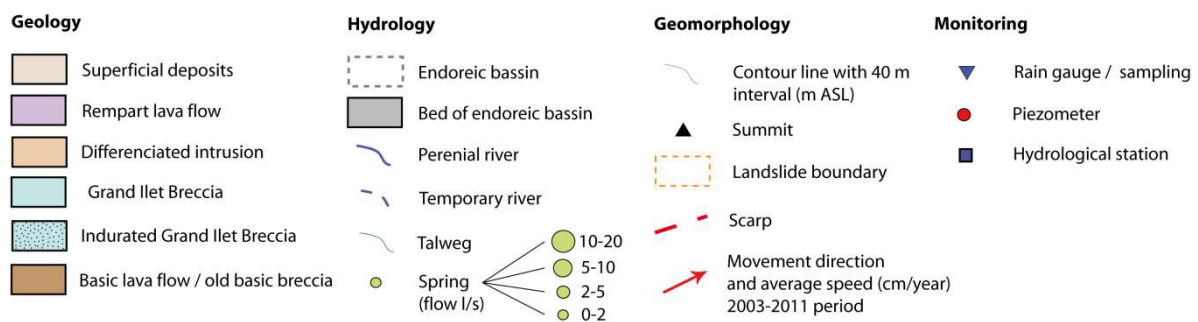
Figure 6.2 : Carte géologique et hydrogéologique du secteur de Grand Ilet. Les dispositifs de suivi des eaux de surface et des eaux souterraines sont également représentés. Les classes de débit sont établies à partir des mesures effectuées à l'été 2011.
