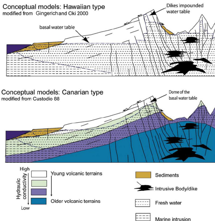
Figure 1.18 : Schémas conceptuels hydrogéologiques des milieux volcaniques, de type hawaïen (Gingerich et Oki, 2000) et de type canarien (Custodio et al., 1988), dans (Join et al., 2005)).
