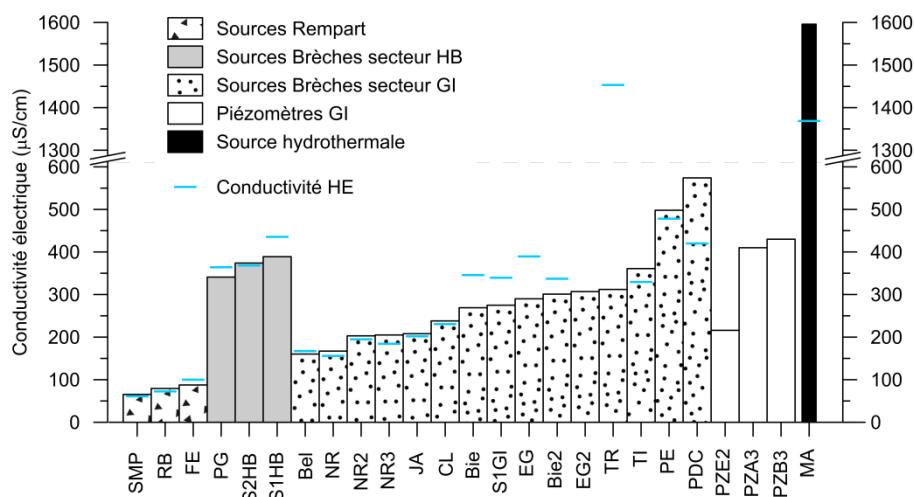
Figure 5.3 : Conductivité électrique à 25°C des sources et des piézomètres dans le cirque de Salazie à l'étiage 2011. Les conductivités des sources RA, TI2 et MP, mesurées uniquement en hautes eaux, ne sont pas reportées.
