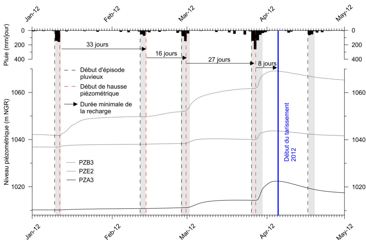
Figure 4.7 : Piézométrie dans PZA3, PZE2 et PZB3 durant les épisodes de recharge de la saison des pluies 2012. La durée minimale de la recharge correspond à la durée entre le début de la hausse piézométrique après un épisode pluvieux et le début de la hausse piézométrique suivante.
