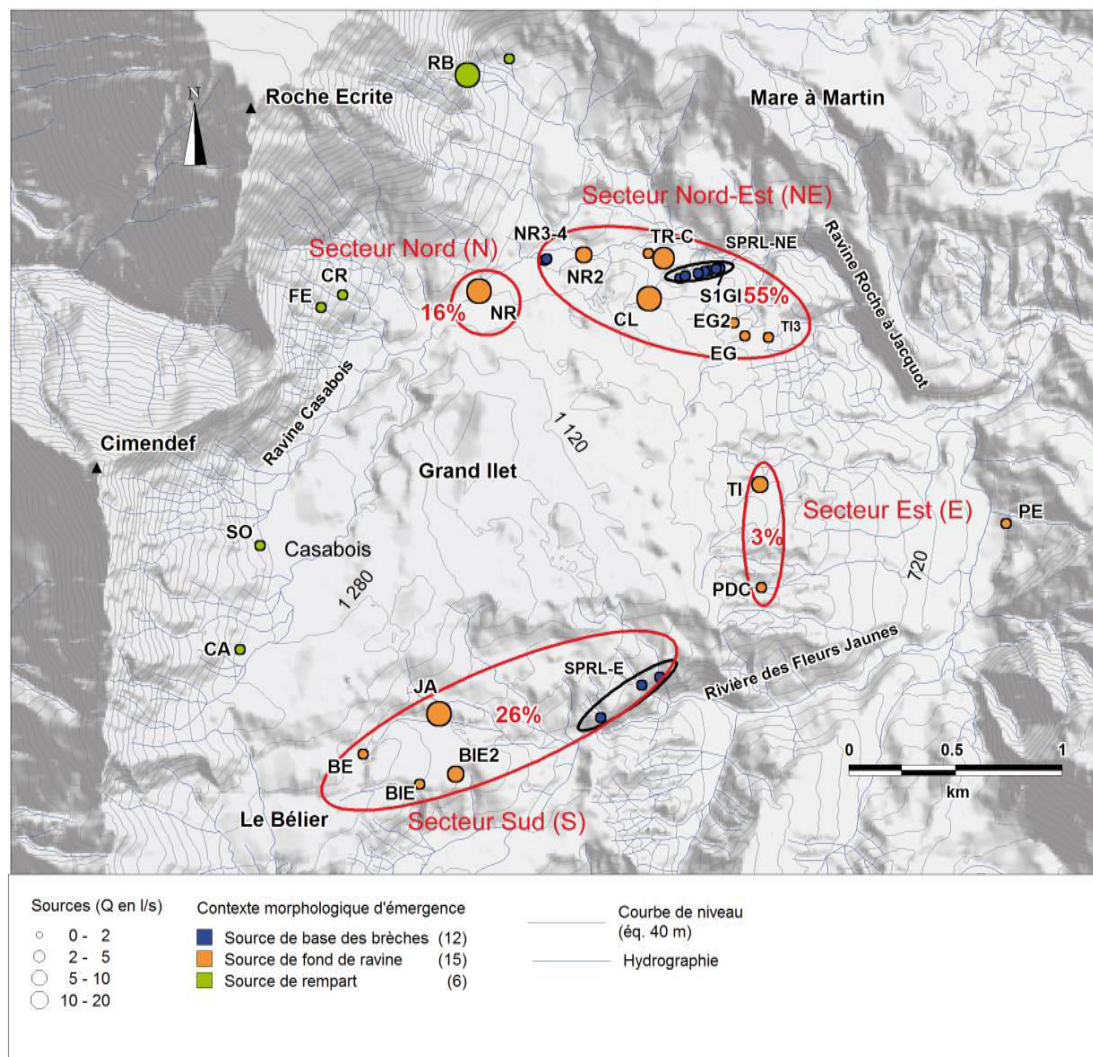
Figure 4.2 : Répartition spatiale des débits d'étiage des sources du secteur de Grand Ilet. Les pourcentages de débits sortants sont calculés par secteur pour les sources des brèches.
