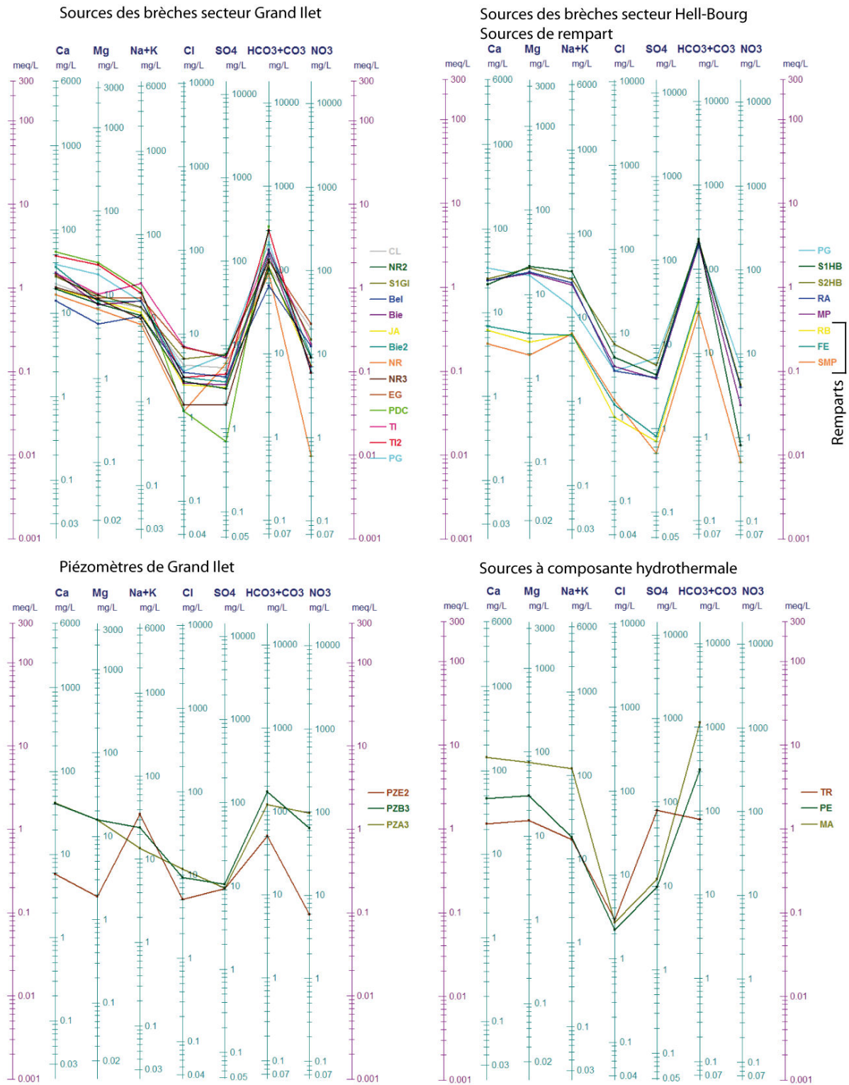
Figure 5.4 : Diagrammes de Schöeller Berkaloff des analyses de la campagne en BE (les sources RA, TI2 et l'analyse de la Mare à Poule d'Eau MP prélevées en HE sont également représentées)
