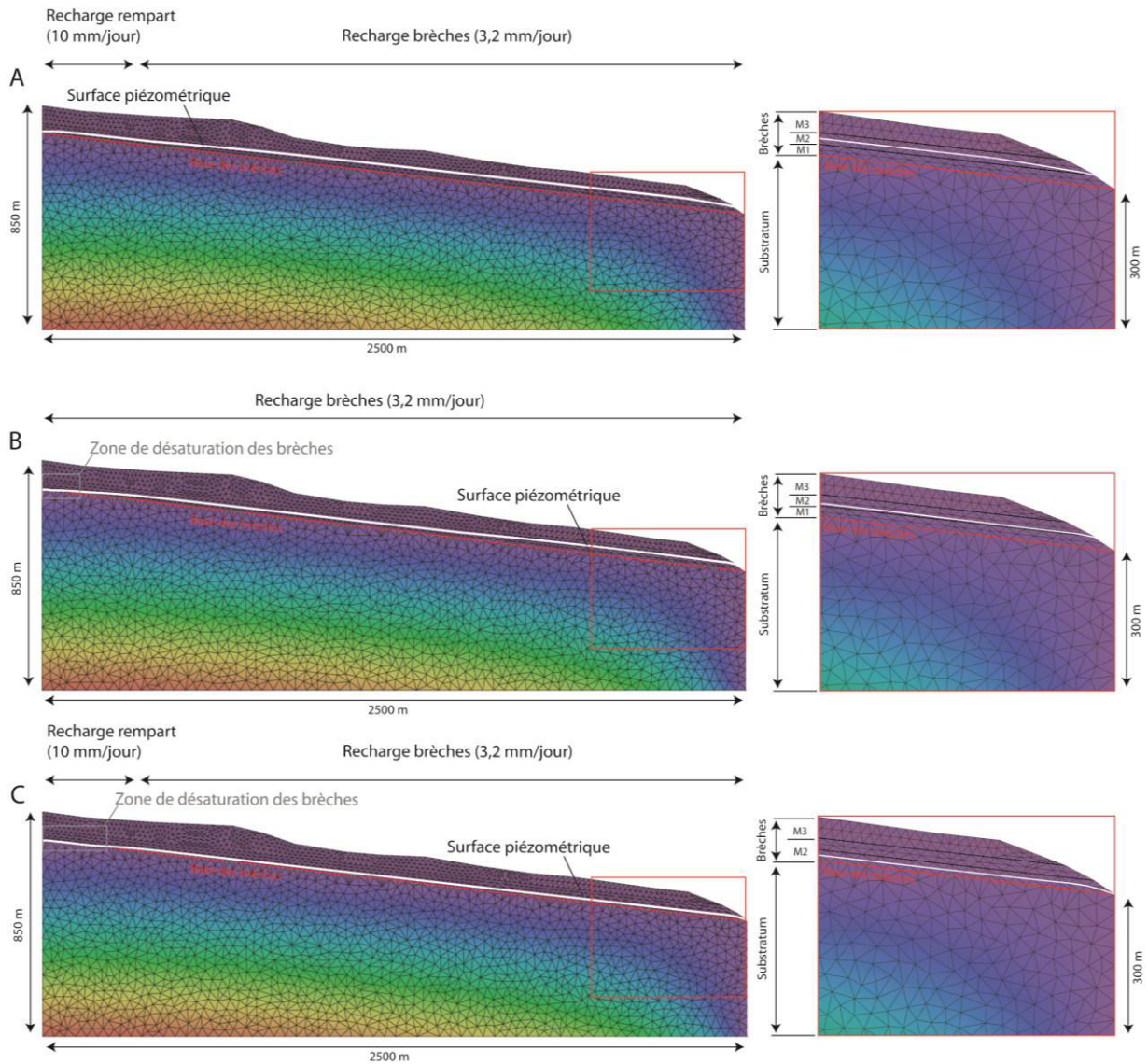
Figure 7.4 : Influence de la recharge et de la conductivité hydraulique des brèches sur la géométrie de la surface piézométrique dans le modèle 2D vertical. A) Modèle initial avec 3 milieux de brèches et la recharge des remparts ; B) Modèle sans la recharge des remparts avec 3 milieux de brèches ; C) Modèle avec la recharge des remparts, sans le milieu M1 à K = 1.10^{-5} m/s.
