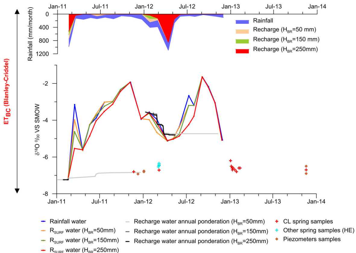
Figure 6.17 : Evolution temporelle (i) de la signature de l'eau du réservoir R_{SURF} (ii) de la signature pondérée de la recharge par cycle hydrologique (Recharge water annual ponderation) pour l'unité de GI, en fonction de la valeur de H_{BR} , en utilisant l' ET_{BC} .
