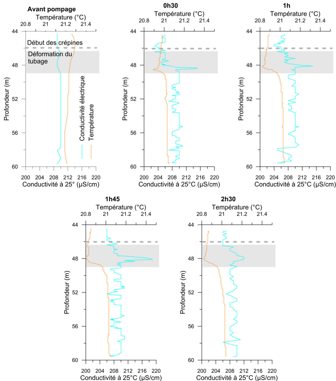
Figure 5.13 : Logs de conductivité électrique (bleu) et de température (orange) réalisés dans le piézomètre PZE2 au cours du pompage réalisé le 10 décembre 2011. La position des crépines et la localisation des zones de déformation des tubages sont représentées sur les graphiques. Le niveau piézométrique est par ailleurs situé à 37,85 m de profondeur.
