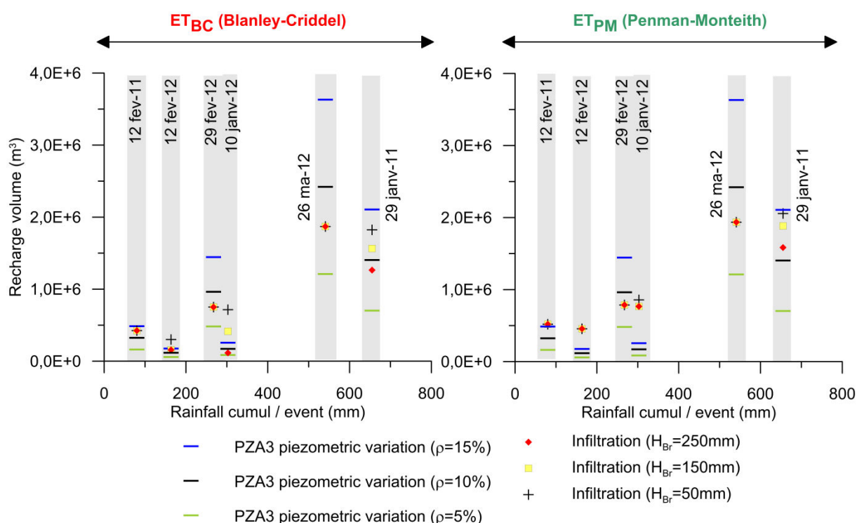
Figure 6.16 : Volumes de recharge estimés par évènement à partir de l'amplitude des variations piézométriques (pour différentes valeurs de porosité) et par le calcul du bilan, en fonction des cumuls de pluie par évènement pour l'unité de Grand Ilet.
