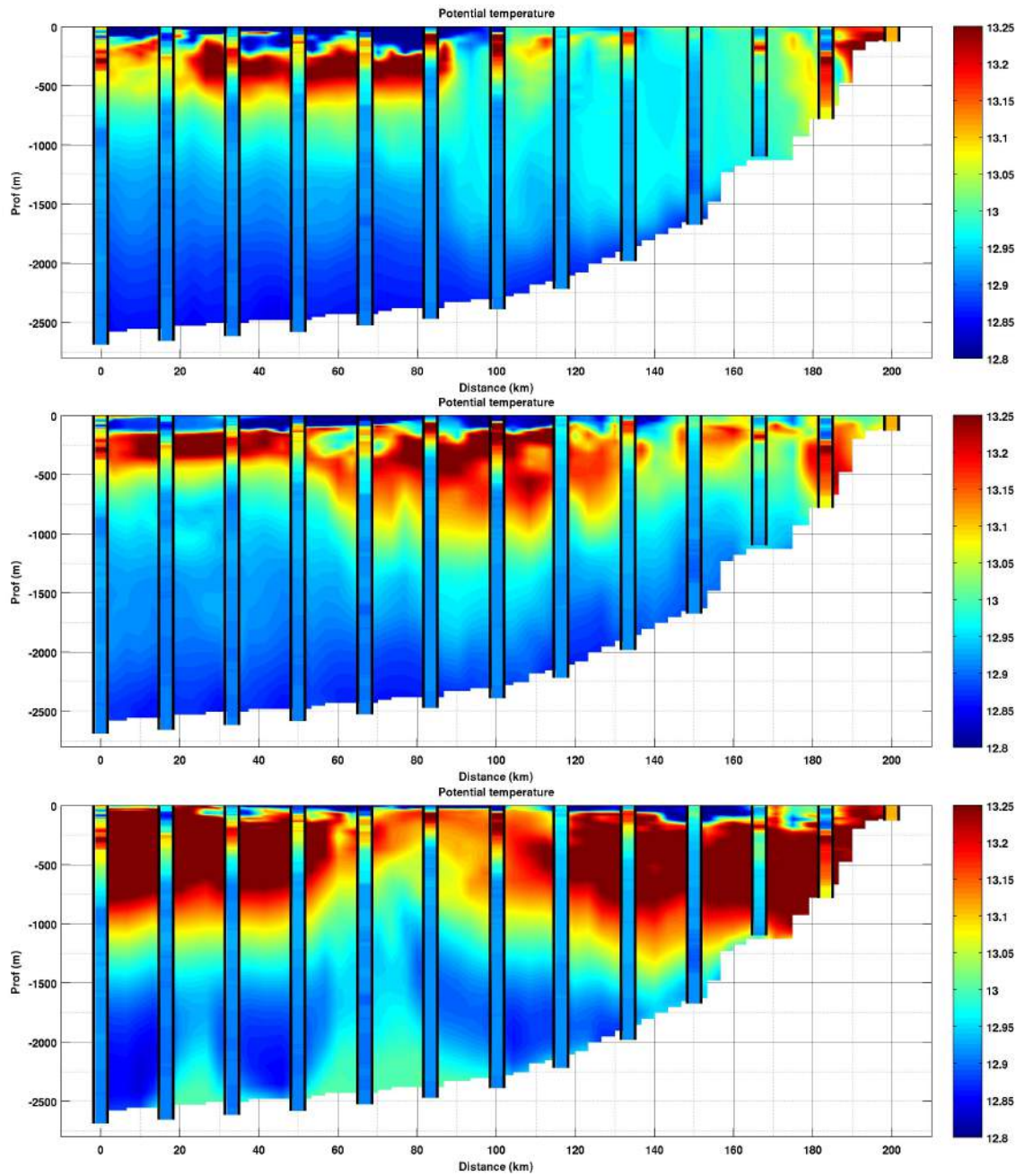
FIGURE A.7 – Comparisons des valeurs de température potentielle observées pendant la radiale M de CAS-CADE avec celles modélisées par les configurations : (en haut) Convec1kmEcm, (au milieu) Convec1kmArp, (en bas) ConvecObcArp. Les profils CTD le long de la radiale sont superposés au champ de température potentielle modélisé et co-localisé.
