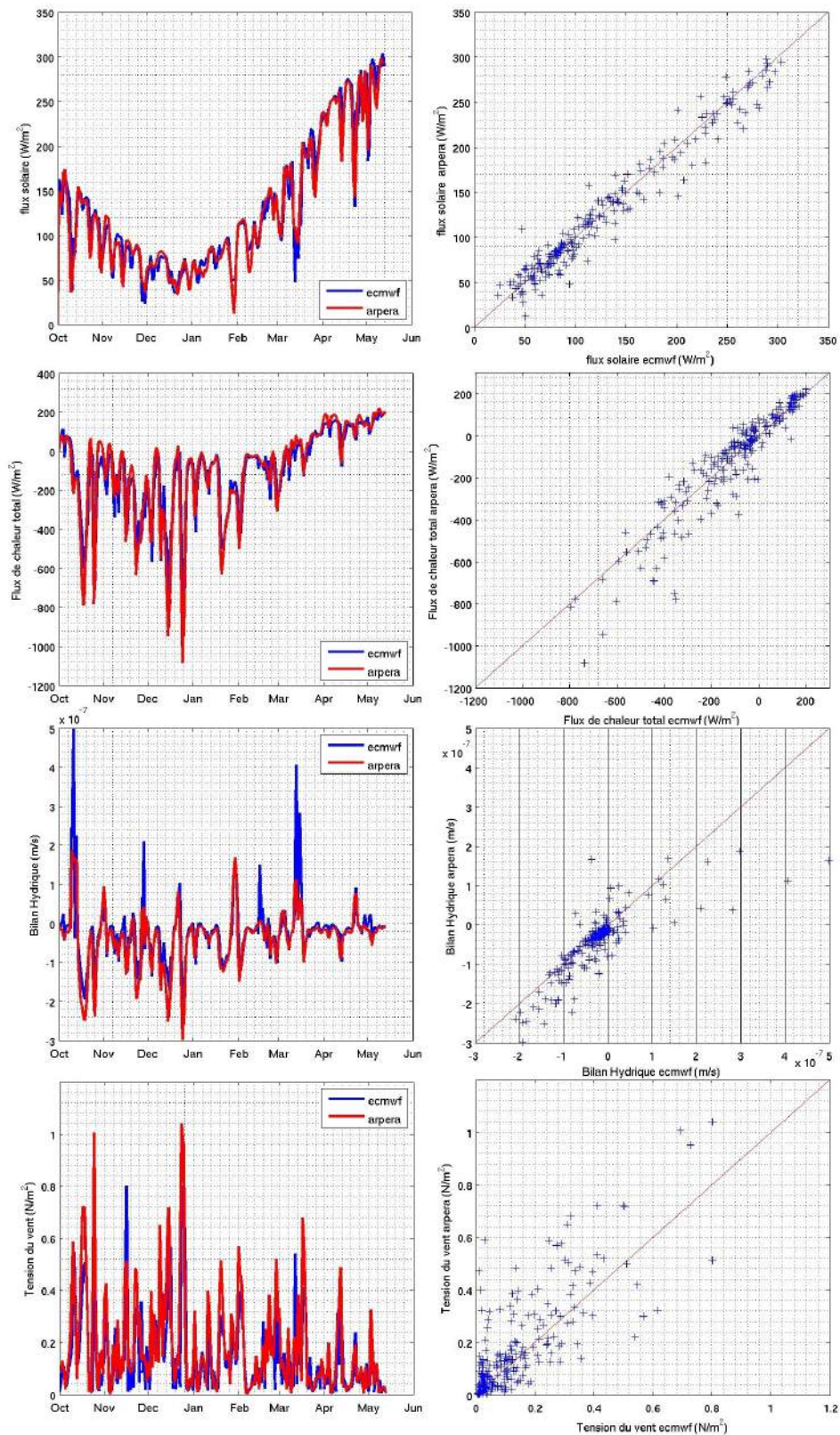
FIGURE 3.20 – Comparaison des moyennes des flux atmosphériques en sortie du modèle utilisés dans les configurations dans un rectangle centré sur la zone de convection ( 150km*100km ). On représente les évolutions respectives (à gauche) et les comparaisons (à droite) du flux solaire, du flux de chaleur total, du bilan hydrique (précipitation - évaporation) et de la tension du vent (de haut en bas).
