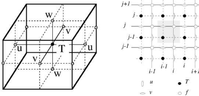
FIGURE 2.5 – Arrangement des variables sur la grille C-Arakawa et son indexation horizontale associée.
