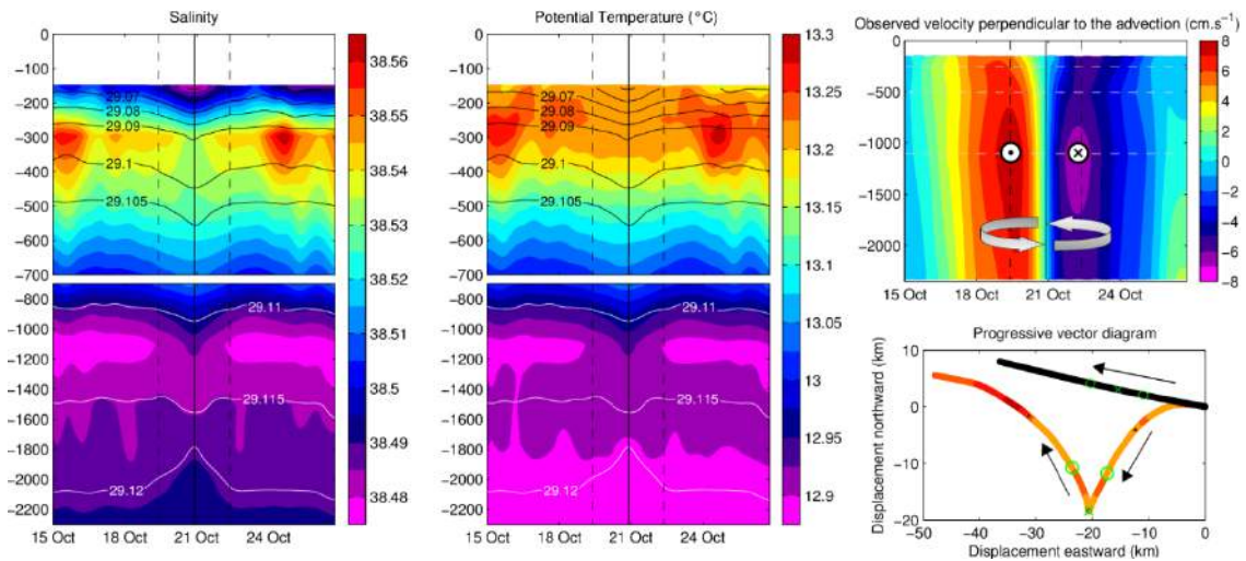
FIGURE 5.2 – Coupe de temp erature potentielle, de salinit e, du champs de vitesse d'un cyclone de subm eso echelle traversant la ligne du mouillage Lion le 21 octobre 2010 (source : Houpert et al. [2014a])
