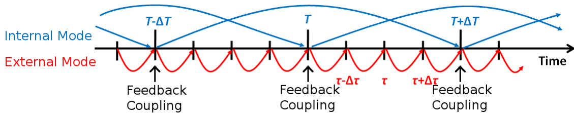
FIGURE 2.6 – Illustration de la technique du "time-splitting" et du couplage barotrope/barocline.
