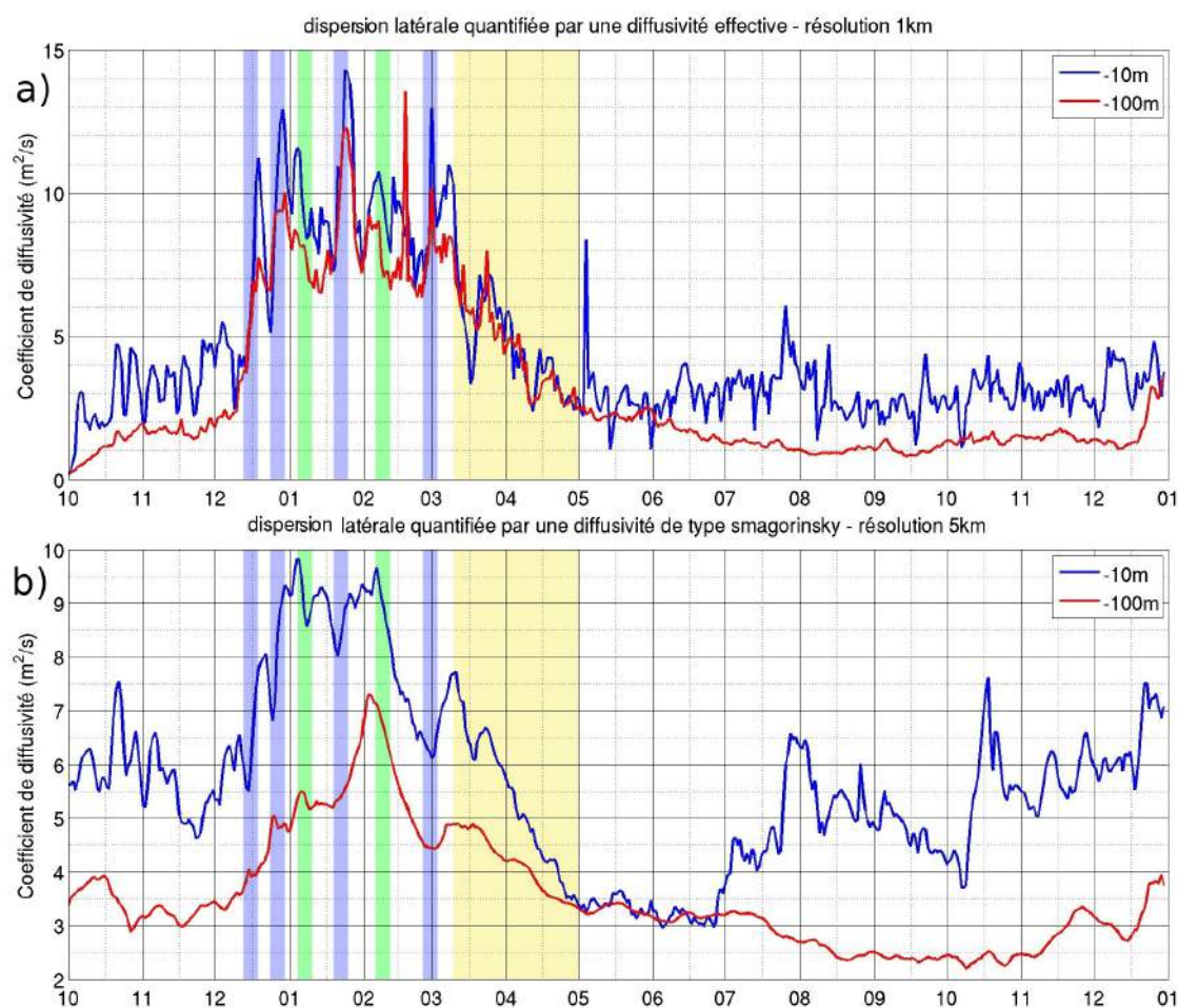
FIGURE 4.22 – Evolution du coefficient de diffusivité moyenné sur la zone de convection à (bleu) 10m et (rouge) 100m de profondeur. En haut, le coefficient \kappa_{app,5km} est calculé de manière effective dans le modèle à 1km de résolution. En bas, il est calculé comme un coefficient de diffusivité de sous maille de type Smagorinsky dans le modèle à 5km de résolution.
