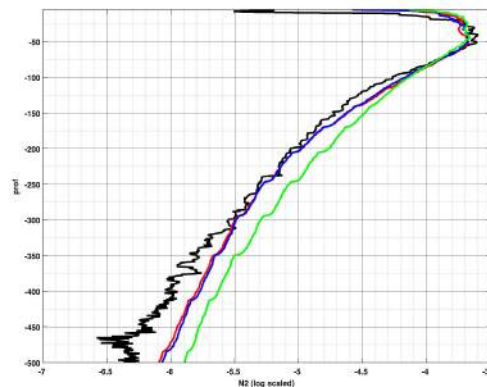
FIGURE 3.8 – Profil de la fréquence de stratification N^2 moyenne (échelle logarithmique décimale) des observations (noir) et des configurations Convec1kmEcm (bleu), Convec1kmArp (rouge) et ConvecObcArp (vert).
