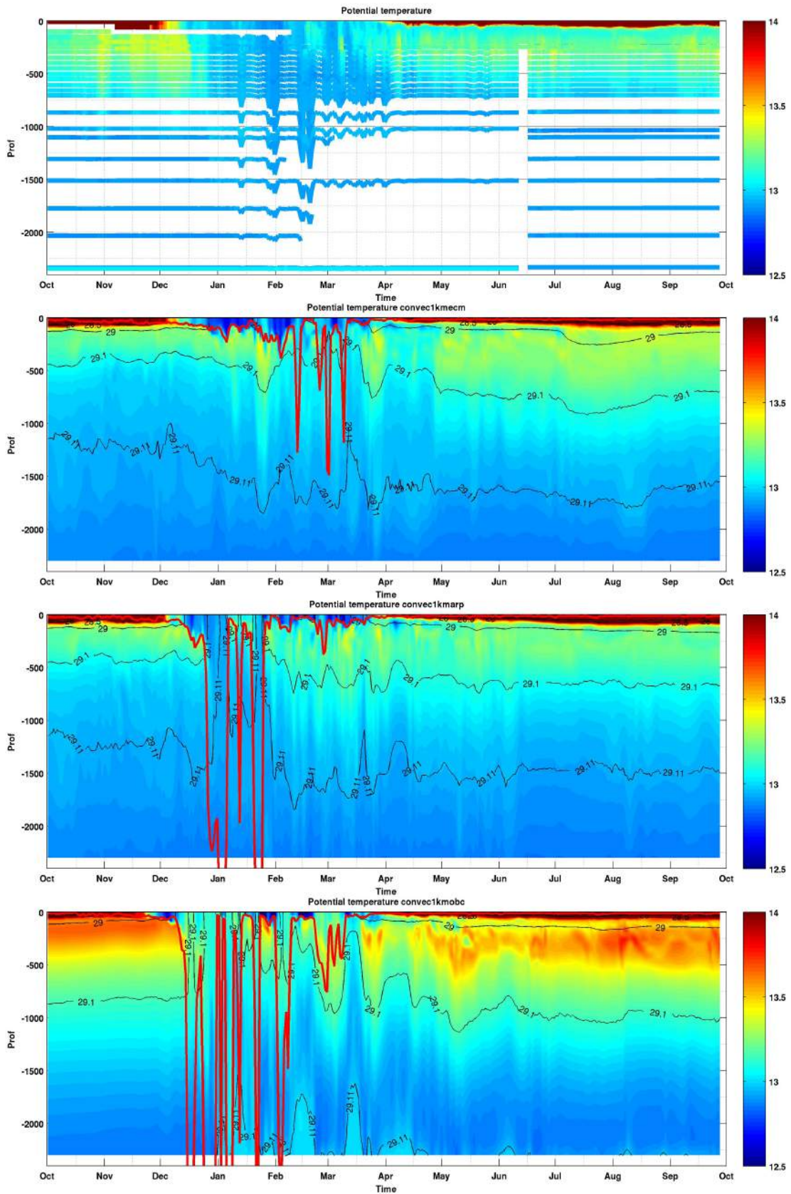
FIGURE 3.11 – Serie temporelle de la température potentielle au mouillage issue (de haut en bas) des observations et des configurations Convec1kEcm, Convec1kArp et ConvecObcArp. La courbe rouge indique la profondeur de la couche de mélange avec un critère de densité à 10m + 0.01kg.m^{-3} .
