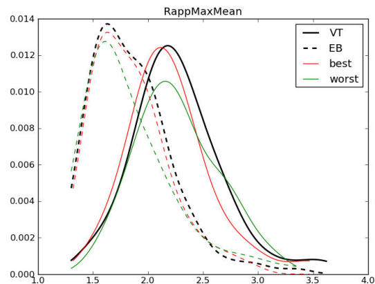
FIG. II.3.13: Densités de probabilités pour RappMaxMean pour les VT (courbes pleines) et les EB (courbes tiretées). La couleur noire correspond aux densités de probabilité calculées sur l'ensemble du training set (100%); la couleur rouge, à celles calculées pour le tirage ( sub-training set 60%) ayant permis d'obtenir la meilleure classification; la couleur verte, à celles du moins bon tirage.
