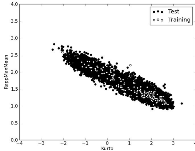
FIG. II.3.4: Corrélation entre deux attributs : kurtosis et rapport du maximum sur la moyenne de l'enveloppe.
