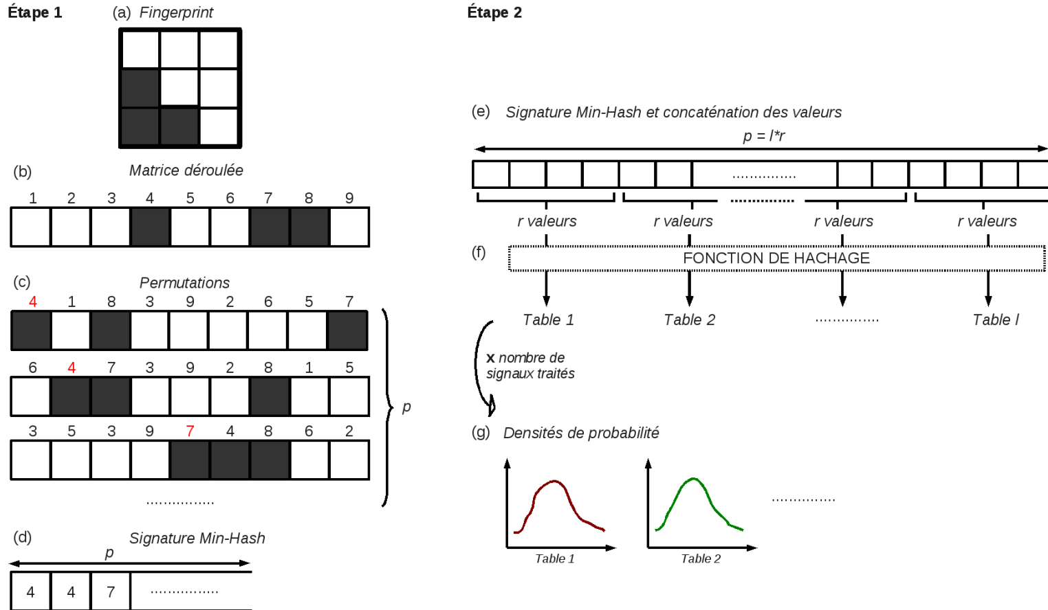
FIG. I.2.33: ( Gauche ) Schéma explicatif pour la génération de la signature Min-Hash. (a) Empreinte (matrice). Les cases noircies correspondent aux bits de valeur 1. (b) Matrice de l'empreinte déroulée. (c) p permutations de l'ordre des bits de la matrice déroulée. (d) Écriture de la signature Min-Hash : vecteur de longueur p comprenant les positions du premier bit de valeur 1 pour chaque permutation. ( Droite ) Schéma explicatif pour la génération des tables de hachage. (e) Concaténation de la signature Min-Hash par découpage en l groupes de valeurs disjointes des autres groupes. (f) Calcul des l valeurs de hachage pour chaque table via la fonction de hachage. (g) Densités de probabilité calculées pour chaque table à partir de l'ensemble des valeurs de hachage.
