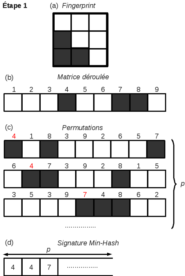
FIG. I.2.33: (Gauche) Schéma explicatif pour la génération de la signature Min-Hash. (a) Empreinte (matrice). Les cases noircies correspondent aux bits de valeur 1. (b) Matrice de l’empreinte déroulée. (c) p permutations de l’ordre des bits de la matrice déroulée. (d) Écriture de la signature Min-Hash : vecteur de longueur p comprenant les positions du premier bit de valeur 1 pour chaque permutation. (Droite) Schéma explicatif pour la génération des tables de hachage. (e) Concaténation de la signature Min-Hash par découpage en l groupes de valeurs disjointes des autres groupes. (f) Calcul des l valeurs de hachage pour chaque table via la fonction de hachage. (g) Densités de probabilité calculées pour chaque table à partir de l’ensemble des valeurs de hachage.
