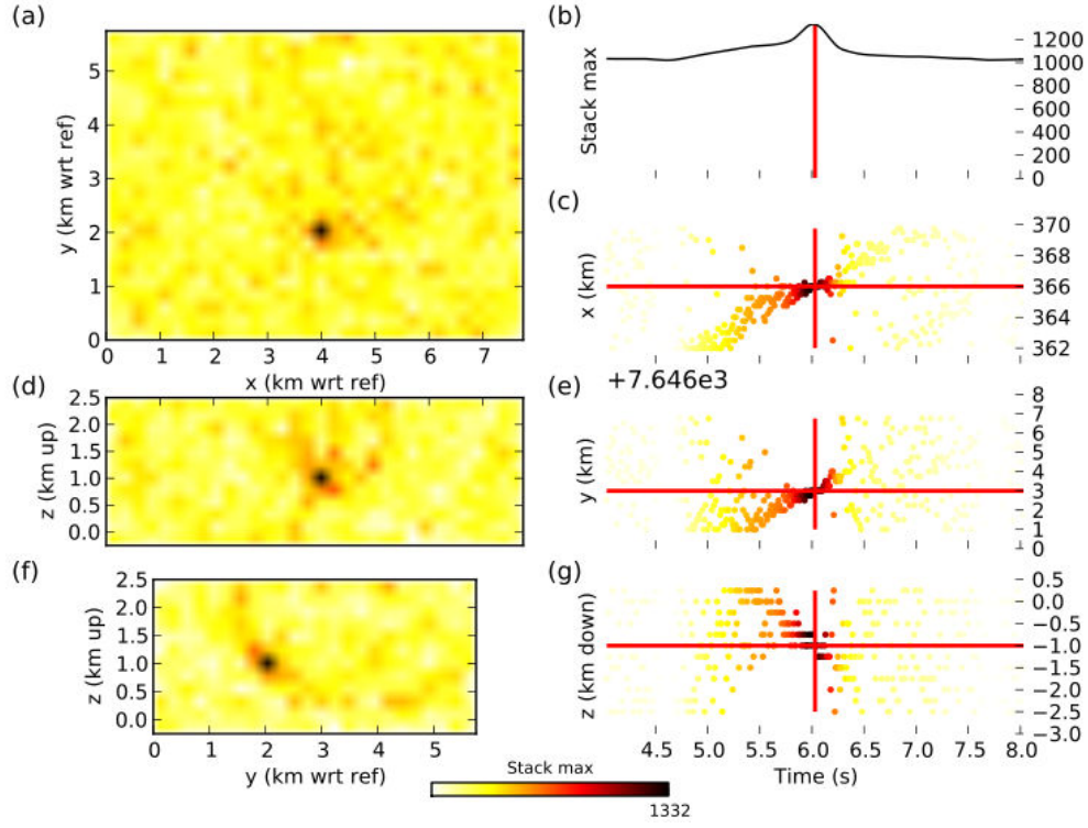
FIG. I.1.8: Test synthétique visant à montrer la capacité de Waveloc à localiser un événement avec un SNR de 1.5. Pour le détail concernant la description des sous-figures, se référer à la figure I.1.6.
