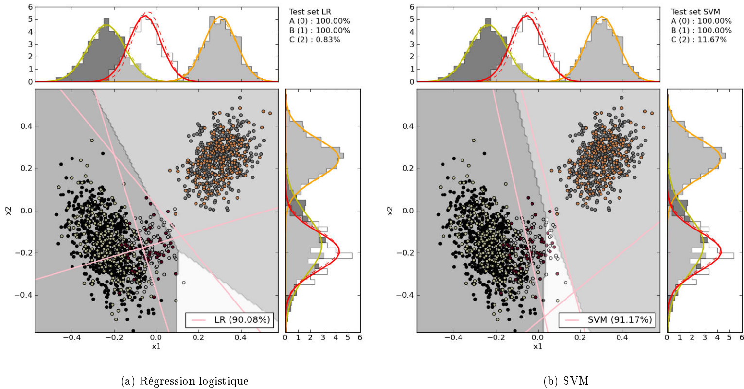
FIG. III.1.4: Résultats de la classification pour un jeu de données synthétique comportant 3 classes inégalement réparties pour la régression logistique (a) et la SVM linéaire (b). La classe noire constitue 50% des données; la grise 40% et la blanche 10%. Les éléments du training set sont également représentés (en jaune, orange et rouge respectivement). Les densités de probabilité associées aux deux caractéristiques x_1 et x_2 sont visibles de part et d'autre de la figure, avec les courbes continues pour le test set et les courbes tiretées pour le training set .
