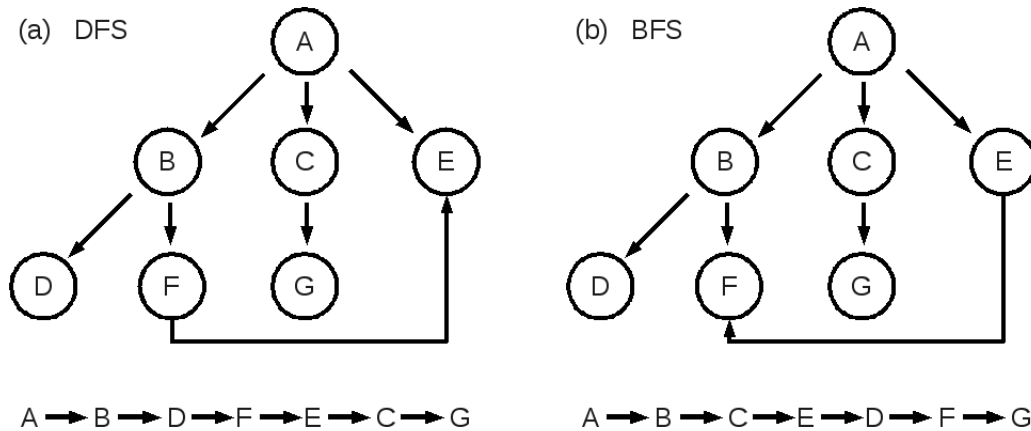
FIG. I.1.9: (a) Algorithme de DFS. (b) Algorithme de BFS. On considère 7 événements : l'événement A est fortement corrélé à B, C et E. B est corrélé avec A, D et F ; C avec A et G ; D avec B ; E avec A et F ; F avec B et E ; et G avec C. En partant du sommet A, l'algorithme DFS va explorer d'abord trouver B, puis D. En D, la branche se termine, il revient au niveau précédent et examine le deuxième événement corrélé à B (F)... et ainsi de suite. L'algorithme BFS, quant à lui, explore tous les "niveaux" d'un coup : il trouve d'abord tous les événements corrélés à A, puis à B...
