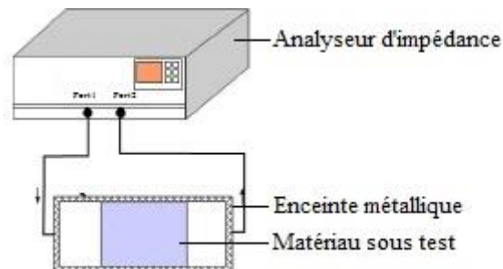
Figure V.28 : Schéma du dispositif de mesure en cavité résonante.
