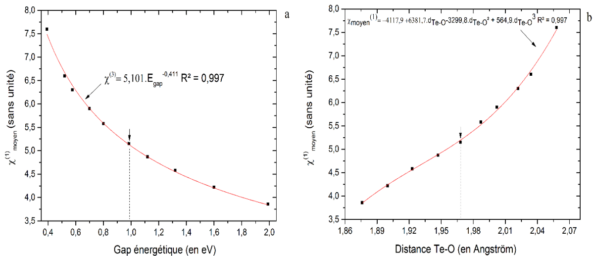
Figure IV.10 : (a) Evolution de la susceptibilité optique linéaire d'ordre 1 moyenne en fonction du gap énergétique du composé TeO 3 -β, (b) Evolution de la susceptibilité optique non-linéaire d'ordre 1 moyenne en fonction de la longueur de liaison dans le composé TeO 3 -β. La ligne en pointillé indique la distance Te-O de la structure de référence.
