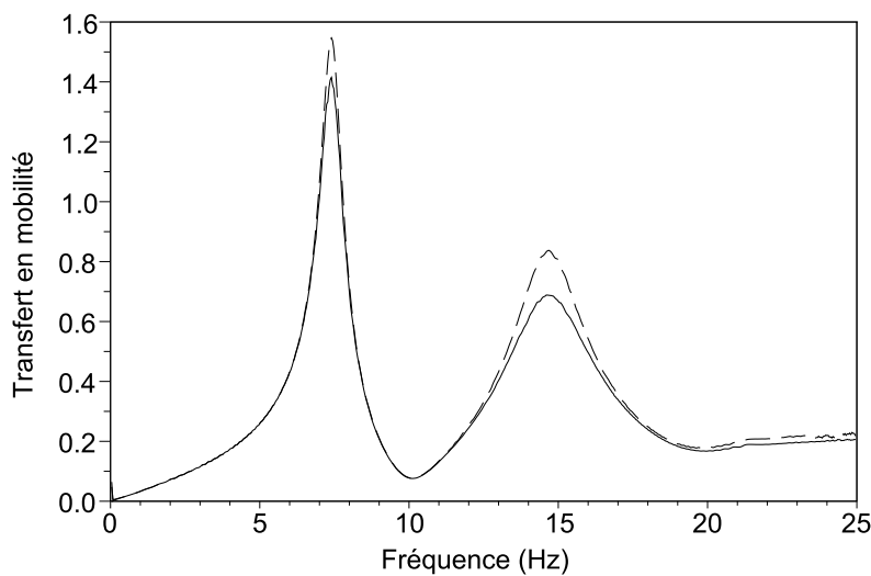
FIGURE V.50 – Fonctions de transfert en mobilité obtenues pour un pilotage en déplacement d'amplitude 0,8\text{ mm} (ligne pleine) et pour un pilotage en force d'amplitude 50\text{ N} (en pointillés).
