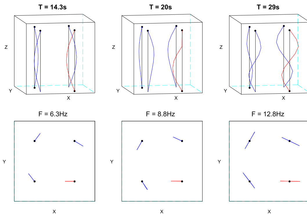
FIGURE V.45 – Premier POM obtenu aux pics d'énergie des assemblages 2, 3 et 4, pour un essai simulé en eau stagnante, d'amplitude 0,8\text{ mm} . La SWPOD est ici appliquée à chaque assemblage séparément.
