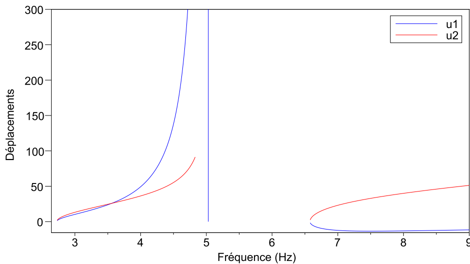
FIGURE III.2 – Tracé des déplacements des masses 1 et 2 aux résonances en fonction des fréquences de résonance des premier, second et troisième modes, pour une approximation à 1 harmonique. ( u_1 en bleu, u_2 en rouge)
