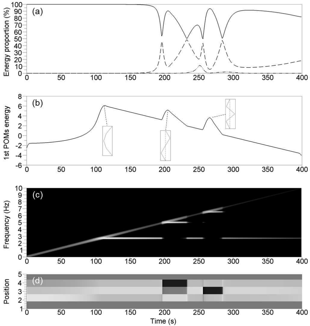
FIGURE III.5 – Résultats pour un test avec \xi_1 = 0,1\% et F_a = 10\text{ N} . (a) Proportions d'énergie capturées par le premier (ligne pleine), second (pointillés) et troisième (points) POMs. (b) Energie capturée par le premier POM. (c) Représentation temps-fréquence de la première POC multipliée par sa POV associée \lambda_1^T \hat{G}_1(\tau, f) . (d) Evolution temporelle du premier POM \Phi_1^T .
