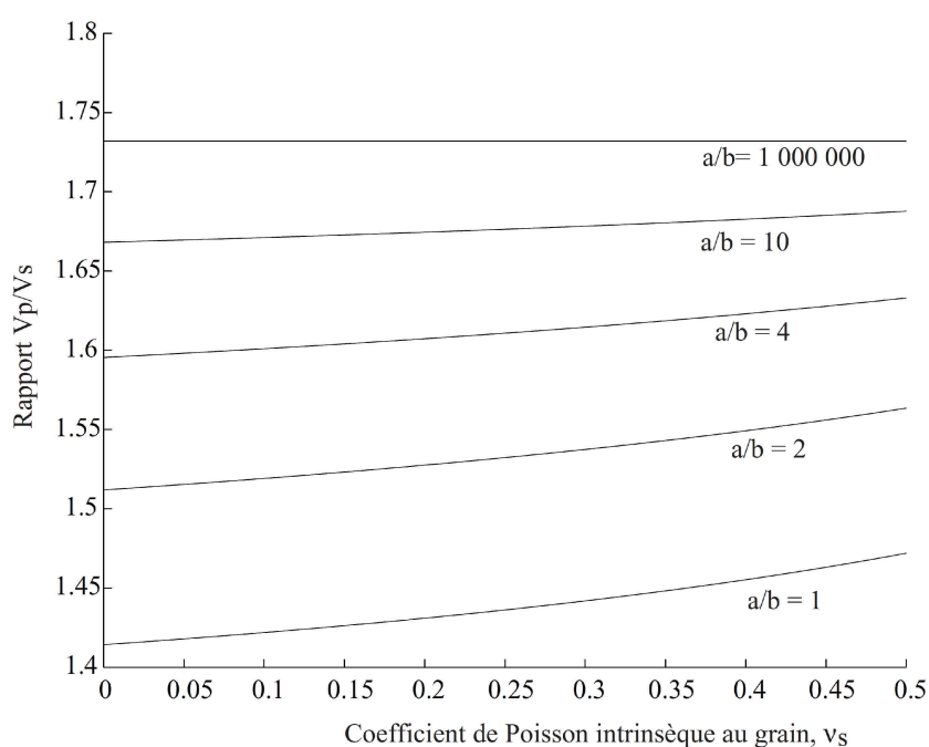
FIGURE 23 – Évolution du rapport V_P/V_S en fonction du coefficient de Poisson intrinsèque au grain, et en fonction du rapport a/b , d'après [Digby, 1981].
