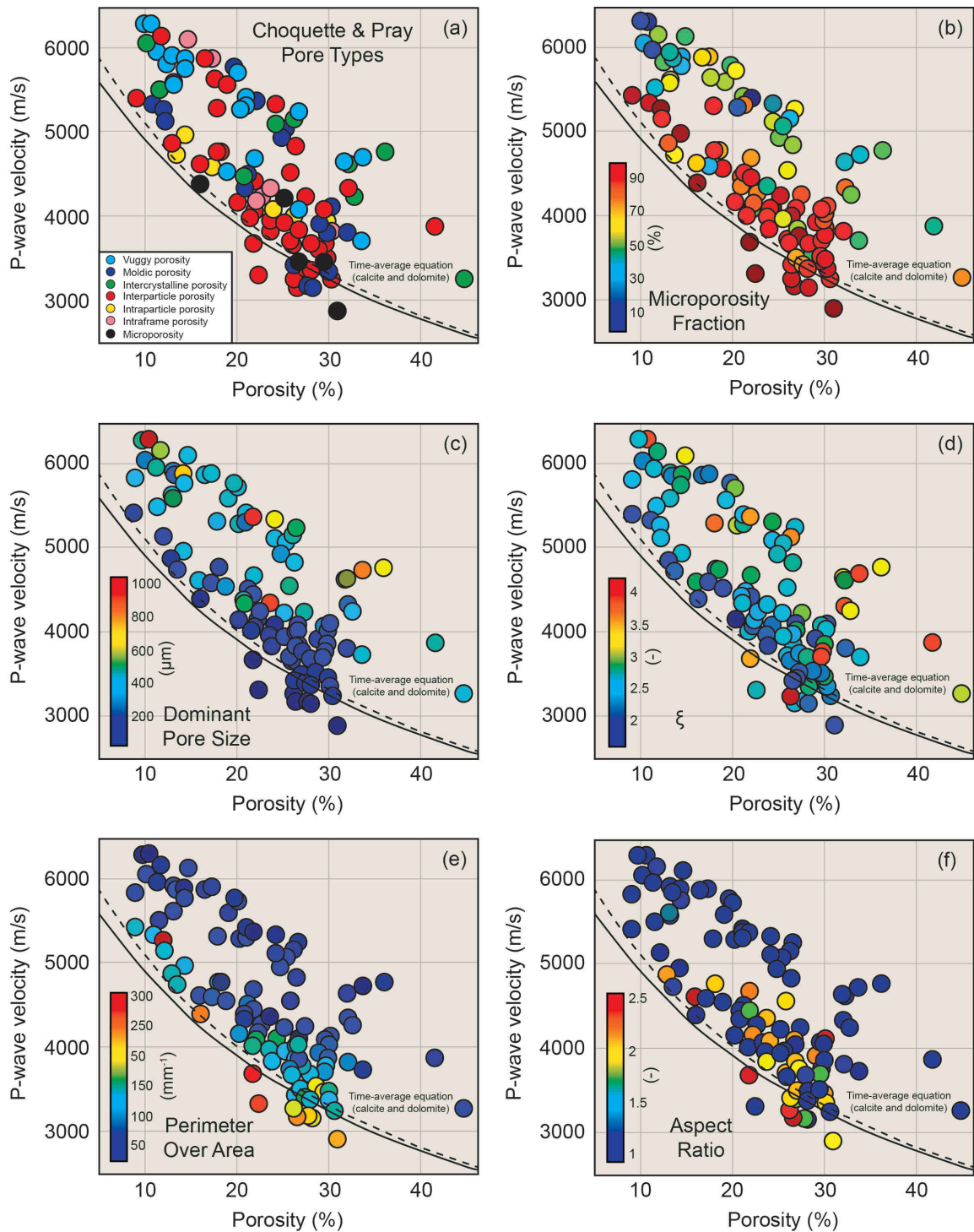
FIGURE 8 – Influence de la proportion de microporosité (%), de la taille moyenne des pores (DomSize), leur arrondi ( \xi ), la surface spécifique moyenne des pores (PoA) et leur aspect ratio, sur les valeurs de V_P . Modifié d'après Weger et al. [2009].
