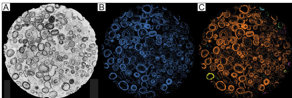
FIGURE 82 – Orthoslices obtenue au nano-Ct scan pour un échantillon microporeux. A - image brute obtenue. B - Réseau poreux (bleu) après traitement et seuillage de la matrice minérale (noire). C - Connectivité du réseau poreux. Les zones de même couleur sont des zones connectées. Makhloufi et al. [2013].
