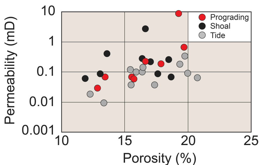
FIGURE 83 – Données de porosité et de perméabilité pour l’Oolithe Blanche des carrières de Bourgogne, Makhloufi et al. [2013].
