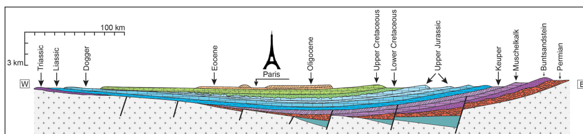
FIGURE 26 – Coupe théorique Est-Ouest du Bassin de Paris, modifié d'après Delmas et al. [2010].
