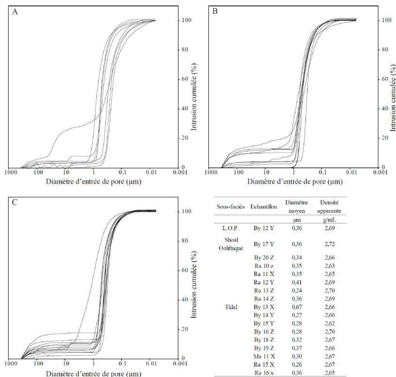
FIGURE 81 – Porosimétrie mercure sur une sélection d'échantillons de l'Oolithe Blanche, Makhloufi et al. [2013].
