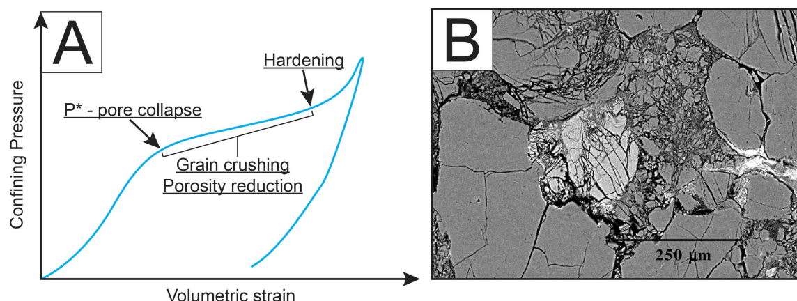
FIGURE 70 – A - Comportement mécanique d’une roche poreuse sous régime hydrostatique. B - Effondrement des pores ( pore collapse ) et rupture (ou broyage) des grains ( grain crushing ) à la pression P^* dans le grès de Darley Dale [Wong et al. 1999].
