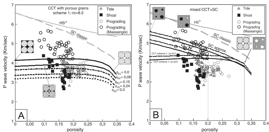
FIGURE 24 – Modélisation des propriétés effectives dans la formation de l'Oolithe Blanche du bassin de Paris [Casteleyn et al. 2011]. A - Approche auto-cohérente (A – C) qui explique les variations de vitesse dans les faciès progradant principalement dominés par la macroporosité dans le ciment. B - Modèle de contacts de sphères cimentées ( CSC ) modifié [Dvorkin et al. 1999] qui montre que les vitesses dans les faciès de shoal et tidaux sont gouvernées par la microporosité dans les ooides.
