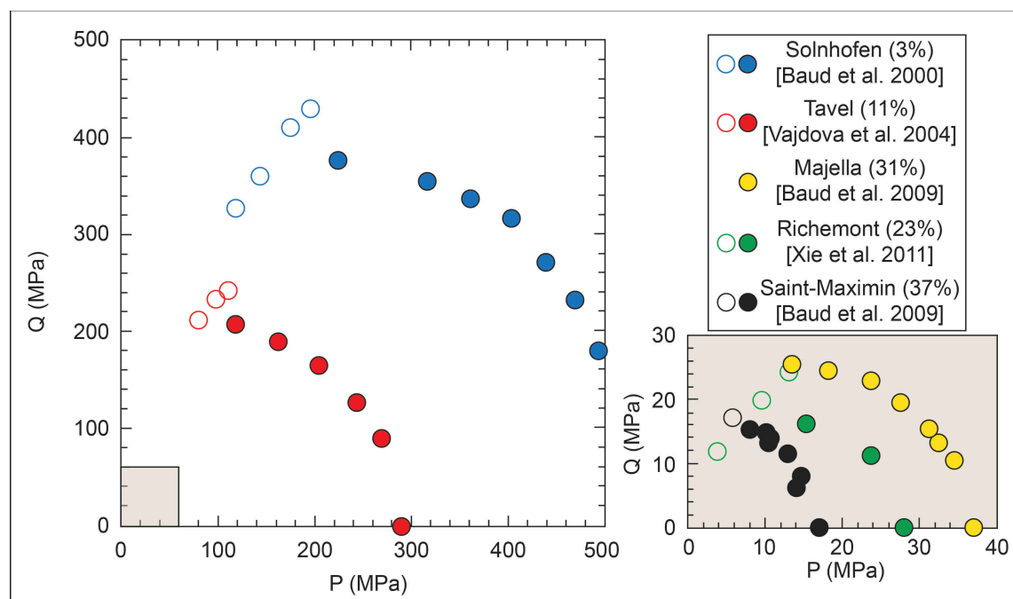
FIGURE 73 – Enveloppes de rupture pour différents calcaires, issues de la littérature [Wong et al. 2012]. Les symboles ouverts correspondent à la contrainte à la rupture, et les symboles fermés correspondent à C^* , la pression maximale avant la compaction inélastique.
