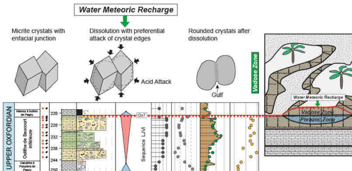
FIGURE 61 – Émersion au sommet de la Séquence LJVI et phénomènes associés observés dans le forage EST205.
