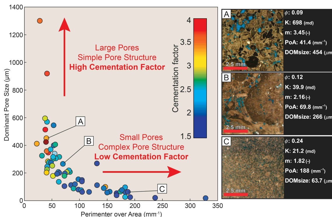
FIGURE 19 – Crossplots de la surface spécifique des pores ( PoA ) et de la taille de pore dominante. Les données sont discriminées par les valeurs de l'exposant de cimentation m . Les photos représentent les différentes combinaisons des paramètres. Modifié d'après Verwer et al. [2011].
