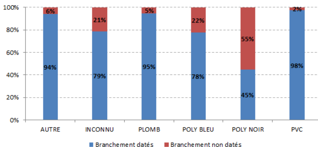
FIGURE 2.5 – Datation finale des branchements par nature de matériau
