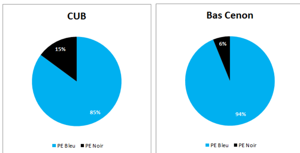
FIGURE 4.21 – Comparaison du patrimoine branchements entre le réseau de la CUB et le sous-secteur du Bas Cenon
