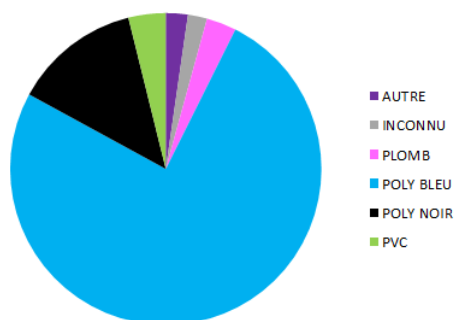
FIGURE 2.4 – Répartition par matériau du nombre de branchements (source MMS-APIC , 2014)
