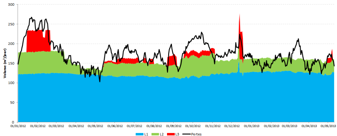
FIGURE 4.23 – Décomposition de la chronique des pertes selon les trois états de dégradation
