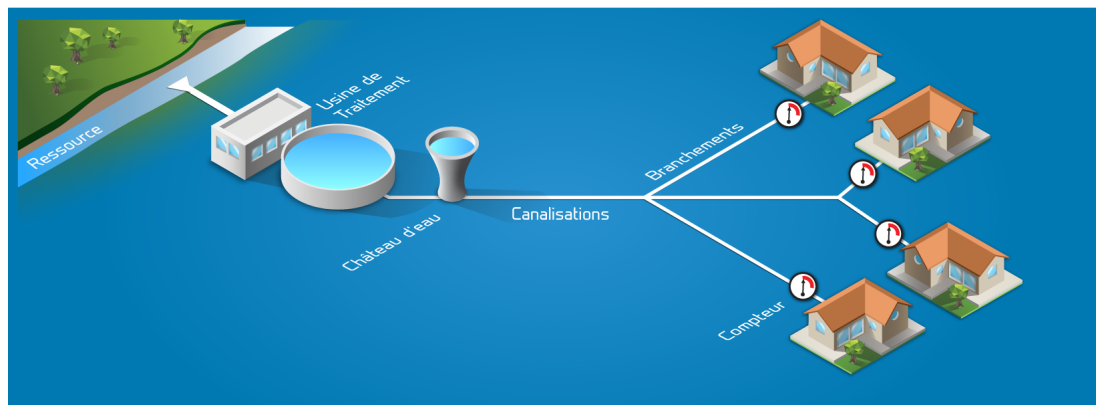
FIGURE 2.1 – Schéma du réseau d'adduction d'eau potable.
