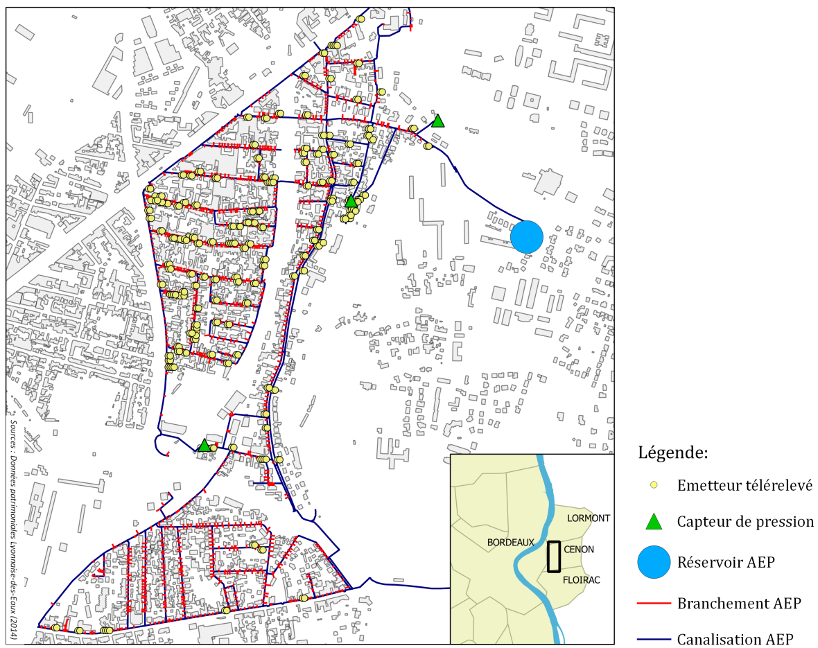
FIGURE 2.10 – Le réseau d'alimentation en eau potable (AEP) de la Cote 50 à Cenon
