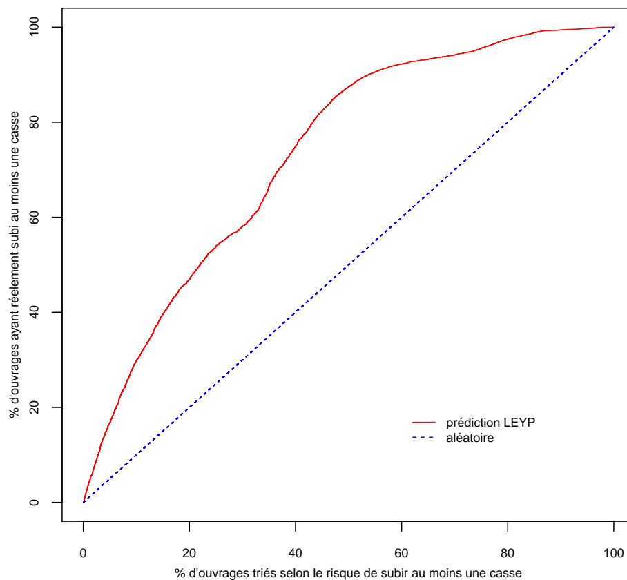
FIGURE 4.13 – Qualité d’ajustement pour le modèle LEYP
