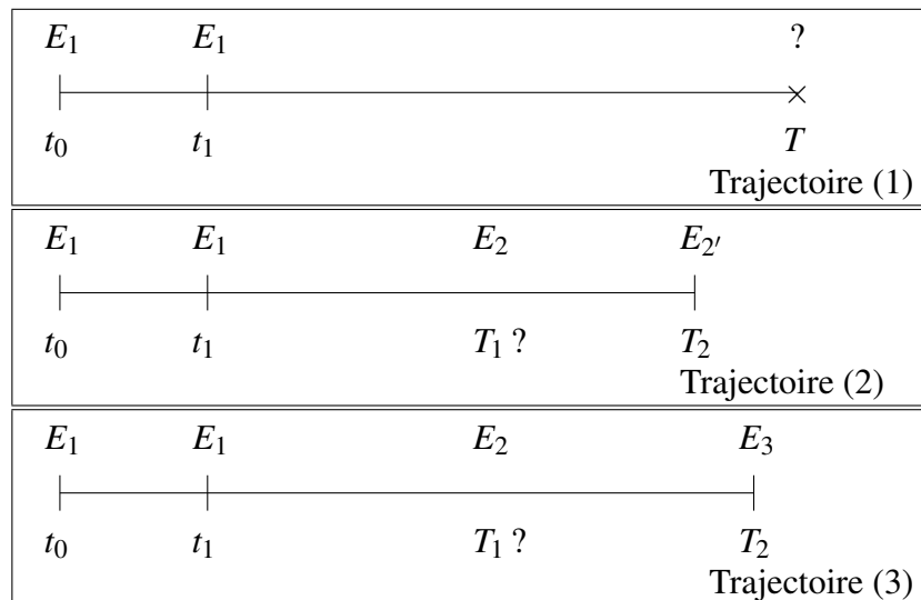
FIGURE 4.17 – Trajectoires observables pour le modèle MED
