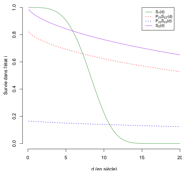
FIGURE 4.18 – Fonction de survie pour les ouvrages en Fonte Grise - Amiante Ciment
