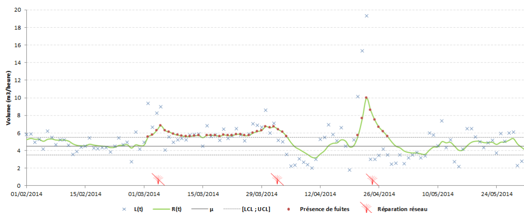
FIGURE 4.6 – Carte de contrôle EWMA pour la détection des fuites sur le secteur de la Cote 50
