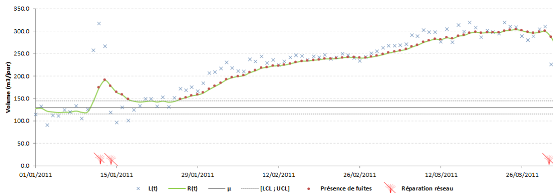
FIGURE 4.5 – Carte de contrôle EWMA pour la détection des fuites sur le secteur de Canéjan
