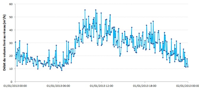
FIGURE 2.6 – Débits de volumes livrés
