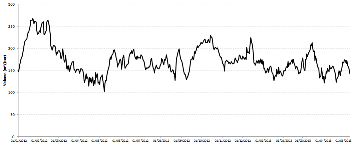
FIGURE 4.22 – Chronique des pertes à décomposer à l'aide du modèle de débit de fuite
