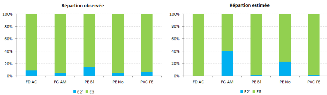
FIGURE 4.15 – Validation du modèle de risques concurrents
