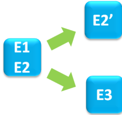
FIGURE 4.14 – Le modèle de risques compétitifs
