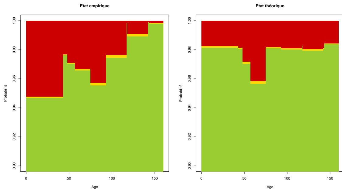
FIGURE 4.11 – Résultats d’estimation des probabilités d’appartenance à un état du modèle GompitZ pour le matériau Fonte Grise-Amiante Ciment par classe d’âge (vert = E_1 , jaune = E_2 , rouge = E_3 )
