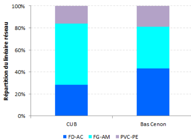
FIGURE 4.20 – Comparaison du patrimoine canalisations entre le réseau de la CUB et le sous-secteur du Bas Cenon
