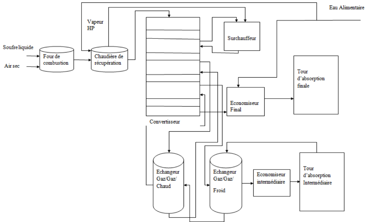
Figure 2.8. Unité de préparation d'acide sulfurique
