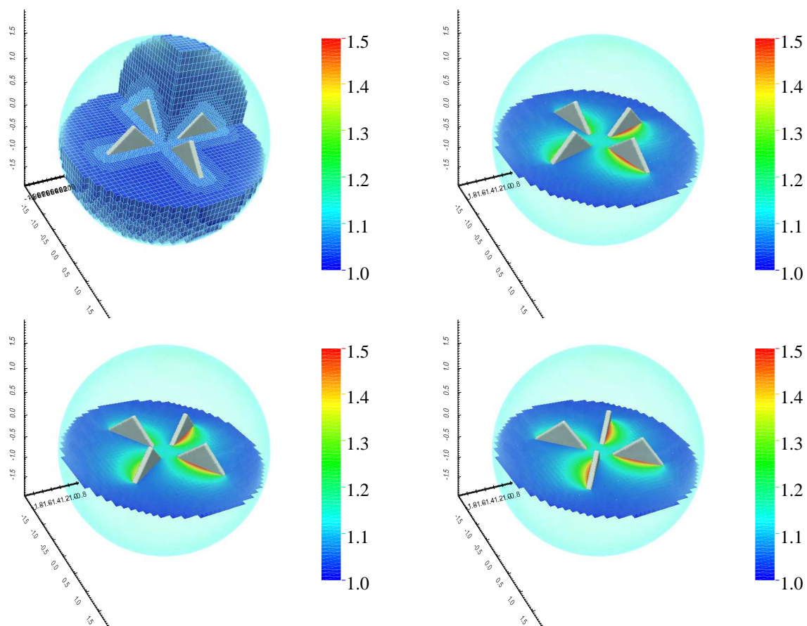
FIGURE 4.14 – Résultats de la simulation 3D du radiomètre de Crookes pour Kn = 0.5 . Le champ de température T/T_0 sur le plan z = 0 est représenté à t \times L/\sqrt{2RT_0} = 0, 5, 10 et 15 (de gauche à droite et de haut en bas). Le maillage est visible sur l'image représentant l'instant initial.
