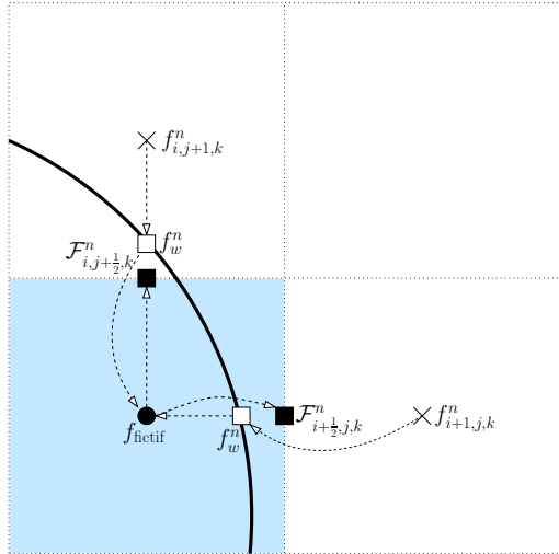
FIGURE 2.13 – Procédure de calcul du flux : après interpolation de la valeur de la fonction de distribution sur la paroi, puis dans la maille fictive bleutée, le flux est déterminé par les éq. (2.24). et (2.25)
