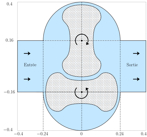
(b) Géométrie complète de la pompe. Toutes les unités sont données en mètre et les lobes sont construits avec r = 0.038\text{m}
