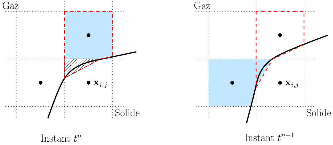
FIGURE 3.13 – Sur la gauche, la maille virtuelle hachurée \bar{\mathcal{C}}_{i,j}(t^n) fusionne avec la maille bleutée \bar{\mathcal{C}}_{i,j+1}(t^n) car L_{i,j+\frac{1}{2}}^n est supérieur à L_{i-\frac{1}{2},j}^n . Le volume de contrôle \mathcal{C}_{i,j}^n résultant de cette fusion est tracé avec la ligne pointillée rouge. Sur la droite, le même volume de contrôle au pas de temps suivant, c'est-à-dire \mathcal{C}_{i,j}^{n+1,*} , est toujours tracé avec la ligne pointillée rouge. Maintenant, la maille virtuelle \bar{\mathcal{C}}_{i,j}(t^{n+1}) va fusionner avec \bar{\mathcal{C}}_{i-1,j}(t^{n+1}) car L_{i-\frac{1}{2},j}^{n+1} est devenu plus grand que L_{i,j+\frac{1}{2}}^{n+1} . Le nouveau volume de contrôle \mathcal{C}_{i,j}^{n+1} est bleuté.
