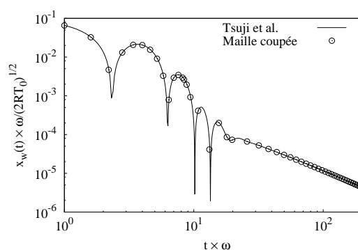
(b) La position initiale du piston est x_w^0 = 0.1 \sqrt{2RT_0}/\omega .
