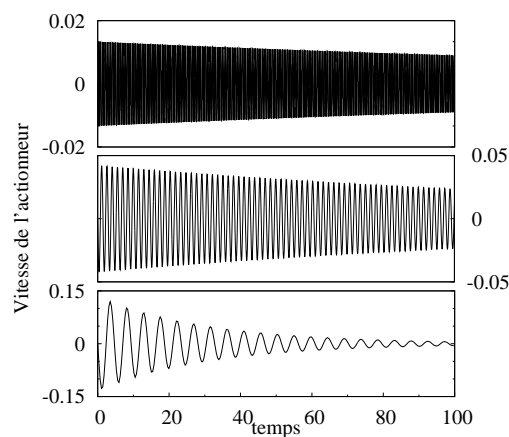
(b) Simulations avec maille fictive de la vitesse de l'actionneur pour trois valeur de L_0 . De bas en haut : 100cm, 10cm et 1cm.
