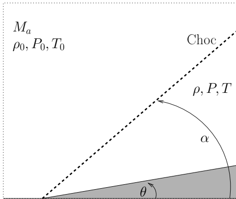
(a) Configuration de l'écoulement : le solide est grisé et la vitesse d'entrée à gauche est horizontale. Le choc est représenté par la ligne pointillée.
