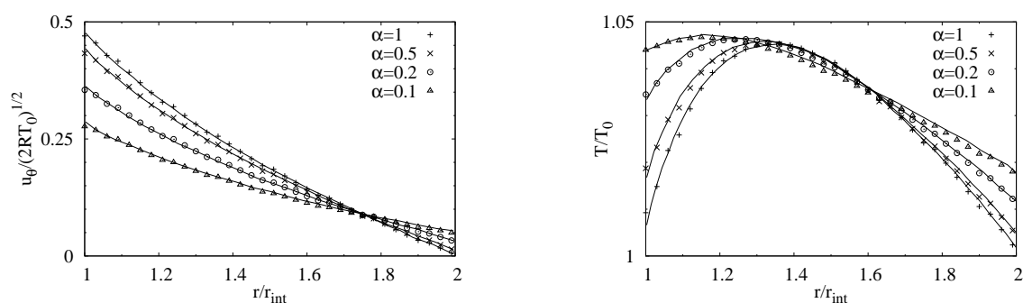
(a) Profils de vitesse radiale. La solution pour la méthode maille coupée est prise sur le rayon horizontal.
