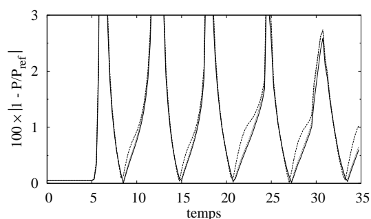
(b) Paroi fixe : seule la discrétisation maillage conforme de l'équation BGK est tracée car elle se superpose avec celles sur grille cartésienne.
