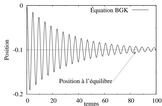
(d) Position de l'actionneur : simulation faite avec la méthode maille coupée.
