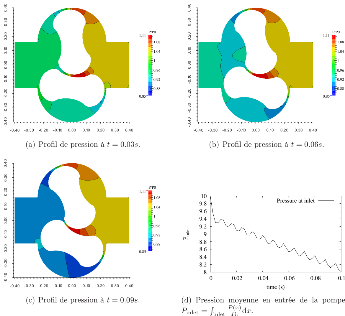
FIGURE 3.21 – Champs de pression à différents instants obtenus avec le schéma semi-implicite d'ordre 1, sur un maillage 200^2 .
