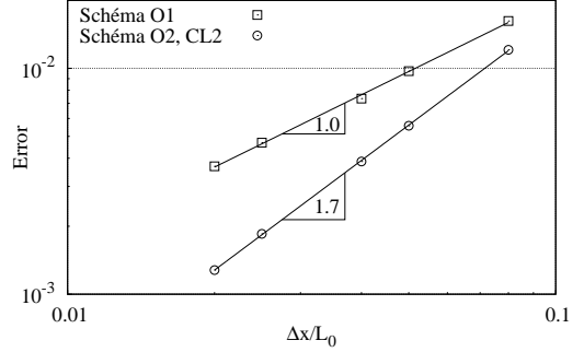
(b) Convergence de la vitesse. L'erreur vaut \epsilon(\Delta x) = \sum |u_x^n(\Delta x) - u_x^n(\frac{1}{2}\Delta x)|/u_\infty , où u_x^n est la vitesse des cylindres au temps 0.2n \times L_0/\sqrt{2RT_0} . L'indice n prend les valeurs de 1 à 500 dans la somme.
