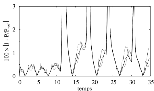
(a) Paroi mobile : seule la discrétisation maillage conforme de l'équation BGK est tracée car elle se superpose avec celles sur grille cartésienne.
