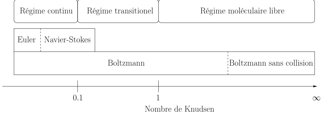
FIGURE 1.1 – Modèles associés aux différents régimes en fonction du nombre de Knudsen.
