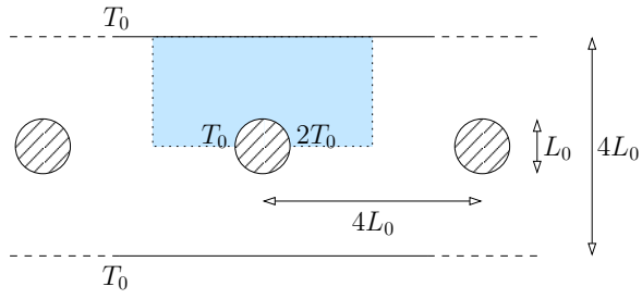
(a) Configuration de l'écoulement. Le domaine de calcul est bleuté, et la température sur les cylindre est donnée par T(\theta \in [-\pi, \pi]) = (2 - \frac{\theta}{\pi})T_0 .
