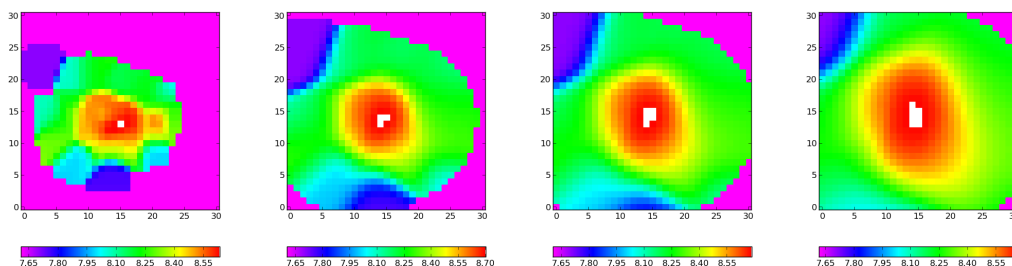
FIGURE 8.1 : Cartes de métallicité du disque isolé en rotation, la résolution varie de gauche à droite : 0,15'' ; 0,50'' ; 0,65'' ; 0,85'' . La métallicité a été calculée en utilisant la calibration Pérez-Montero & Contini (2009) pour chaque pixel et est représentée selon les couleurs sur l'échelle en dessous des cartes dans les unités de 12 + \log(O/H) .
