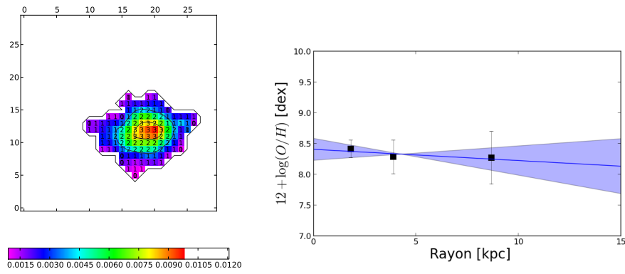
FIGURE 7.3 : Galaxie 020218856, à gauche, carte de flux H \alpha , en 10^{-15} ergs s ^{-1} cm ^{-2} , à droite, gradient de métallicité.
