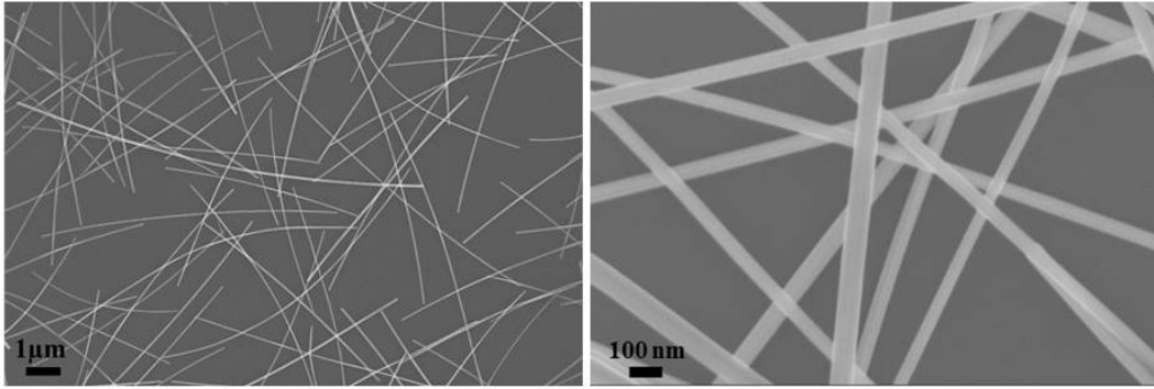
FIGURE 2.22 – Clichés MEB à différents grossissements de Ag NF ( d = 65 \pm 15 nm ; L = 11 \pm 3 \mu\text{m} ).
