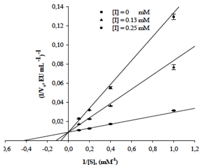
Figure 31: Les graphiques de Lineweaver-Burk de l'inhibition de l'activité de la PPO de champignon de couche sur le pyrogallol par l'acide benzoïque. Concentrations de l'acide benzoïque sont : 0 ( \blacksquare ), 0.13 ( \blacktriangle ), et 0.25 ( \bullet ) mM.
