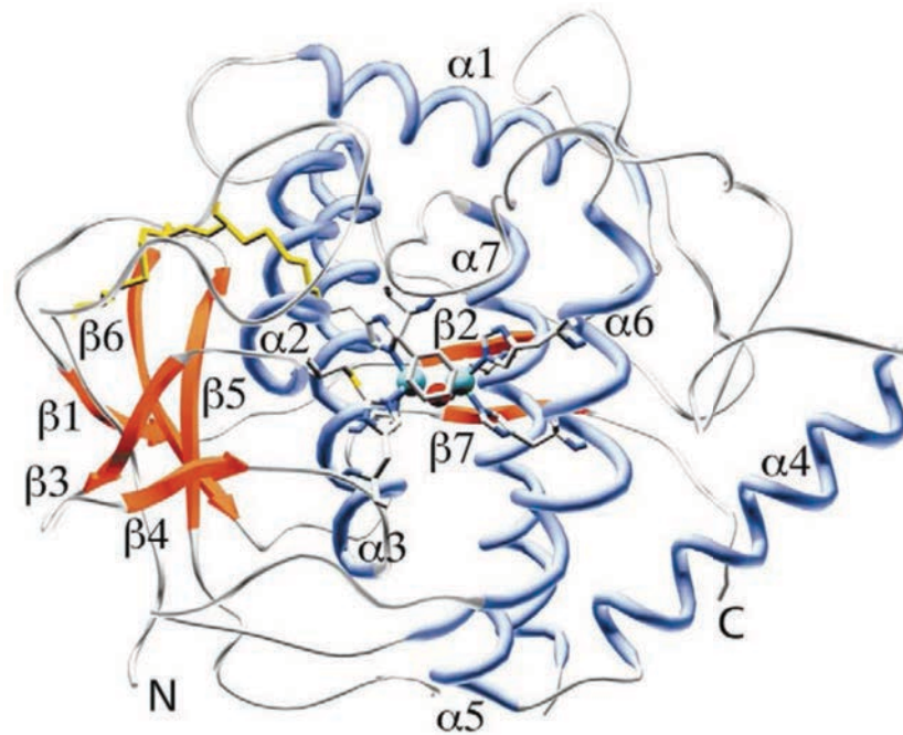
Figure 2: Vue de face de la catéchol oxydase de 39 Kda (les atomes sont colorés par le type d'atome : carbone : gris, l'azote : bleu, soufre : jaune, oxygène : rouge, cuivre : cyan (Eicken et al., 1999).
