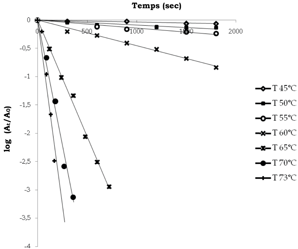
Figure 28: Détermination des constantes de vitesse d'inactivation thermique (k) de la PPO du champignon de Paris à différentes températures.
