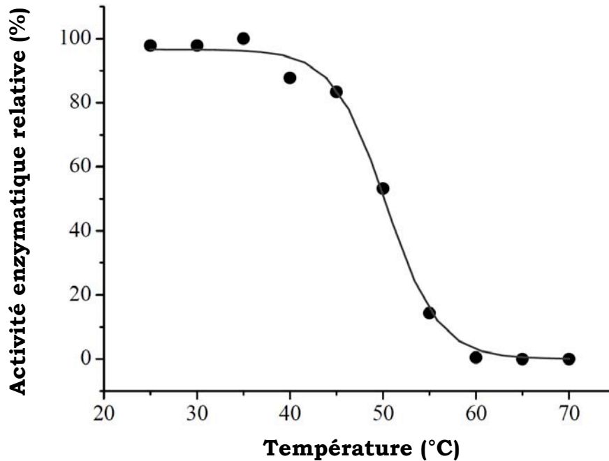
Figure 26: Stabilité thermique de la PPO du champignon de Paris ( Agaricus bisporus ) après 30 min de traitement thermique. Le milieu réactionnel contient 20 mM de pyrocatechol dans 0.1 M de tampon phosphate de sodium à pH 7.0.
