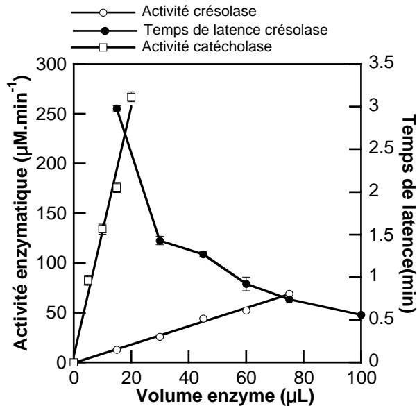
Figure 42. Effet du volume d'enzyme sur les vitesses initiale de la réaction de l'extrait brut de la PPO de truffe de désert ( Terfezia leonis Tul.). (○) Activité crésolase, (□) Activité catécholase, (●) Influence du pH sur la période de latence de l'activité crésolase.
