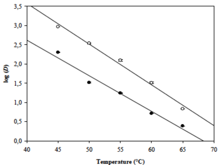
Figure 48: Variation du temps de réduction décimal avec la température pour la PPO de la truffe du désert (○) Activité crésolase, (●) Activité catécholase
