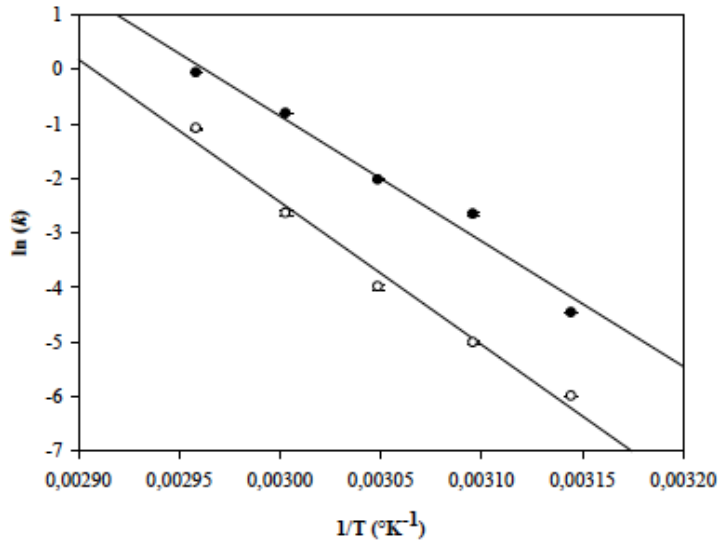
Figure 47: Graphique d'Arrhenius relatif à la vitesse d'inactivation thermique de la PPO de la truffe du désert (○) Activité crésolase, (●) Activité catécholase
